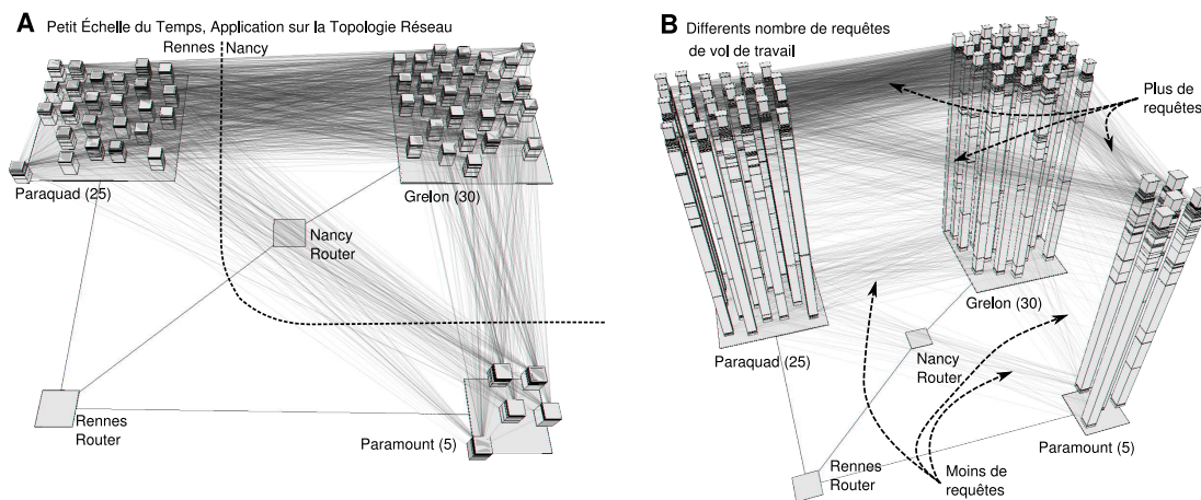
FIG. B.7 – Deux captures d’écran du prototype Triva pendant la visualisation d’une application composé de 60 processus, à différentes échelles de temps.
