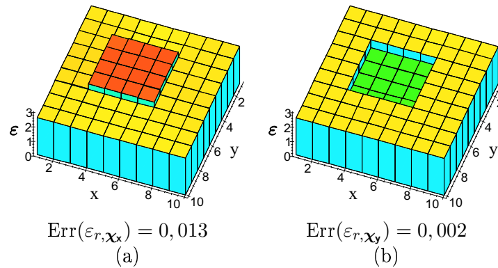
FIG. 8.43: Profil de permittivité anisotrope de \chi_x (a) et \chi_y (b) obtenu avec régularisation
