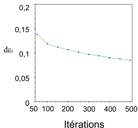
FIG. 8.38: Combinaison de polarisation avec champ d'antennes – Erreur normalisée en fonction des itérations
