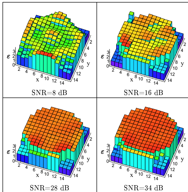
FIG. 8.11: Profils reconstruits en fonction du SNR. Simulations réalisées avec régularisation et pour la configuration I
