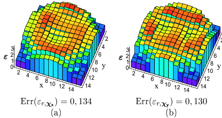
FIG. 8.26: Profils de permittivité de \chi_x (a) et \chi_y (b), reconstruits dans la bande [2–3] GHz avec 3 fréquences, sans régularisation et pour la configuration IV
