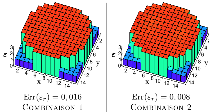
FIG. 8.35: Combinaison de polarisation pour un champ incident en ondes planes – Profils de permittivité
