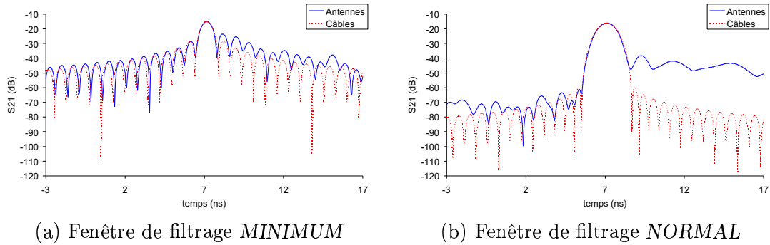
FIG. 2.41: Réponse impulsionnelle en transmission de l'antenne ETSA_A0 — bande [0,15–1,5] GHz
