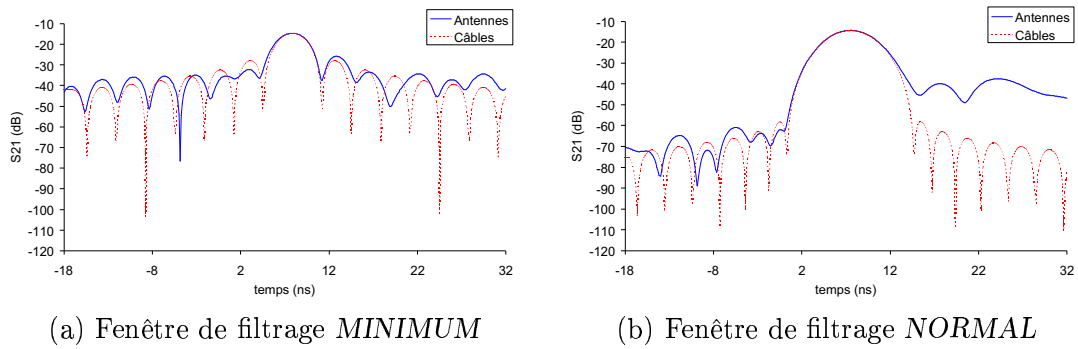
FIG. 2.42: Réponse impulsionnelle en transmission de l'antenne ETSA_A0 — bande [0,15–0,45] GHz
