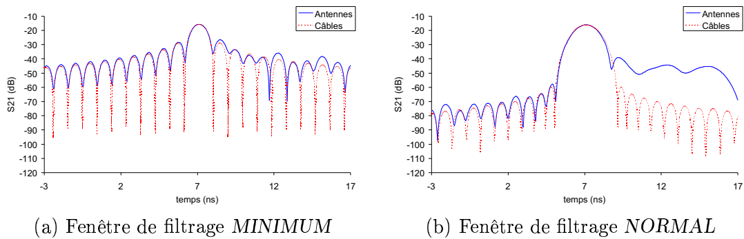
FIG. 2.43: Réponse impulsionnelle en transmission de l'antenne ETSA_A0 — bande [0,45–1,5] GHz
