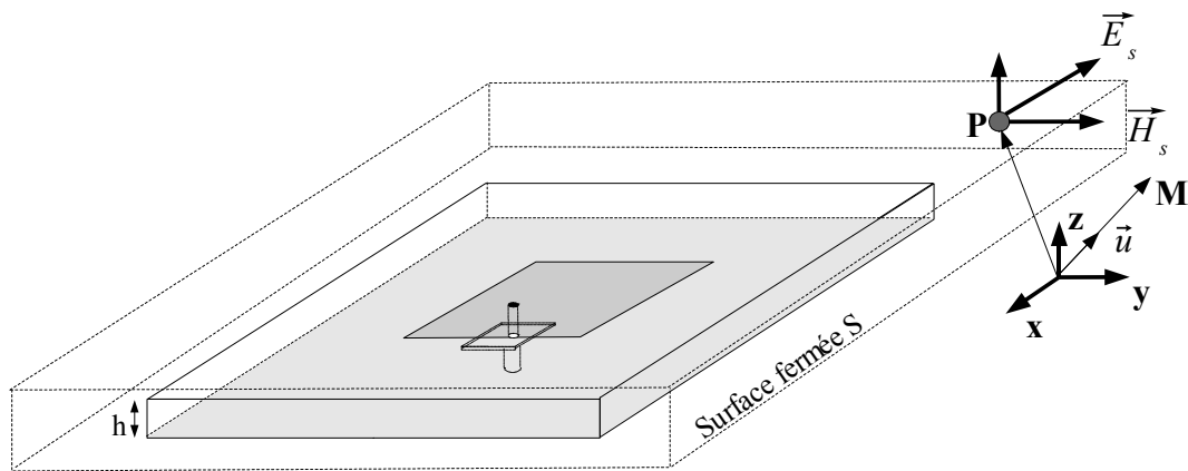
Figure 1.13 : Calcul du diagramme de rayonnement mettant en appliquant le principe d'équivalence
