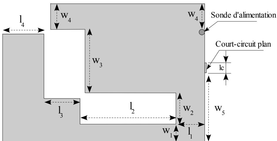
Figure 5.13 : Géométrie de l'antenne PIFA avec trois fentes arbitraires
