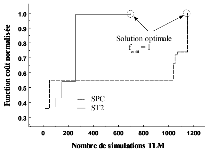
Figure 3.21 : Influence du type de sélection sur la convergence de l'AG
