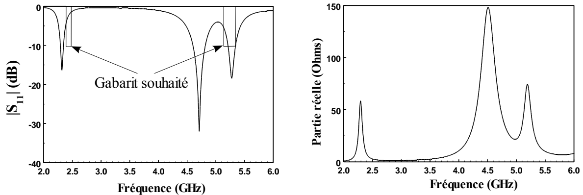
Figure 4.6 : |S_{11}|_{\text{dB}} et partie réelle de l'impédance d'entrée de l'antenne originale
