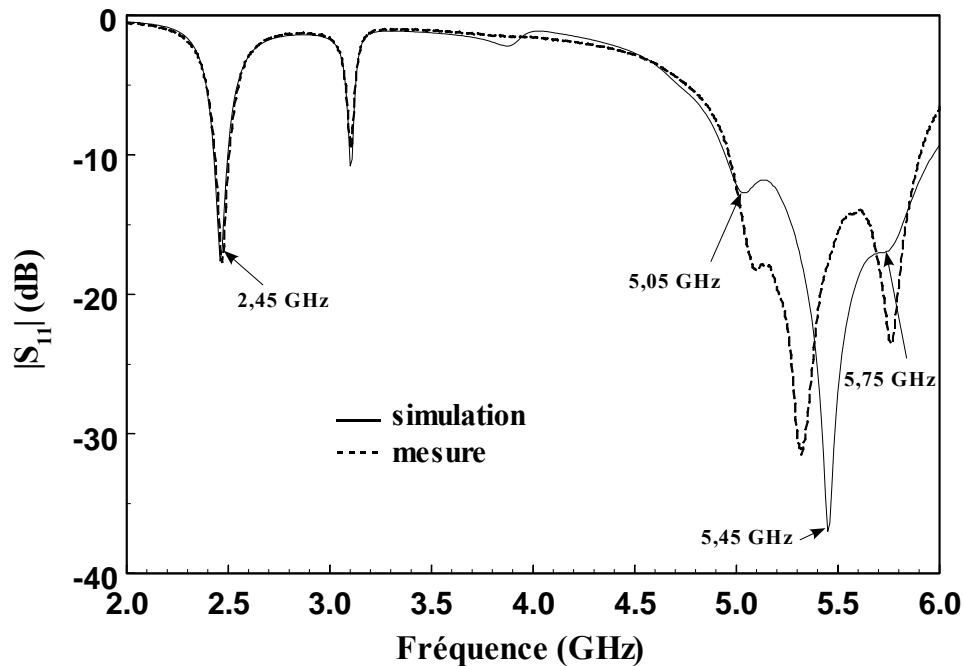
Figure 4.21 : |S_{11}|_{dB} de l'antenne carrée WLAN/HIPERLAN2 indoor et outdoor
