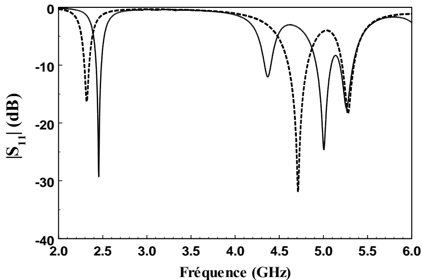
Figure 4.9 : Evolution du coefficient de réflexion — Antenne optimisée - - - - Antenne originale
