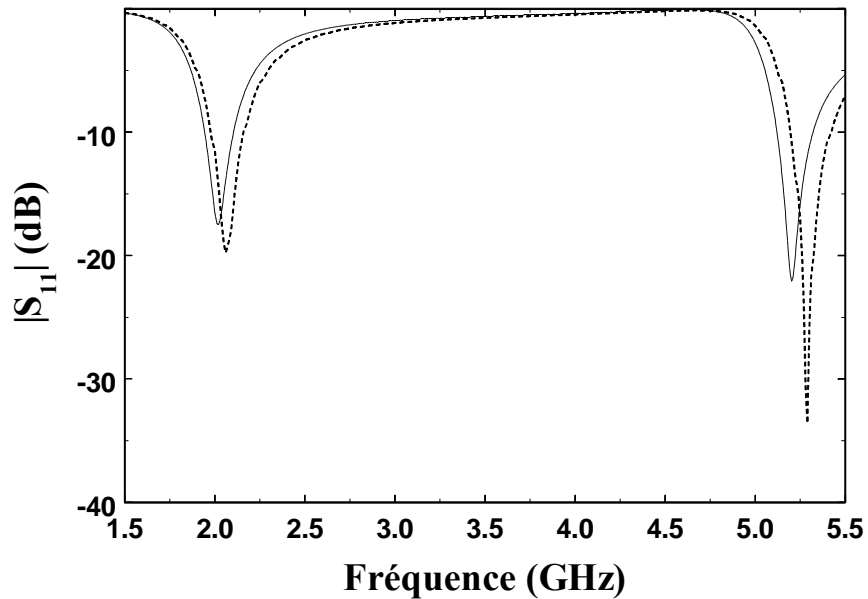
Figure 5.25 : |S_{11}|_{dB} de l'antenne fil-plaque UMTS/HIPERLAN2
