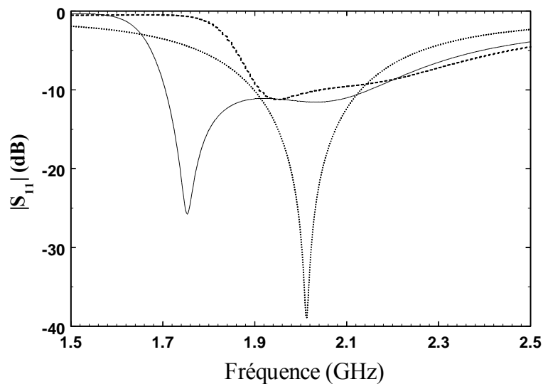
Figure 5.10 : Comparaison ( |S_{11}|_{dB} ) de l'antenne PIFA originale (...) et l'antenne optimisée simulé par TLM (—) et par IE3D (---)
