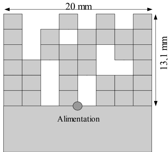
Figure 3.17 : Forme du pavé rayonnant vue de dessus
