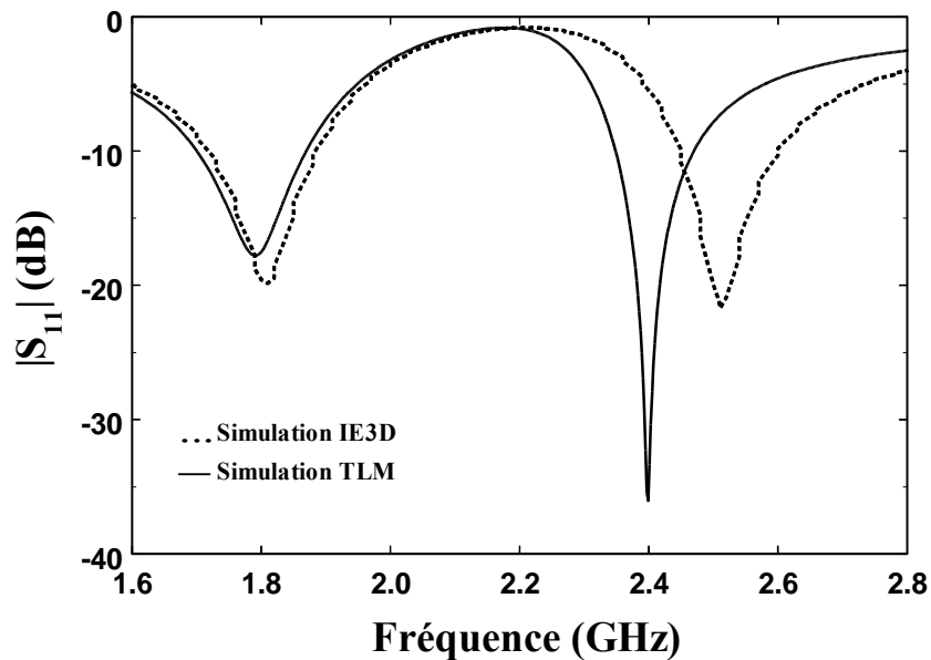
Figure 5.7 : |S_{11}|_{dB} de l'antenne PIFA-DCS/WLAN
