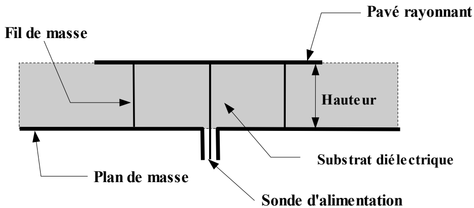
Figure 1.3 : Antenne fil-plaque monopolaire vue latérale
