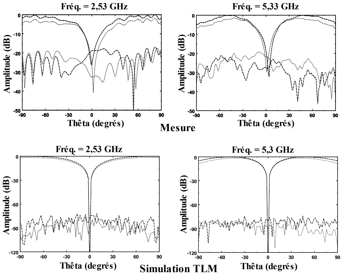
Figure D1 : Diagrammes de rayonnement de l'antenne fil-plaque monopolaire WLAN/HIPERLAN2 mesurés et simulés par TLM sur un plan de masse 50 x 50 mm 2
