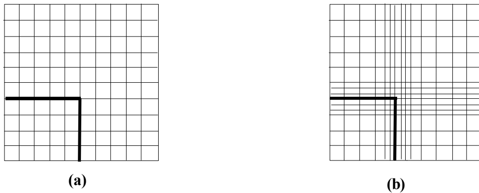
Figure 1.8 : Différentes formes de maillage a) Maillage uniforme b) Maillage variable
