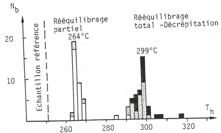
Figure 29. Histogramme de T_h obtenu après expérimentation (PECHER, 1981) Echantillon 1C ( n_p = 200 MPa, T = 500^\circ\text{C} ), classes de 2^\circ\text{C} ; en blanc : grandes inclusions secondaires isolées correspondant à des inclusions partiellement rééquilibrées en pointillé : grandes inclusions secondaires entourées de petites inclusions fluides* en noir : petites inclusions secondaires* *Ces deux catégories correspondent à des inclusions fluides décrépitées et des néo-inclusions formées autour d'elles, par colmatage des microfractures apparues.
