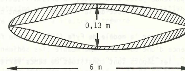
Figure 3. Calcul de la masse de remplissage minéral d'une fente assimilée à une ellipse.
