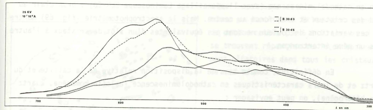
Figure 69. Spectres obtenus après passage au spectrophotomètre du CENG. Cristaux de quartz - section B30d3.
