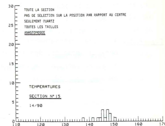
Figure 44. A droite, histogrammes de T_h obtenus après tri des inclusions en fonction de leur forme - section n°15. A gauche, on a reporté l'histogramme brut de la fig. 43.
