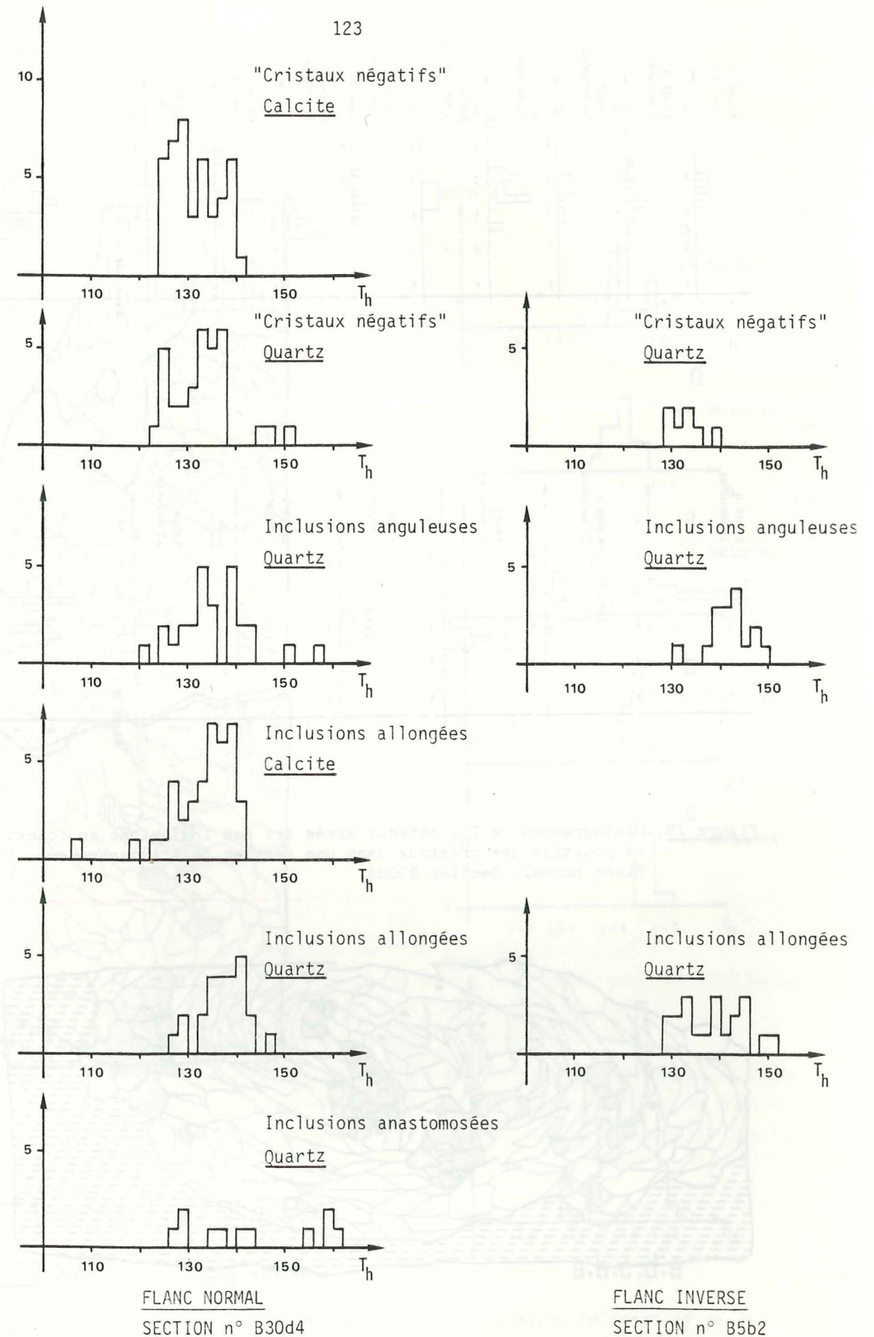
Figure 77. Histogrammes des T_h en fonction de la forme des inclusions fluides.
