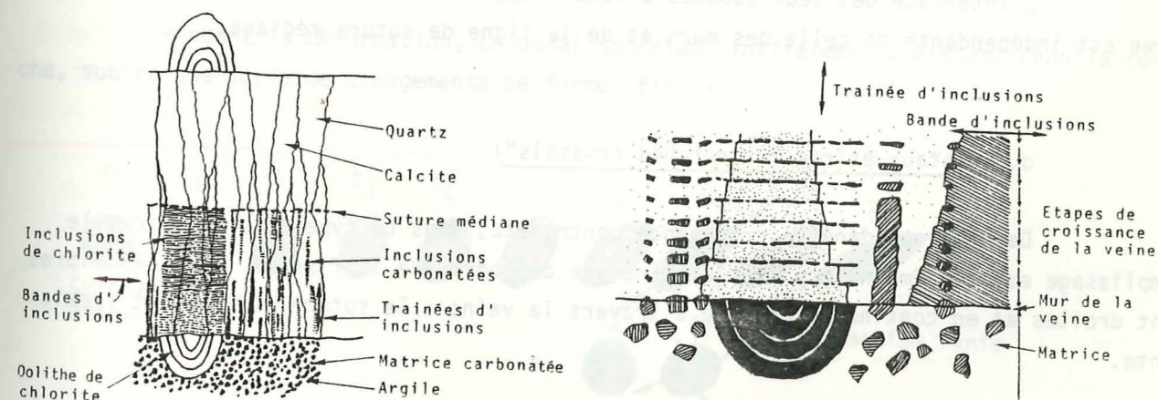
Figure 8. Diagrammes schématiques montrant le remplissage quartzo-calcaïque d'une veine tectonique provenant du massif de l'Aar (Suisse Centrale), d'après Ramsay (1980).
