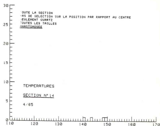
Figure 46. A droite, histogrammes de T_h obtenus après tri des inclusions en fonction de leur forme - section n°14. A gauche, on a reporté l'histogramme brut de la fig. 45.
