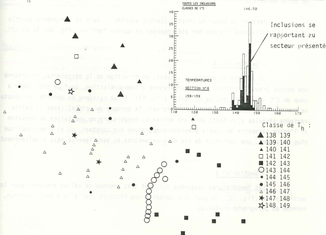
Figure 49. Inclusions particulières à la section n°6. en haut : forme et disposition des inclusions en bas : T_h mesurées.
