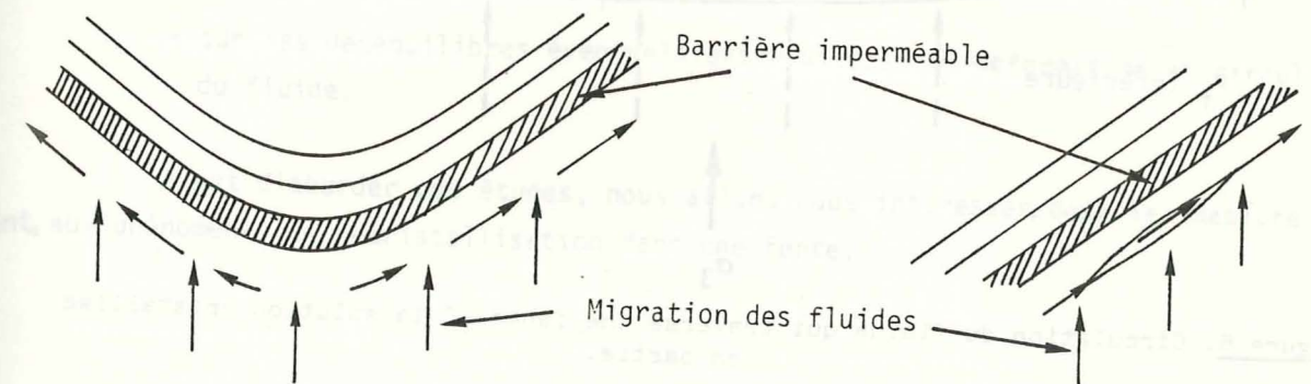
Figure 5. Circulation du fluide lorsqu'il rencontre une barrière imperméable, conséquence sur la cristallisation (Fyfe et al., 1978).
