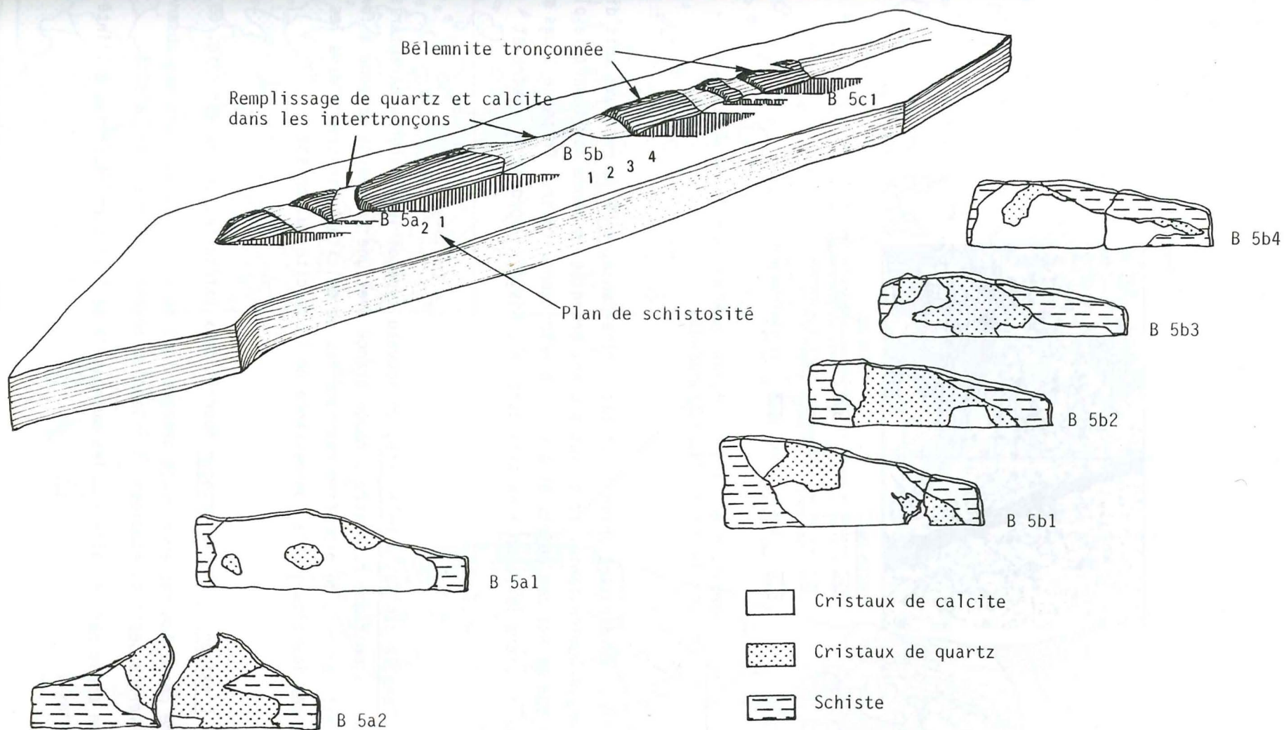
Figure 65. Coupes effectuées perpendiculairement au plan de schistosité. Sections obtenues. Echantillon B5. Flanc inverse.
