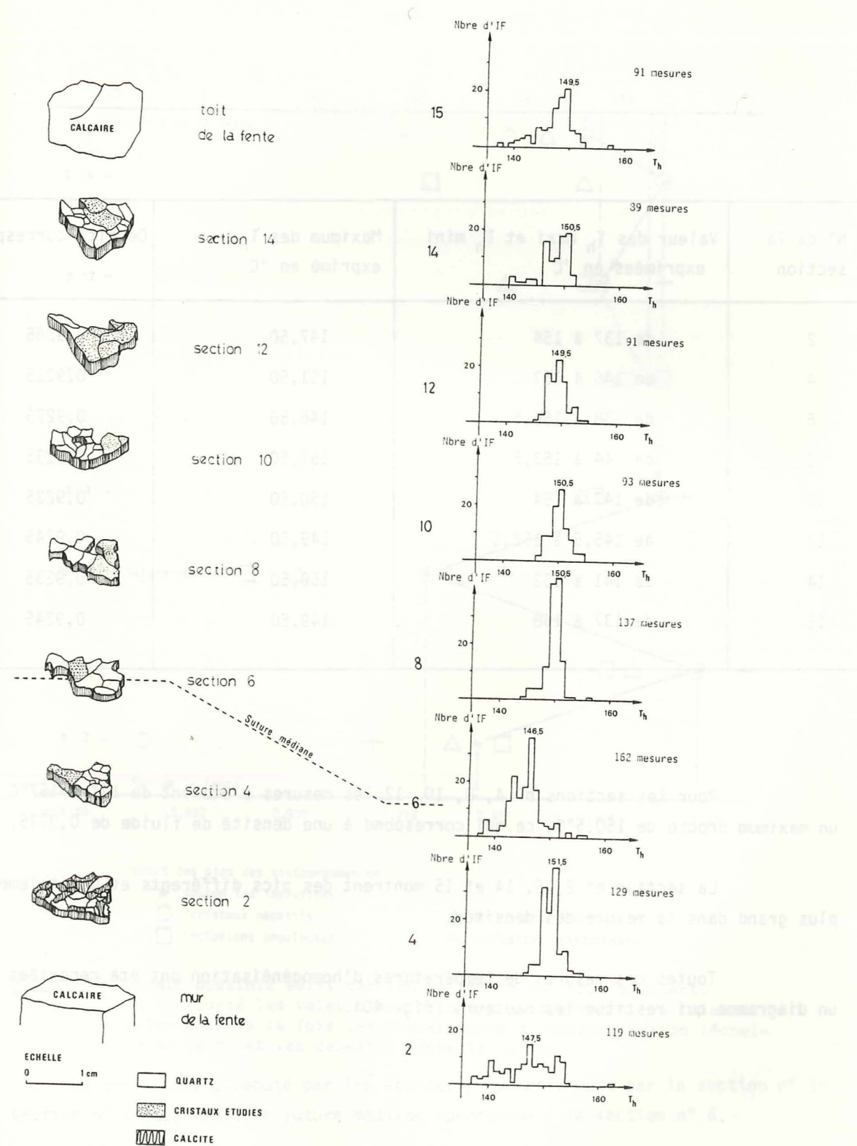
Figure 39. Histogrammes des températures d'homogénéisation en fonction de la position des cristaux étudiés dans la fente.
