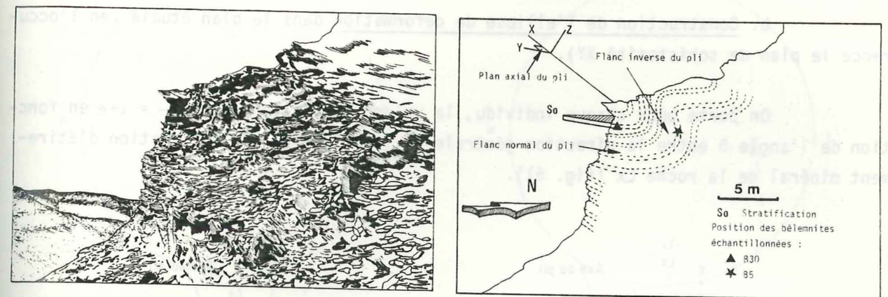
Figure 59. Schéma du pli échantillonné.
