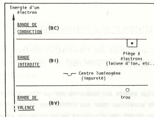
Figure 11. Modèle des "bandes d'énergie" pour les cristaux non conducteurs (Barde, 1979).
