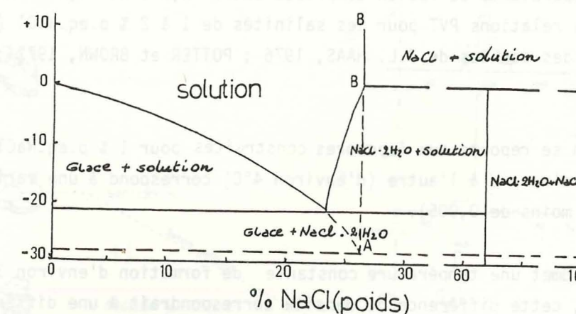
Figure 38. Le système \text{H}_2\text{O} - \text{NaCl} (Int. Crist. Tables IV p. 235, 1928, d'après ROEDDER, 1962, p. 1059).
