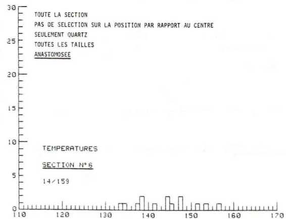
Figure 48. A droite, histogrammes de T_h obtenus après tri des inclusions en fonction de leur forme - section n°6. A gauche, on a reporté l'histogramme brut de la fig. 47.
