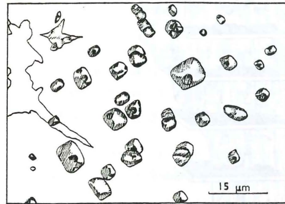
Figure 33. Inclusions fluides en forme de "cristaux négatifs" (section n°8, température ambiante).
