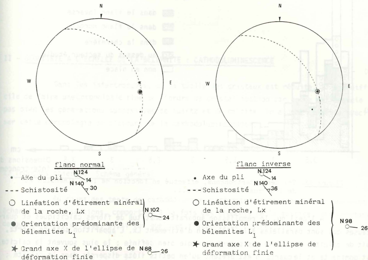
Figure 62. Report des mesures obtenues en hémisphère inférieur.
