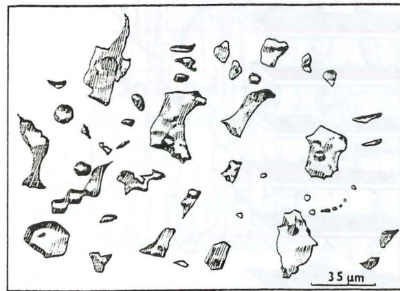
Figure 34. Inclusions fluides anguleuses (section n°8, température ambiante).
