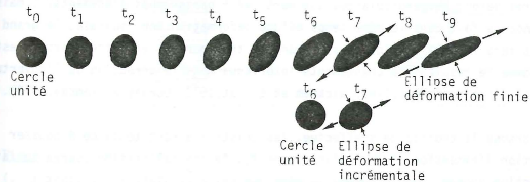
Figure 9. Une séquence de déformation progressive en deux dimensions. La forme de l'ellipsoïde de déformation à différentes étapes indique la déformation totale à des périodes successives au cours de la déformation (Durney et Ramsay, 1973).
