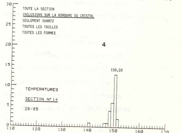
Figure 50. A droite, histogrammes de T_h obtenus après tri des inclusions en fonction de leur position dans le cristal : 1. au centre 2. proches du centre 3. proches de la bordure 4. en bordure du cristal. A gauche, on a reporté l'histogramme brut de la fig. 45.
