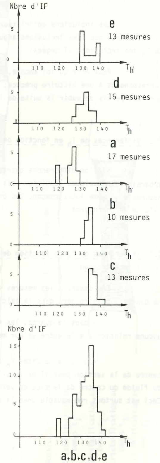
Figure 79. Histogrammes de T_h , obtenus après tri des inclusions en fonction de la position des cristaux dans une section de l'intertronçon. Flanc inverse. Section B5a1.
