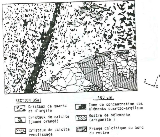
Figure 66. Observation en cathodoluminescence de la matrice schisteuse proche du rostre de la bélemnite.
