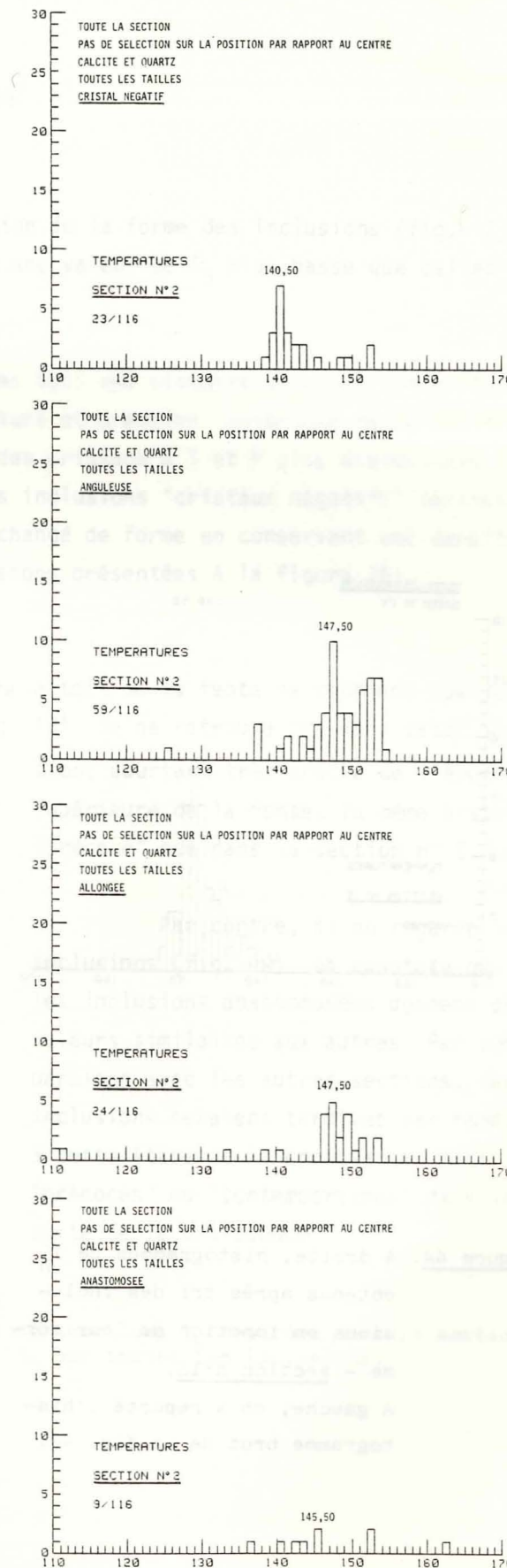
Figure 42. A droite, histogrammes de T_h obtenus après tri des inclusions en fonction de leur forme -section n°2. A gauche, on a reporté l'histogramme brut de la fig. 41.
