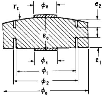
FIGURE 4.12: Géométrie du résonateur rainuré fabriqué.
