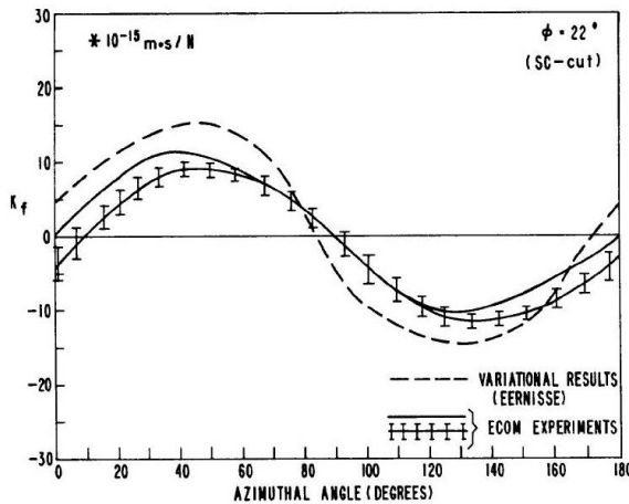
FIGURE 4.21: Coefficient force-fréquence K_f(\psi) pour le résonateur standard [72].
