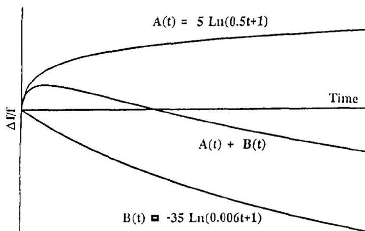
FIGURE 3.1: Allure des différents vieillissements [21].
