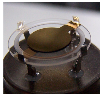
FIGURE 3.23: Montage d'un résonateur en 4 points.
