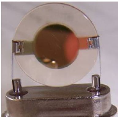
FIGURE 3.21: Montage d'un résonateur en 2 points.
