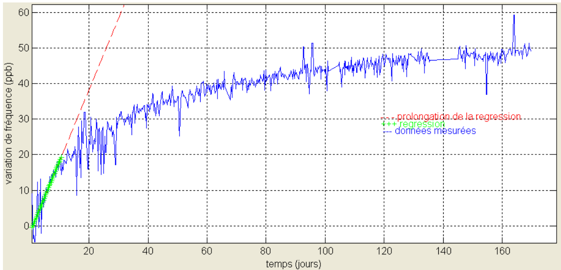
FIGURE 5.22: Régression linéaire du vieillissement d'un oscillateur à quartz sur 10 jours.
