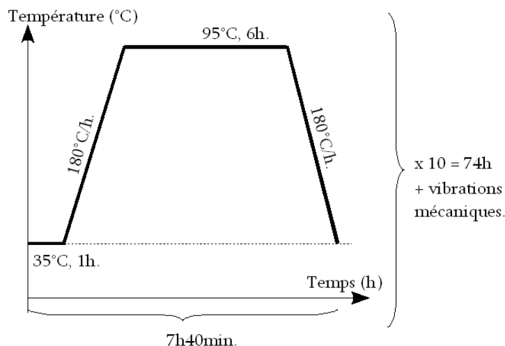
FIGURE 5.24: Illustration du cycle optimal obtenu avec le plan d'expérience.
