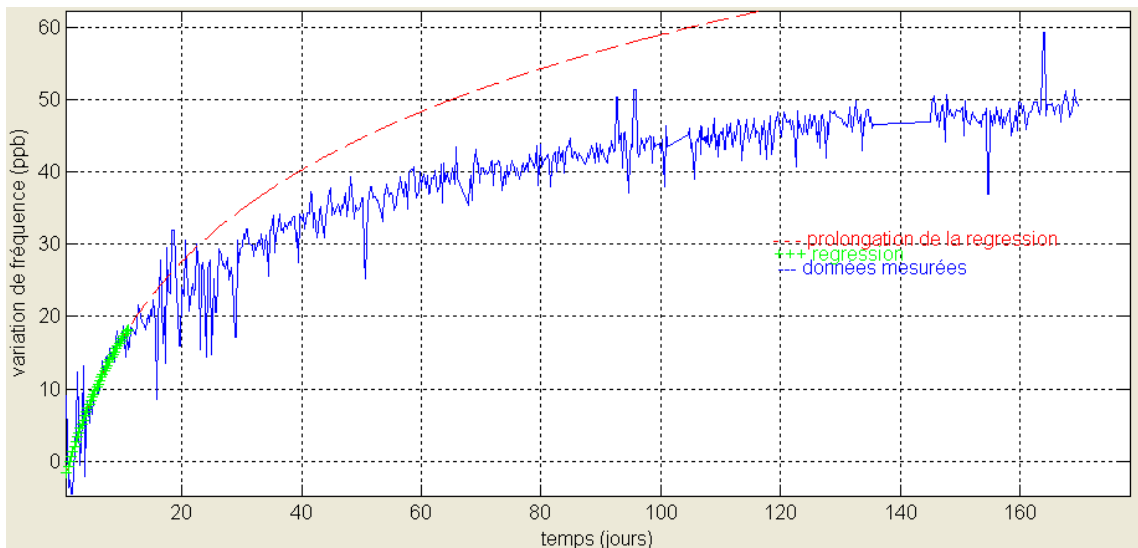
FIGURE 5.23: Régression logarithmique du vieillissement d'un oscillateur à quartz sur 10 jours.
