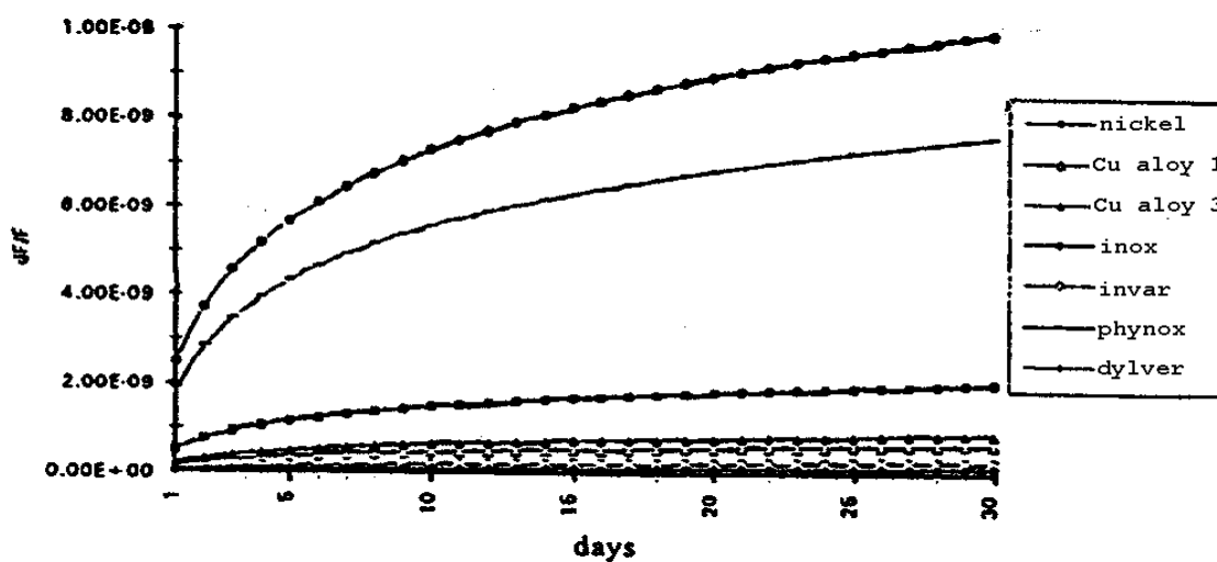
FIGURE 3.28: Variation de fréquence calculée à 75°C pour divers matériaux. [43].
