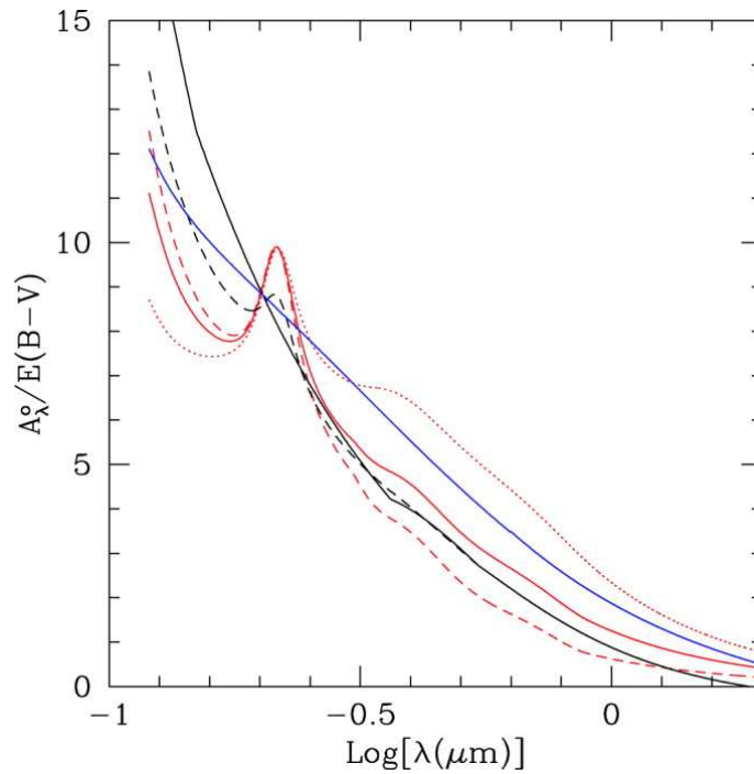
FIG. 6.2 – Courbe d’extinction dans plusieurs environnements (figure extraite de Calzetti 2001). La courbe de la Voie Lactée est montrée pour R_V valant 3.1 (trait rouge plein), 5.0 (trait en tirets rouges) et 2.0 (trait en pointillés rouges). Les deux autres courbes sont celles de la région H II géante 30 Dorade dans le Grand Nuage de Magellan (trait en tirets noirs), et de la barre du Petit Nuage de Magellan (trait plein noir). La courbe bleue est ici à titre de comparaison et représente la courbe d’obscurcissement dans les galaxies à flambée de formation d’étoiles. Le domaine de FUSE se trouve entre \log \lambda(\mu m) \approx -1.05 et -1 , à l’extrême gauche du graphique, où l’extinction est la plus importante.
