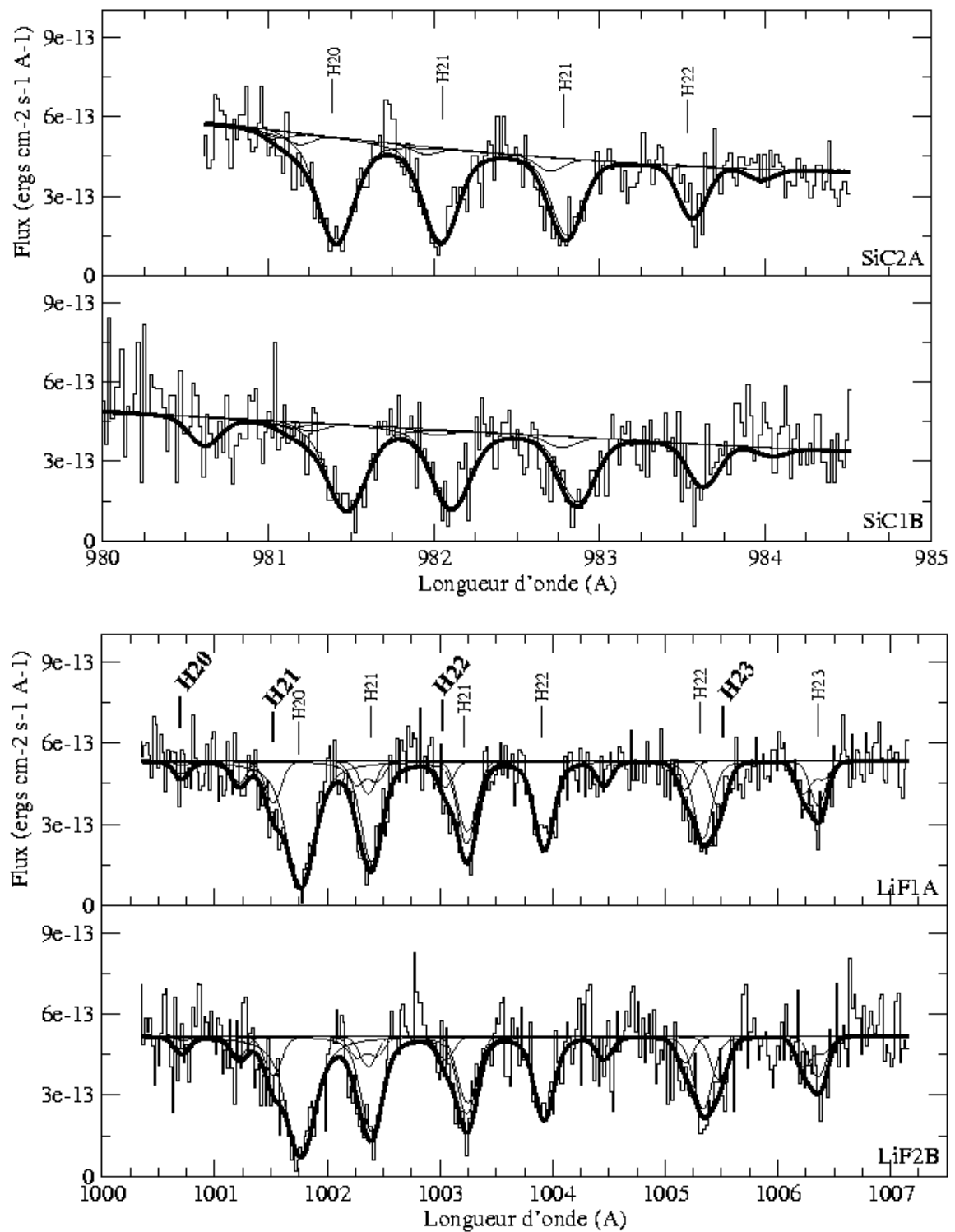
FIG. B.4 – \sim 980-985 \text{ \AA} - Raies d'hydrogène moléculaire de notre Galaxie. \sim 1000-1007 \text{ \AA} - Indices de présence de raies moléculaires dans NGC604 qui sont mélangées avec d'autres raies de la Voie Lactée.
