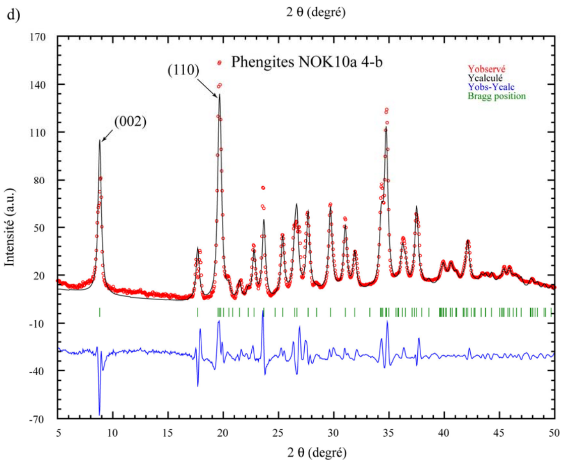
Figure VI-2 : Spectres de diffraction des rayons X obtenus pour quatre fractions de phengites de l'échantillon NOK10a (a) fraction 2+a, (b) fraction 2+b, (c) fraction 2-a et (d) fraction 4-b. L'intensité du signal en unité arbitraire (a.u.) est reportée en fonction de l'angle 2\theta exprimé en degré. Sur chaque figure, le spectre observé ( Y_{\text{observé}} ), calculé après affinement des paramètres de maille ( Y_{\text{calculé}} ), la différence entre le spectre observé et calculé ( Y_{\text{obs}}-Y_{\text{calc}} ), et la position des plans de réflexion (Bragg position) sont représentés.
