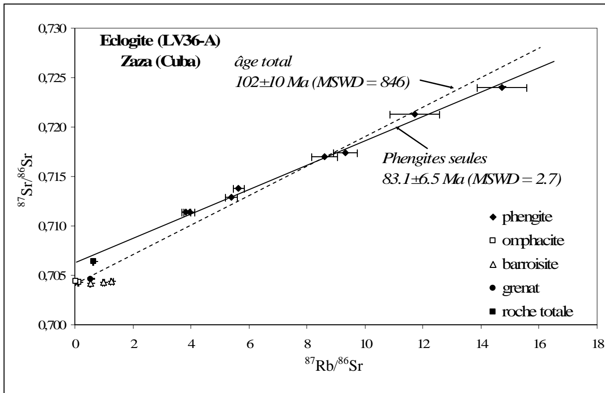
Figure VII-3 : Diagramme isochrone Rb/Sr où sont reportées les analyses de huit fractions de phengite, trois fractions de barroisite, deux fractions d'omphacite, une fraction de grenat et la roche totale d'une éclogite (LV36-A) de la zone de Zaza (Cuba). (Schneider et al., données non publiées).
