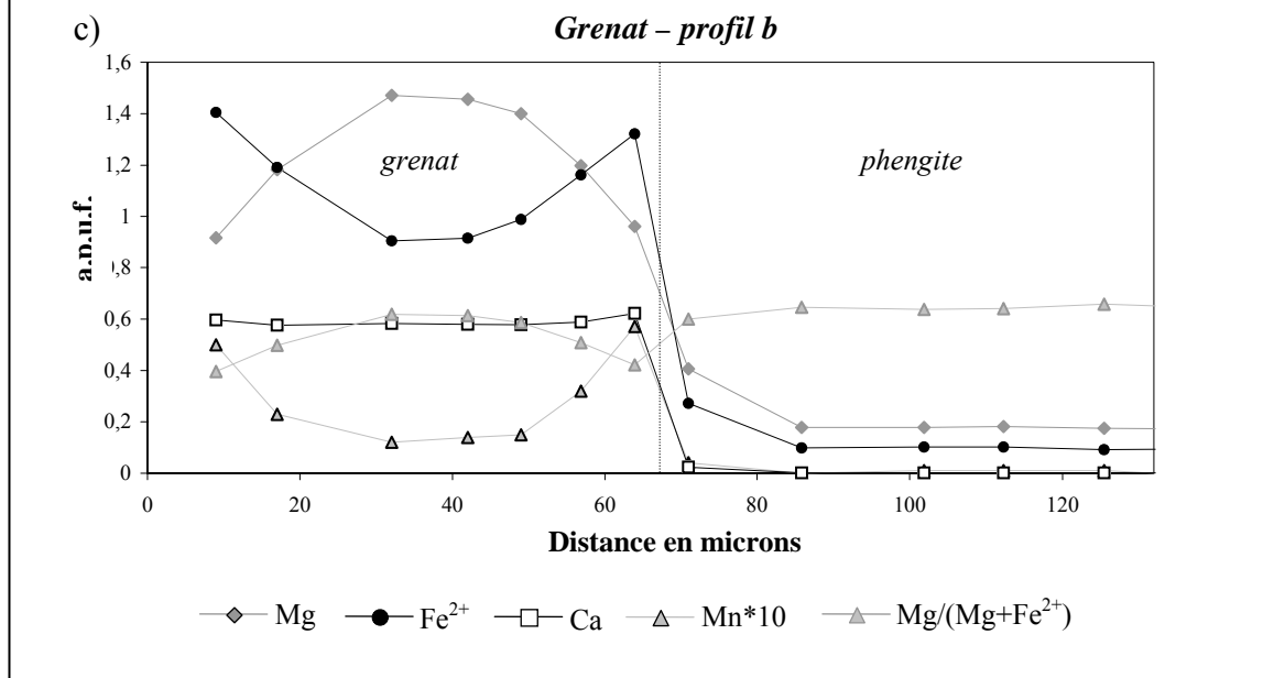
Figure III-7 : profils réalisés à la sonde électronique dans différents minéraux de l'échantillon NOK10a (a) profil réalisé dans une épidote. Ce minéral ne présente pas de zonation remarquable. (b) profil réalisé dans le grenat des figures III-6a, b et c. L'orientation du profil a est montrée sur la figure III-6c. Ce profil montre clairement la distinction entre le grenat granulitique au cœur (grenat I) et le grenat éclogitique en bordure (grenat II). (c) profil réalisé entre un grenat et une phengite vus dans les figures III-6a, b et c. L'orientation du profil b est montrée sur la figure III-6c. La limite entre les deux minéraux est définie par une ligne sur la figure.
