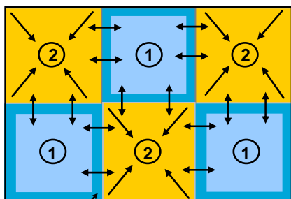
Bordure du minéral 1 participant à la diffusion intergranulaire (1-3 nm)
