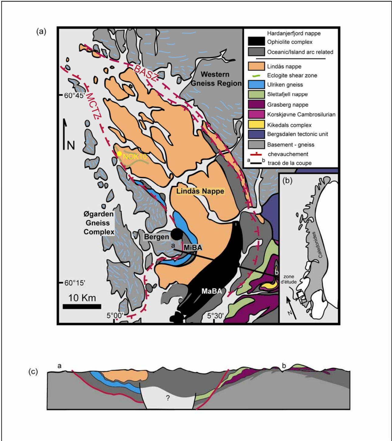
Figure II-5 : (a) Carte géologique de l'arc de Bergen d'après Boundy et al. (1996) et Kühn et al. (2000), montrant la localisation des échantillons sur l'île d'Holsnøy. (b) Localisation de la zone d'étude par rapport aux Calédonides de Norvège. (c) Coupe schématique à travers l'arc de Bergen (a-b) dans Bingen et al. (2001). (MCTZ) Zone majeure de chevauchement Calédonien; (BASZ) zone de cisaillement de l'arc de Bergen; (MaBA) Arc de Bergen majeur; (MiBA) Arc de Bergen mineur.
