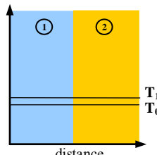
T_1 > T_{f1} Diffusion intergranulaire et volumique efficace. L'équilibre isotopique est préservé.
