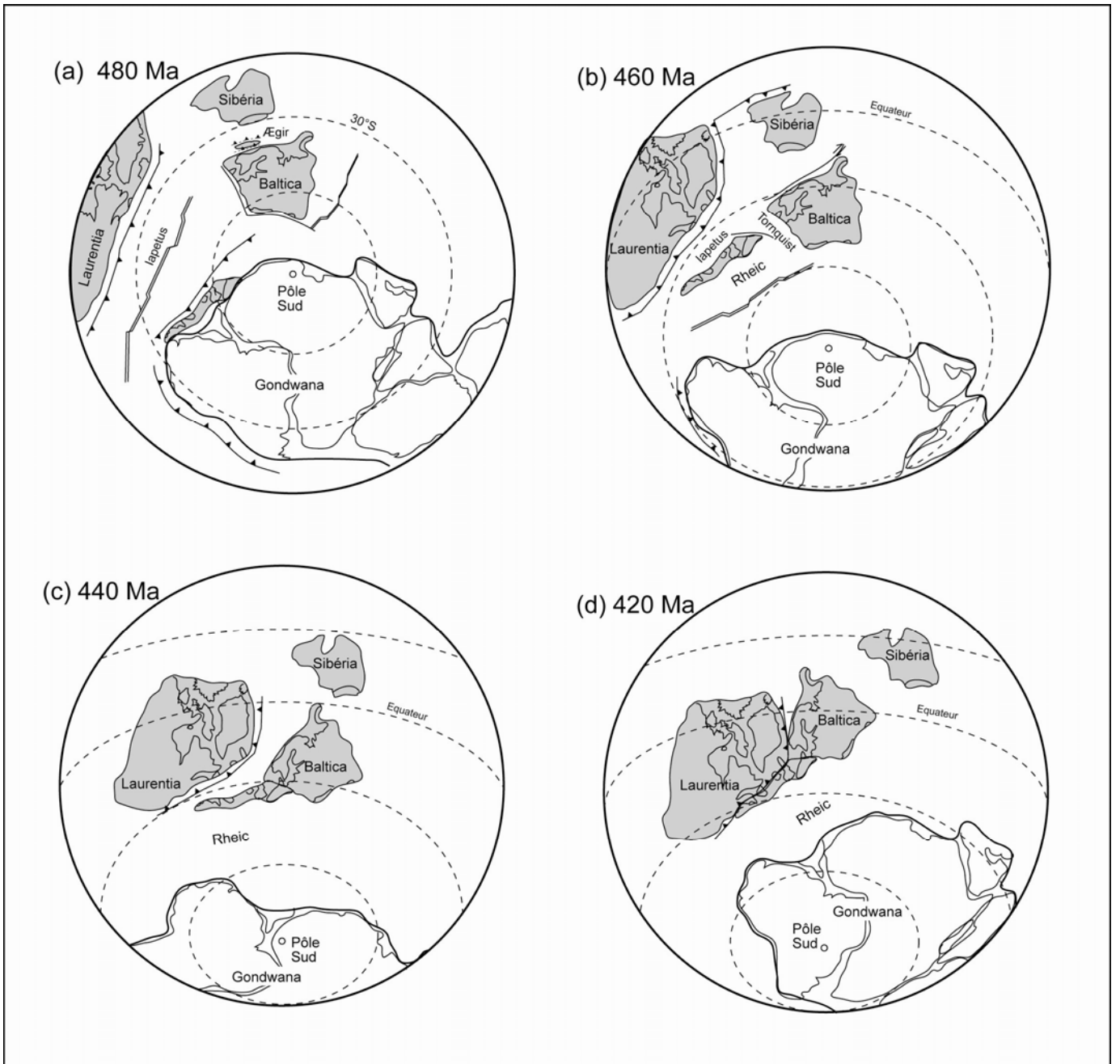
Figure II-3 : Reconstitution paléomagnétique simplifiée de l'Ordovicien inférieur au Silurien supérieur, avec mise en valeur du changement graduel et de l'interaction entre les plaques Baltica, Sibéria et Laurentia (D'après Roberts, 2003).
