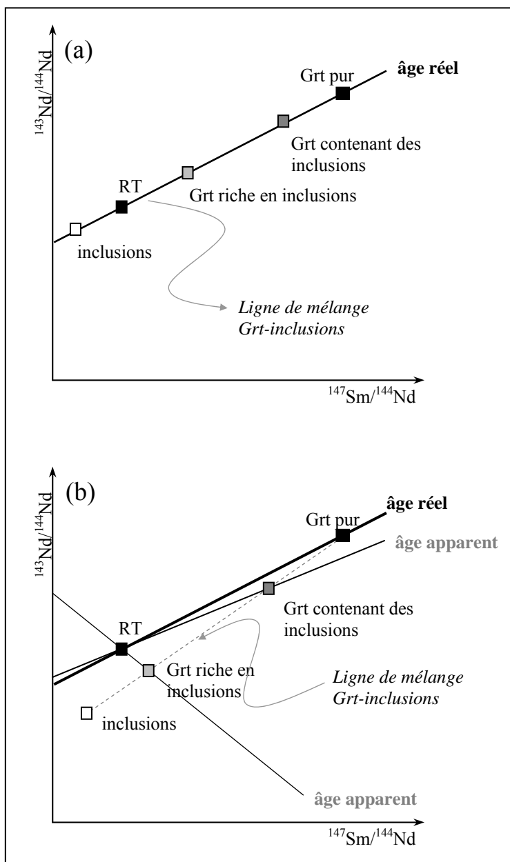
Figure I-17: Diagrammes isochrones Sm/Nd schématiques montrant l'effet de la présence d'inclusions sur la composition isotopique des grenats (Grt). (a) Cas où les inclusions et les grenats sont cogénétiques, dans ce cas l'âge isochrone obtenu correspond bien à l'âge de cette paragenèse. (b) Cas où les inclusions sont héritées d'un protolithe ancien et où elles ne se sont pas rééquilibrées isotopiquement avec les grenats. Dans ce cas l'âge isochrone RT (roche totale)-Grt (avec des inclusions) est un âge apparent qui n'a pas de signification géologique, cet âge peut être négatif dans certains cas.
