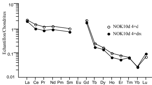
Figure A-7 : Comparaisons entre des données obtenues à l'ICP-MS de l'ISTEEM (Université Montpellier II) à un an d'intervalle sur des mêmes fractions de phengites. Pour les terres rares légères et moyennes, les données sont très reproductibles. La reproductibilité sur les terres rares lourdes est de moins bonne qualité, ce qui peut être expliqué par le fait qu'elles sont présentes en très faible concentration dans les phengites analysées, par conséquent l'erreur sur la mesure est plus importante. Globalement les différences au niveau des terres rares sont attribuées surtout à l'inhomogénéité des poudres (par exemple la différence importante en Tm pour l'échantillon NOK10d 4+c). Par contre on note des différences importantes au niveau des concentrations en Ta et U. Les données en Ta et U ne sont donc pas prises en considération dans la discussion des résultats.
