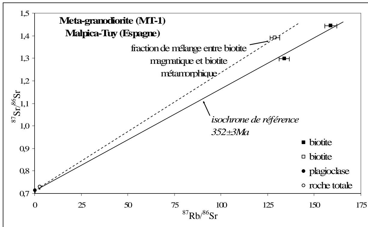
Figure VII-5 : Diagramme isochrone Rb/Sr pour la roche totale et des minéraux d'une méta-granodiorite (MT-1) de Malpica-Tuy (Espagne, dans Santos Zaldegui et al., 1995).
