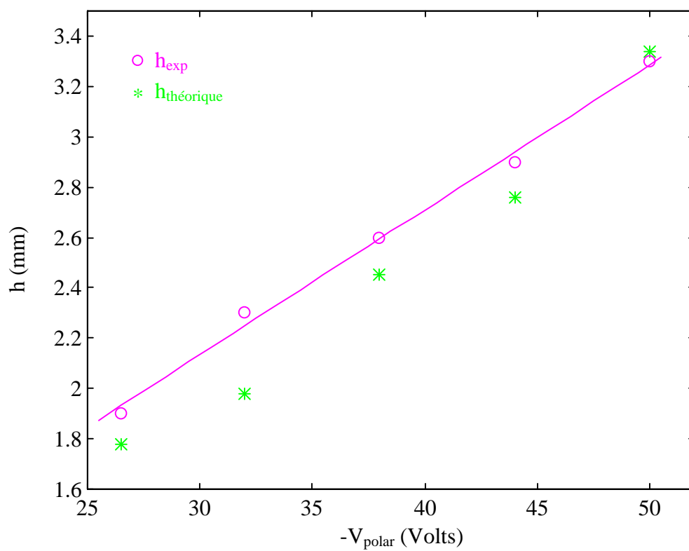
Figure III.8 : Hauteurs de lévitation expérimentales et théoriques en fonction de V_{polar}
