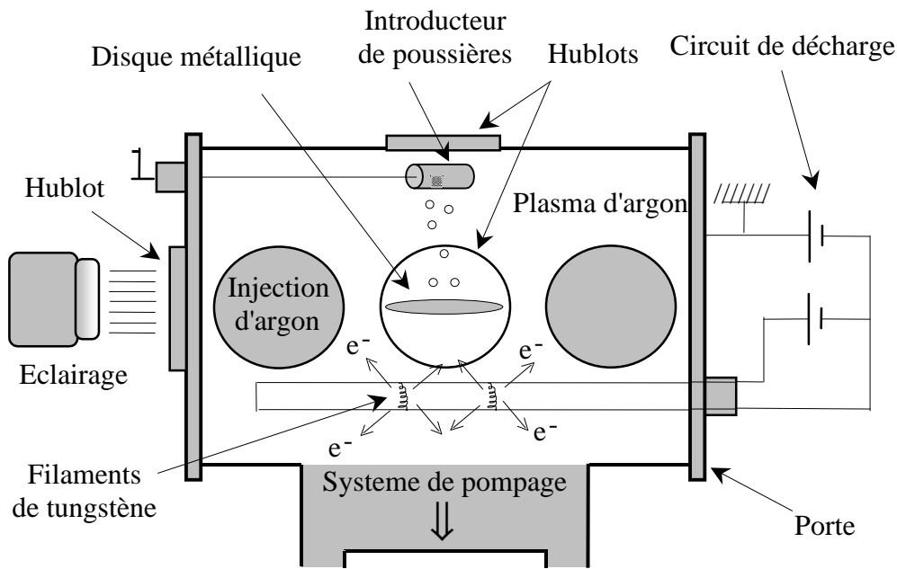
Figure II.1 : Dispositif expérimental
