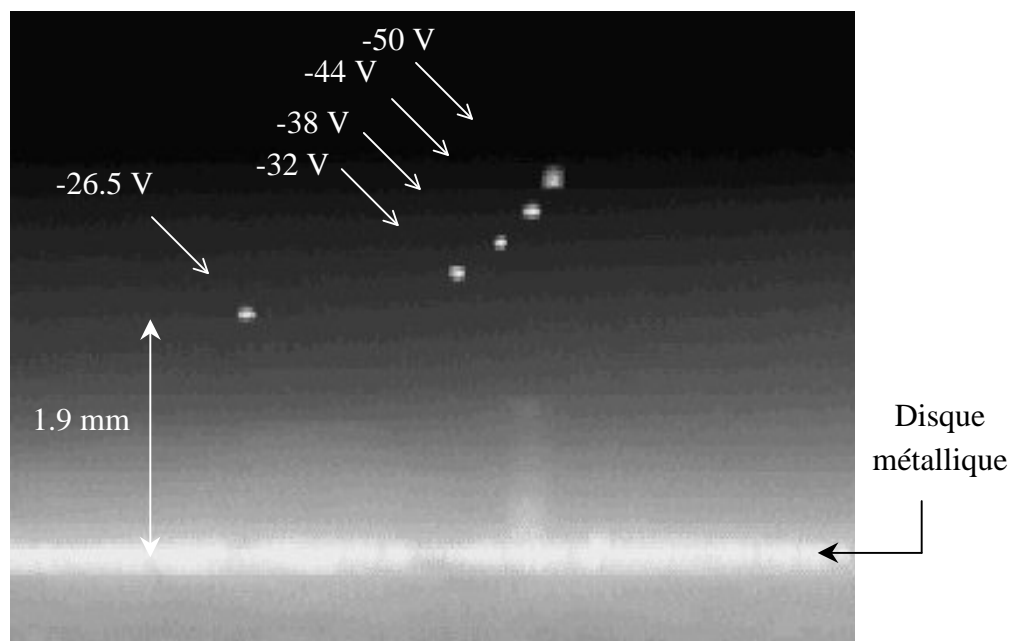
Figure III.7 : Hauteur de lévitation en fonction de V_{polar}
