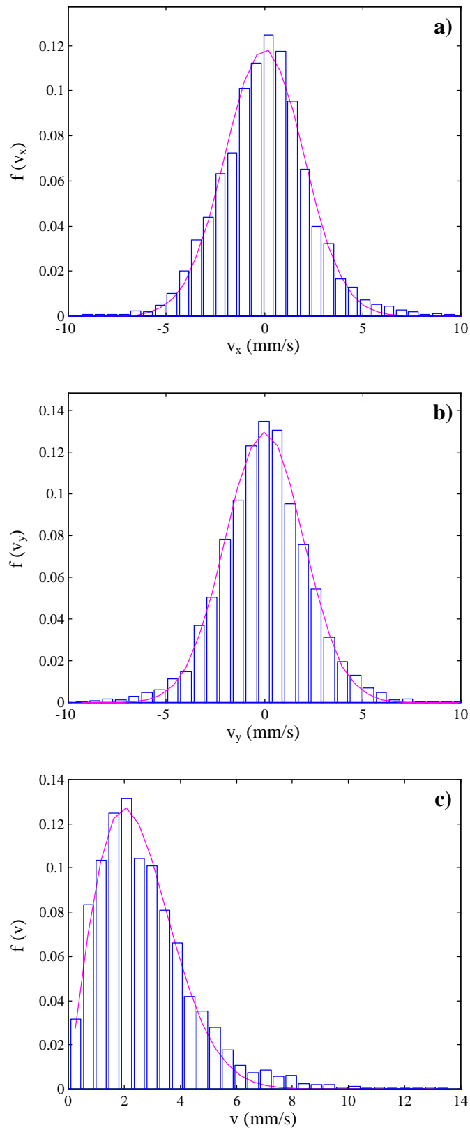
Figure V.15 : Fonction de distribution de a) v_x , b) v_y , c) v
