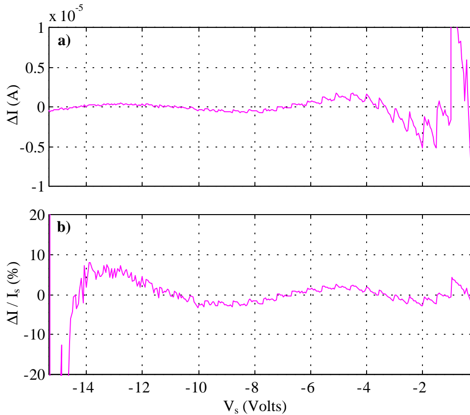
Figure II.11 : a) Erreur \Delta I = I_s - I_{fit} b) Erreur relative \Delta I / I_s
