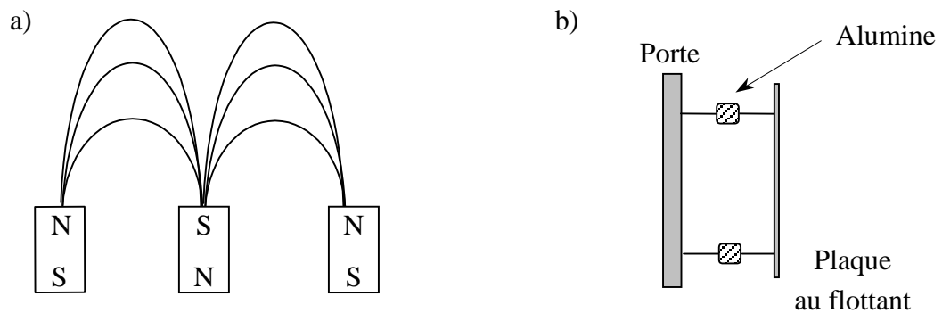
Figure II.5 : Méthodes de confinement a) magnétique b) électrostatique
