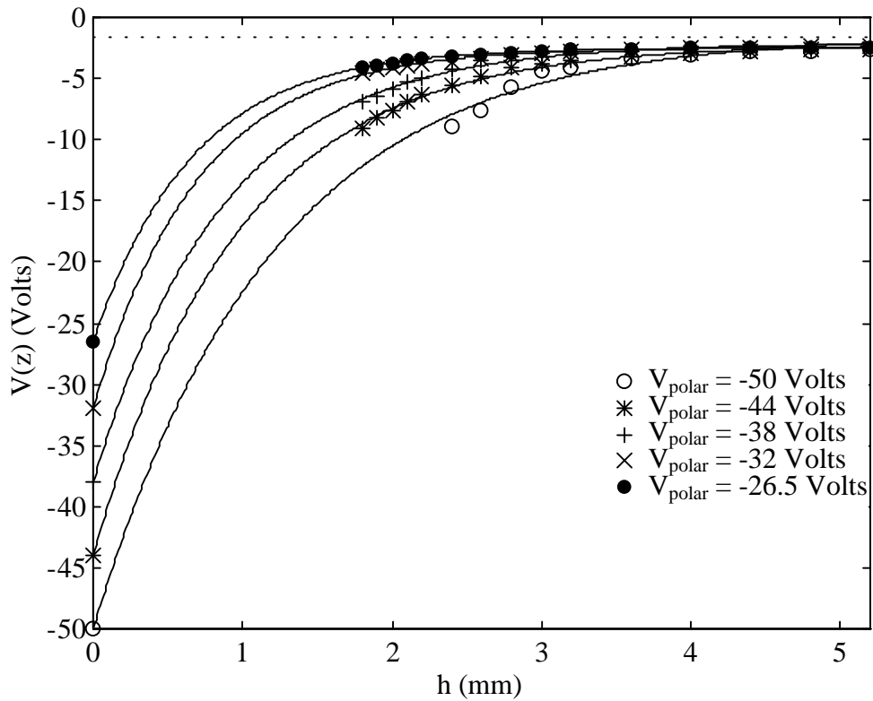
Figure III.4 : Profils de potentiel pour différentes valeurs de V_{polar}
