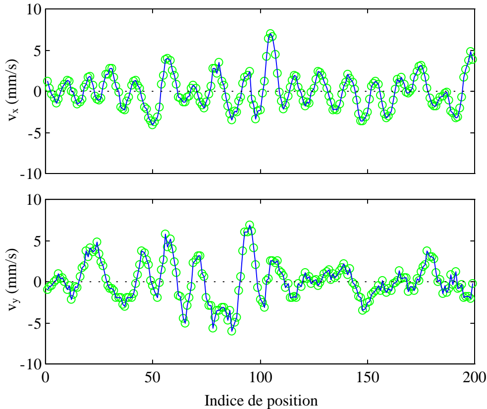
Figure V.17 : Evolution temporelle de v_x et v_y (valeurs moyennes en pointillés)
