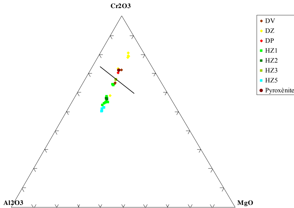
Figure 1.14: Diagramme triangulaire Cr 2 O 3 -Al 2 O 3 -MgO présentant l'évolution de la composition des chromites en fonction des faciès des séquences ultramafiques du massif du Koniambo. Les teneurs en Cr 2 O 3 des chromites des harzburgites de la SHS sont nettement inférieures à celles des chromites observées dans les péridotites de la séquence de Vavouto.
