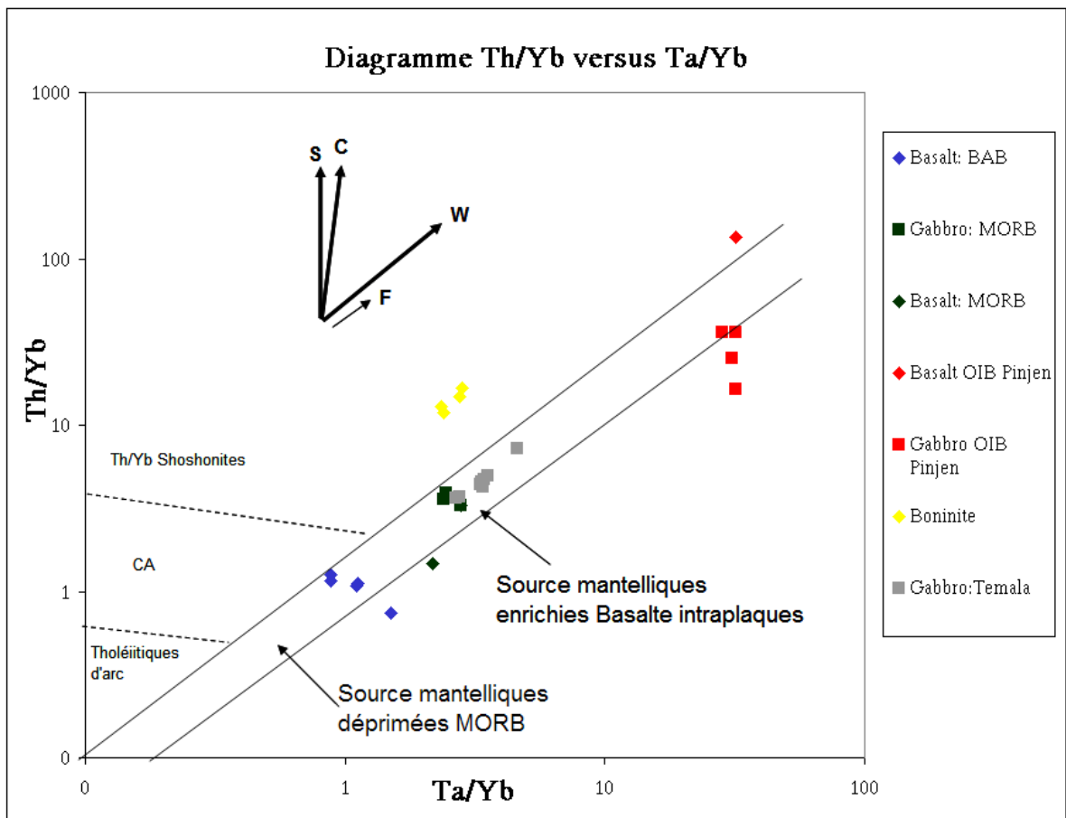
Figure 1.6: Diagramme discriminant Th/Yb versus Ta/Yb (Pearce, 1983) pour les volcanites et gabbros de l'Unité de Poya de la baie de Vavouta. Puisque les éléments Th, Ta et Yb sont incompatibles, les ratios Th/Yb et Ta/Yb minimisent les effets du fractionnement magmatique et permettent de déterminer les caractéristiques originales des sources. Les unités tholéitiques (BAB et MORB) présentent des ratios faibles tandis que les OIB de Pinjen présentent une distribution qui suggère une source mantellique enrichie, typique des basaltes intraplaques. Les gabbros de Témala présentent une affinité géochimique de type MORB. Les vecteurs indiquent les variations chimiques induites par la cristallisation fractionnée (F), les effets de la source (W), la contamination crustale (C), et par la subduction (S).
