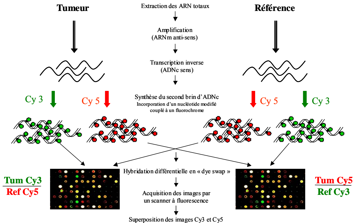
Figure 18 Principe de l'hybridation sur puces à ADN
