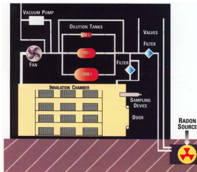
Figure 16 Schéma simplifié des chambres d'inhalation de radon et de ses descendants
