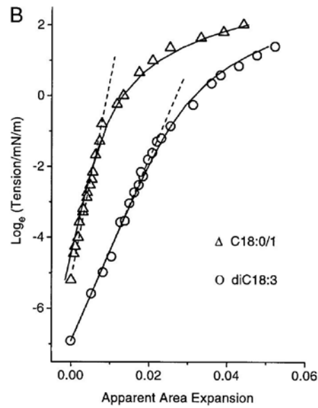
FIG. 2.19: \ln\sigma en fonction de \alpha correspondant à l'aspiration d'une vésicule de SOPC (C 18 :0/1) et de dilinoleoyl-sn-phosphatidilcholine (diC 18 :3), extrait de [Rawicz et al., 2000]. On obtient pour le (C 18 :0/1) k_C = 0,90 \cdot 10^{-19} J ( 22,5 k_B T ) et pour le (diC 18 :3) k_C = 0,56 \cdot 10^{-19} J ( 14 k_B T )
