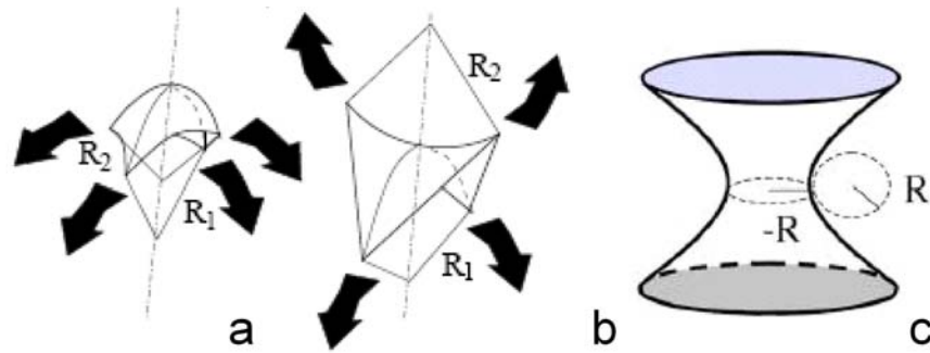
FIG. 2.5: Exemples de surfaces courbes : (a) avec une courbure gaussienne c_1c_2 = 1/R_1R_2 > 0 , (b) avec une courbure gaussienne c_1c_2 = 1/R_1R_2 < 0 (c) avec des courbures opposées 1/R et -1/R , la courbure moyenne est nulle mais la courbure gaussienne est 1/R^2 d'après [Abkarian, 2002]
