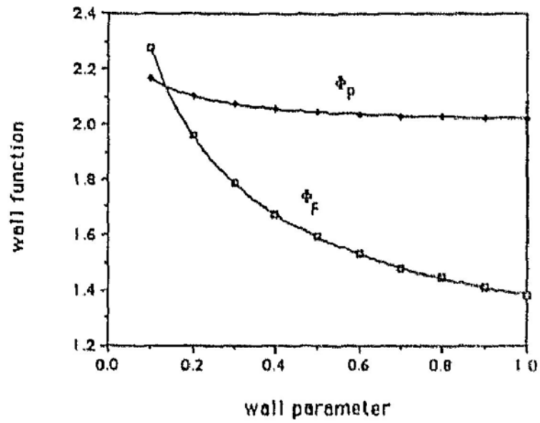
FIG. 2.22: \Phi , "wall function" en fonction de \eta , "wall parameter", pour les deux types de conditions aux limites ("force model" et "punch model"), extrait de [Théret et al., 1988]
