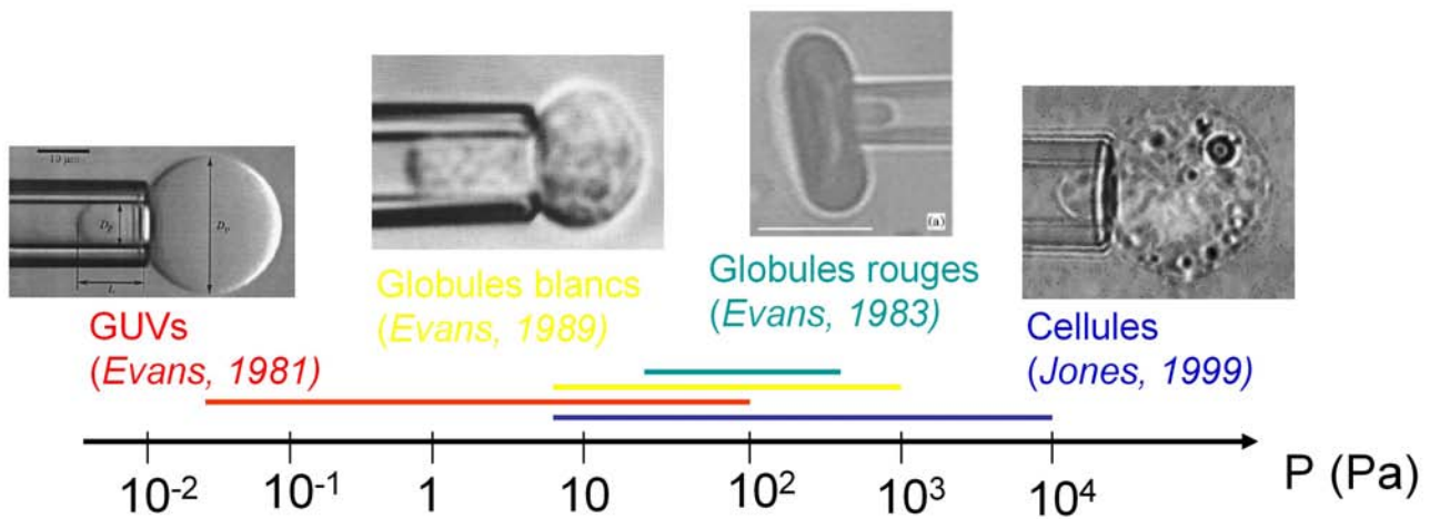
FIG. 2.23: Pressions caractéristiques d'aspiration pour des expériences sur différents types d'objets dont l'étude est rapportée dans [Kwok and Evans, 1981], [Evans and Yeung, 1989], [Evans, 1983], [Jones et al., 1999]
