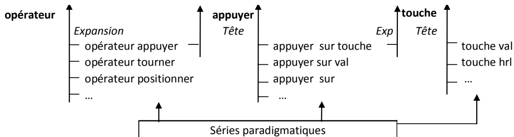
Figure 7.1 – Schéma d'un réseau de dépendances Syntax (extrait DORIS)
