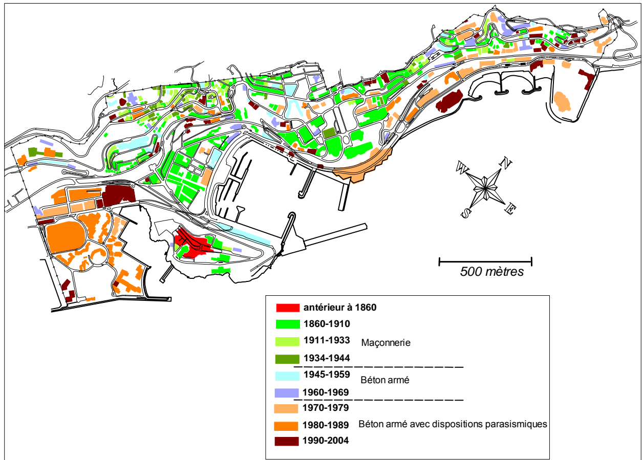
Figure 106 : Plan de Monaco avec les bâtiments ou blocs de bâtiments représentés par périodes et par procédés de construction : vert : maçonnerie; bleu : béton armé; marron orangé : béton armé avec dispositions parasismiques. Chacune de ces grandes périodes a été subdivisée en plusieurs catégories (nuances de la couleur) afin de tenir compte de l'âge et donc de la vétusté du bâti (Sources : DPEU – DEUC).
