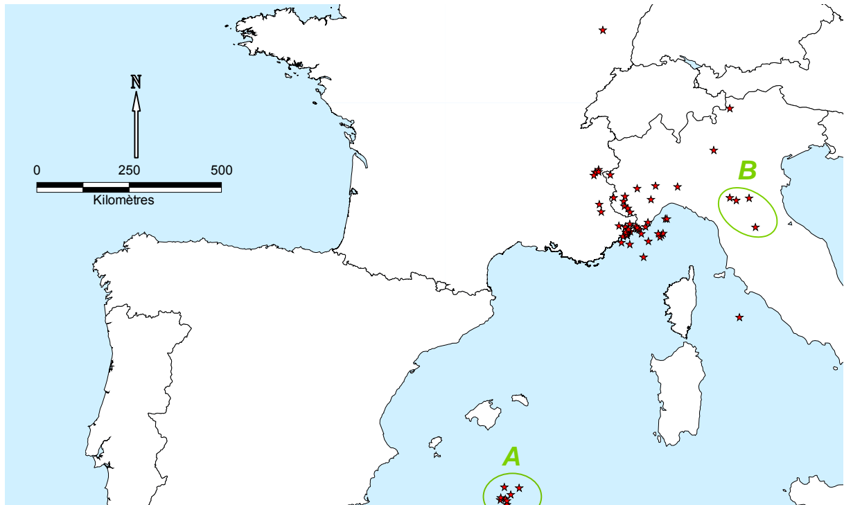
Figure 19 : Principaux séismes enregistrés sur la station de référence du Rocher de Monaco au cours de ces 7 dernières années pour une distance épacentrale inférieure à 800 km (données Renass). la zone A englobe la crise sismique d’Alger de mai 2003, la zone B le séisme du lac de Garde du 24 novembre 2004.
