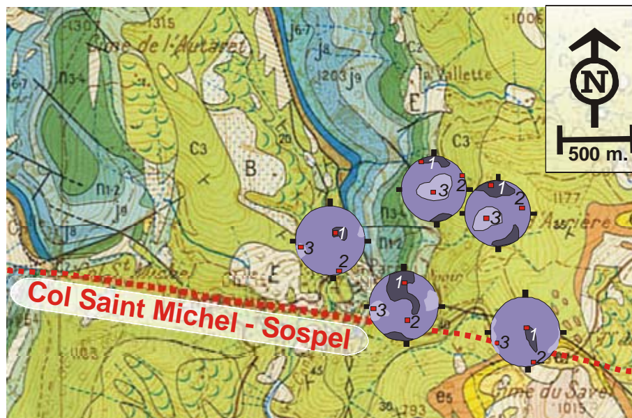
Figure 52 : Paléochamps de déformation relevés dans le crétacé supérieur chevauché par le Jurassique de l'écaïlle de la Rocca Seira au passage de l'alignement N100°E Col Saint Michel - Sospel (feuille Menton – Nice 1/50.000°, Gèze, 1968).
