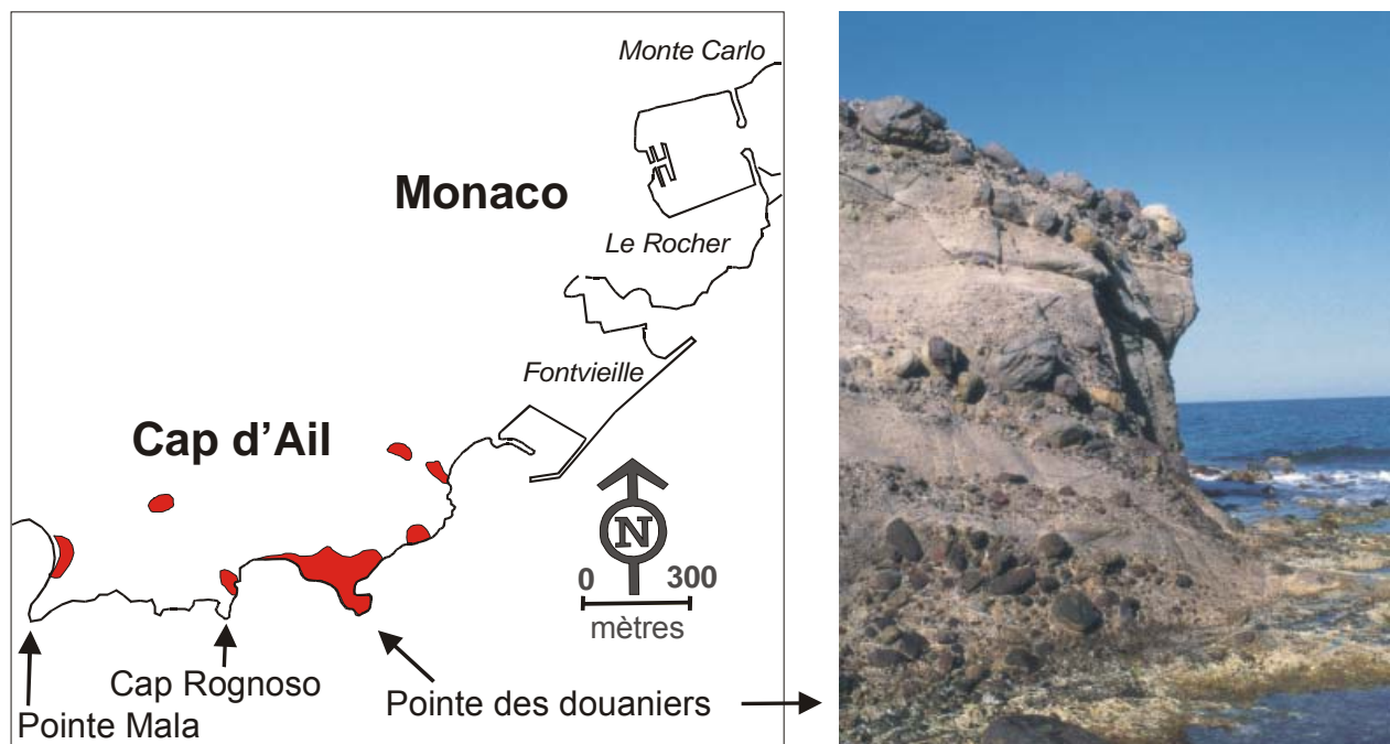
Figure 6 : Localisation géographique du corps magmatique effusif de Cap d'Ail visible en surface à la frontière ouest de Monaco (Gèze, 1968).
