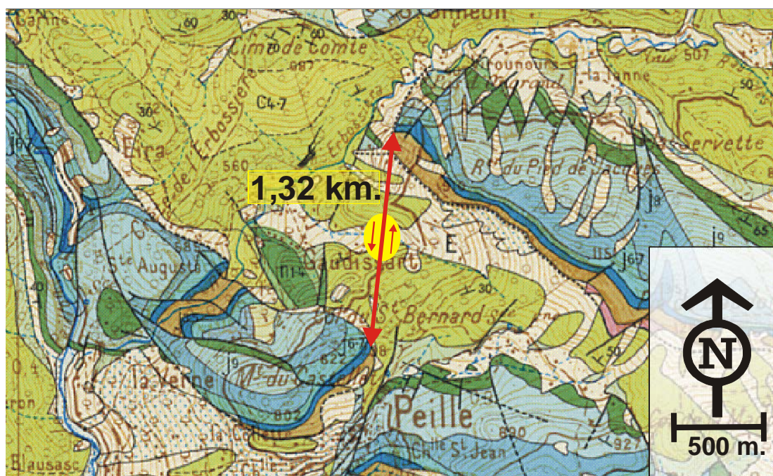
Figure 51 : Quantification du jeu fini horizontal du décrochement senestre de Peille – Laghet entre l'unité du Castellet - Santa Augusta et celle du Baudon (fond cartographique : feuille Menton – Nice 1/50.000 e , Gèze, 1968).
