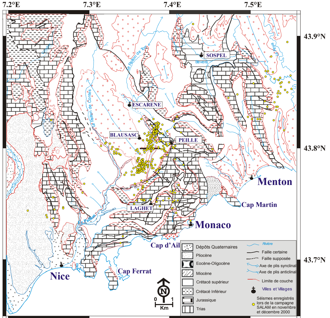
Figure 16 : Séismes de la crise de Blausasc situés dans le contexte géologique et structural de la région (Charreau, 2002).
