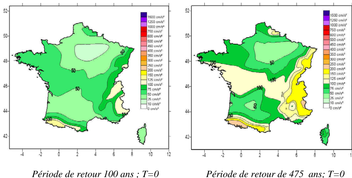
Figure 66 : cartes moyennes finales des accélérations attendues pour la France métropolitaine pour des périodes de retour de 100 ans et de 475 ans (zonage probabiliste Géoter, 2002).
