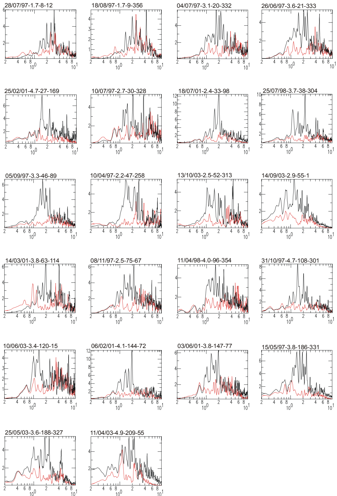
Figure 92 : rapports spectraux H / V séismes pour des événements enregistrés de 1997 à 2003 sur la station FONV en noir et MONA en rouge (AA/MM/JJ – magnitude - distance épicentrale - azimut).
