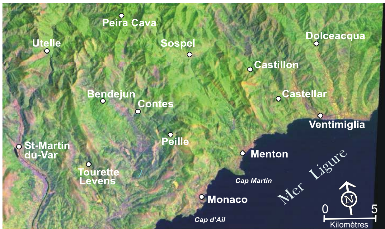
Figure 20 : Cliché Landsat 5 du 23 juillet 1984, traitements en fausses couleurs à partir des images des canaux 4,5 et 6. © Eosys – DEUC.
