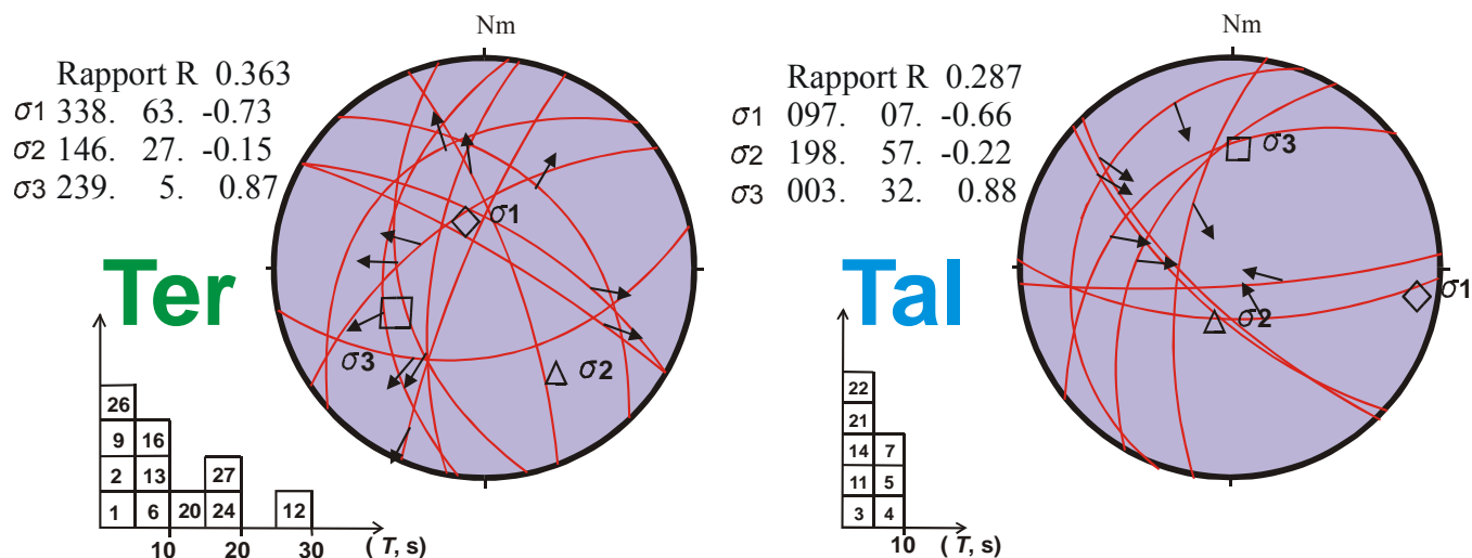
Figure 61 : diagrammes des inversions des mécanismes au foyer pour les zones ter et tal du secteur d'étude
