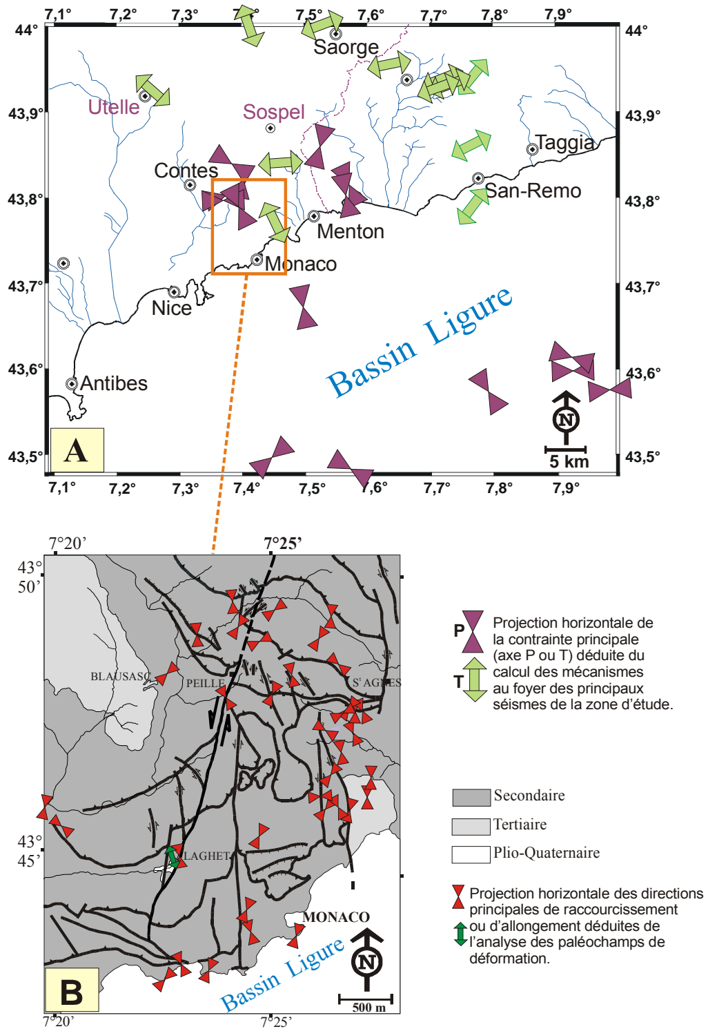
Figure 64 : Projections horizontales des champs de contraintes principaux des séismes pour le sud des Alpes maritimes franco-italiennes (A) et des champs de déformations principaux de la déformation fragile finie autour de Monaco (B).
