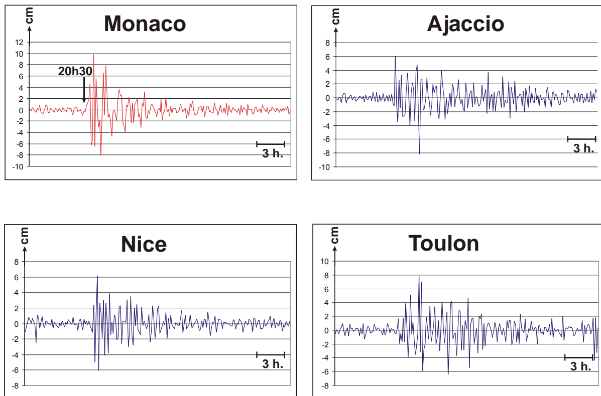
Figure 105 : Enregistrements le 21 mai 2003 du tsunami lié au séisme de Boumerdès par les marégraphes du SHOM situés sur les côtes de la mer Ligure.
