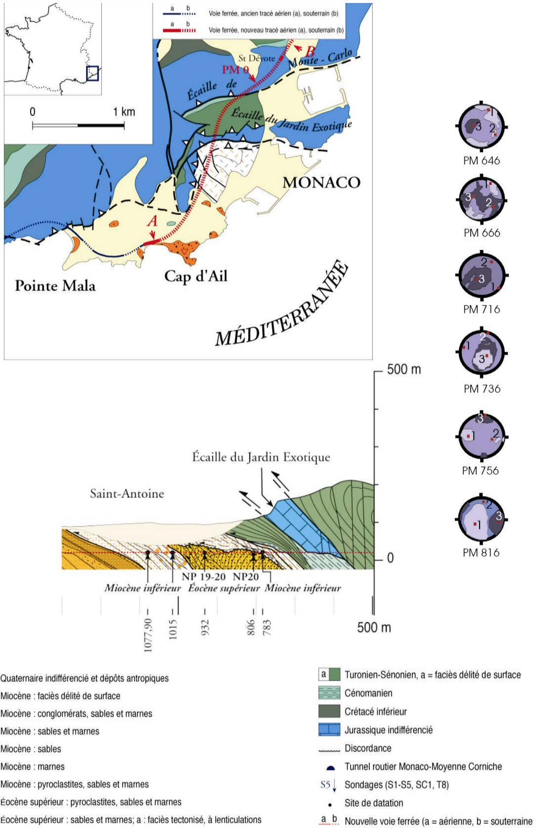
Figure 56 : Carte et coupe géologique réalisées lors du creusement de la galerie de reconnaissance SNCF à Monaco (Ivaldi et al. , 2003) et stéréogrammes des miroirs striés mesurés.
