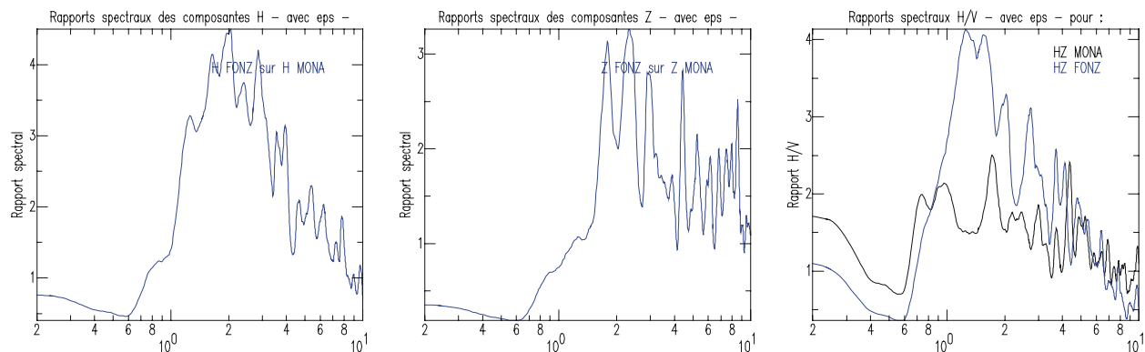
Figure 89 : Rapports spectraux horizontaux, verticaux et rapport H/V sisme des ondes T du séisme principal de magnitude 6.8 de la crise sismique d'Alger du 21 mai 2003.
