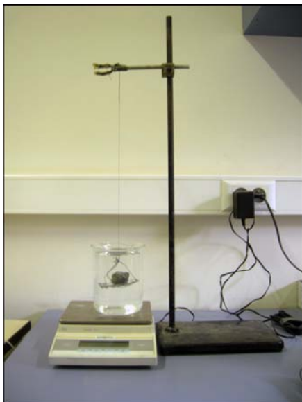
Figure 2.7 Photographie et schéma du dispositif permettant la mesure de la masse volumique des clastes > -4 φ (16 mm) par immersion.
