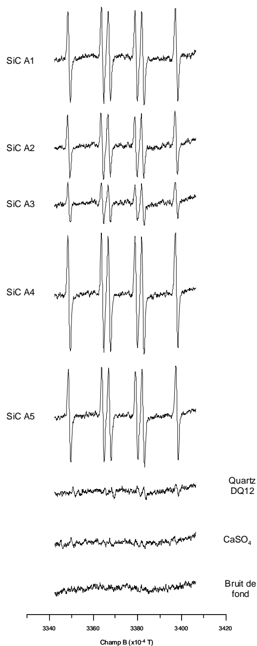
Figure 58 : Signaux RPE de l'adduit [DMPO-COO] • obtenus en présence des poudres industrielles de SiC. L'intensité du signal est proportionnelle à la quantité de radicaux libres COO • générés
