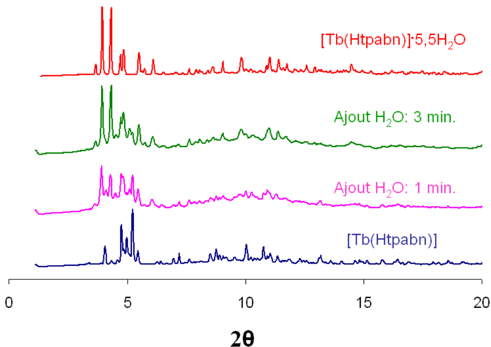
Figure 56 – Etude de l'absorption de molécules d'eau par le complexe anhydre [\text{Tb}(\text{Htpabn})] . Spectres mesurés sur le diffractomètre MAR345 image plate detector pour la radiation K\alpha du Mo ( \lambda = 0,71\text{\AA} )
