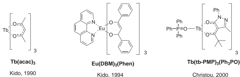
Figure 28 – Complexes de lanthanides utilisés pour la mise au point de composés électroluminescents.
