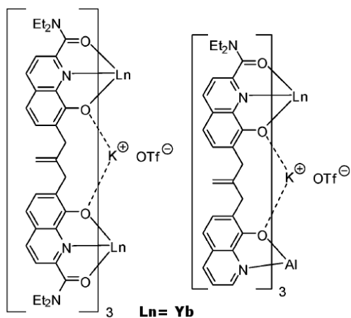
Figure 93 – Hélicates homo- et hétérodimétalliques luminescents [234].
