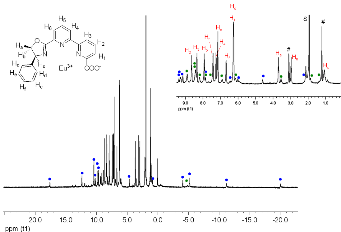
Figure 124 – Spectre RMN ^1\text{H} du complexe \text{Eu}(\text{bis}-(\text{Phoxbipyra})) dans \text{CD}_3\text{CN} . Les protons rouges correspondent à l'espèce C , les signaux verts et bleus, aux espèces C' et B , respectivement ( \text{CD}_3\text{CN} , 400MHz, 298K).
