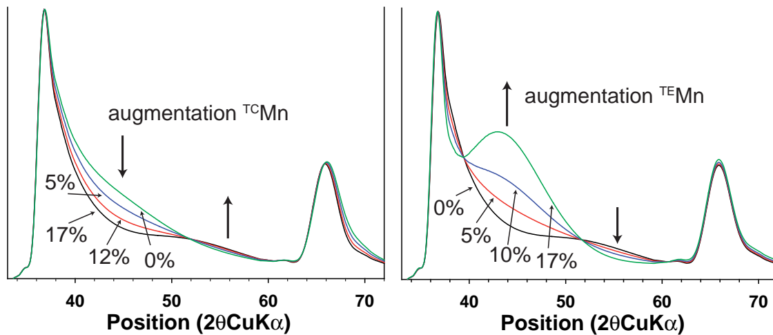
(a) Quantité de {}^{\text{TC}}\text{Mn} variée de 17% à 0%. (b) Effet de la migration de {}^{\text{TC}}\text{Mn} en {}^{\text{TE}}\text{Mn} . A 17%, tout le {}^{\text{TC}}\text{Mn} a migré en position {}^{\text{TE}}\text{Mn} .
