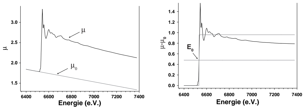
(a) Soustraction de \mu_0
