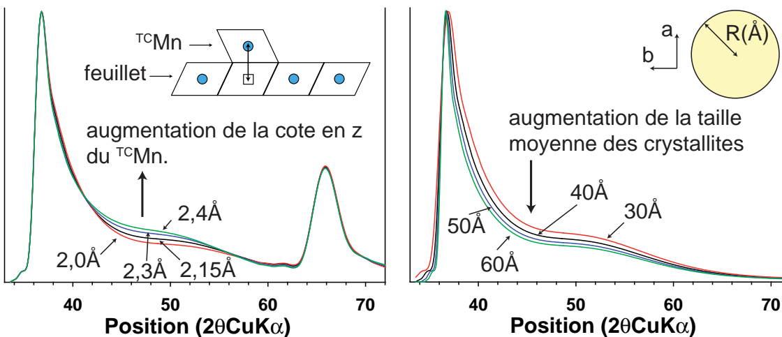
(e) Sensibilité à la cote en z du manganèse inter-foliaire, variée de 2,0 Å à 2,4 Å. (f) Sensibilité à la taille des cristallites (valeur : rayon moyen) .
