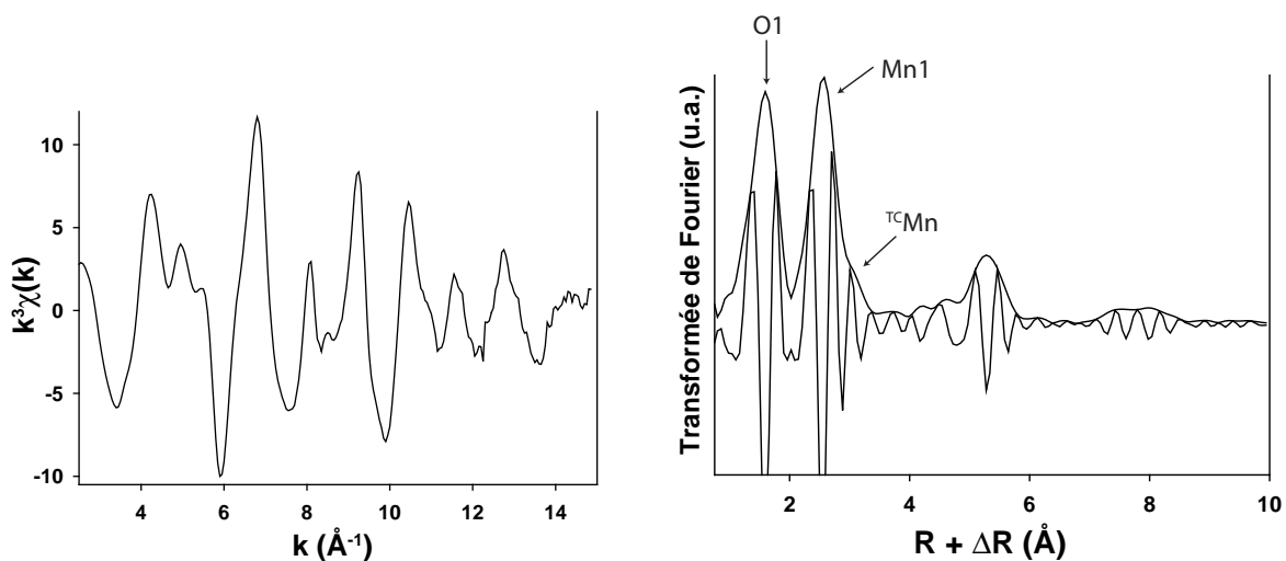
(d) Fonction \chi(k) obtenue.
