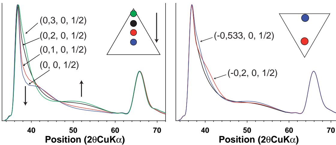
(c) Position des molécules d'eau variée de (0, 0, 1/2) à (0,3, 0, 1/2) . Schéma : illustration de la position par une vue selon c^* . (d) Déplacement des molécules d'eau vers deux positions symétriques : (-0,2, 0, 1/2) et (-0,533, 0, 1/2) .
