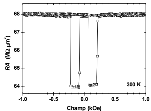
Figure 4.10 : Cycles magnétorésistifs des JTMs Fe/Fe 3 O 4 /MgO/Co à 300 K.
