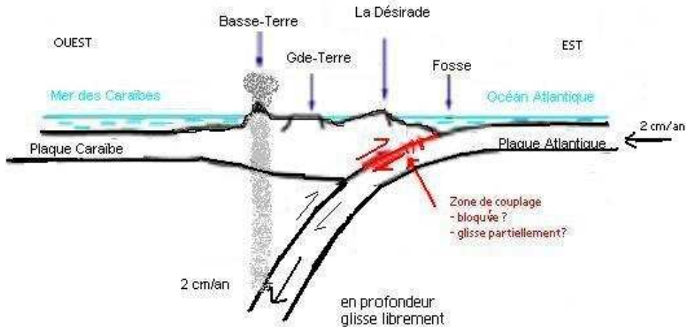
Figure 1.2. Schéma de la subduction des Petites Antilles.
