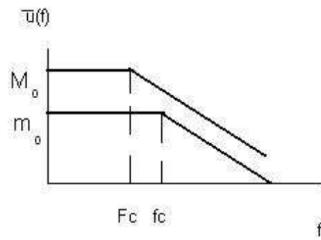
Figure 4.1. Schéma montrant les spectres en déplacement du séisme cible et de la fonction de Green empirique. Le moment sismique et la fréquence coin du séisme cible et de la FGE sont représentés par (M_0, F_c) et (m_0, f_c) respectivement (d'après Ruiz, 2007).
