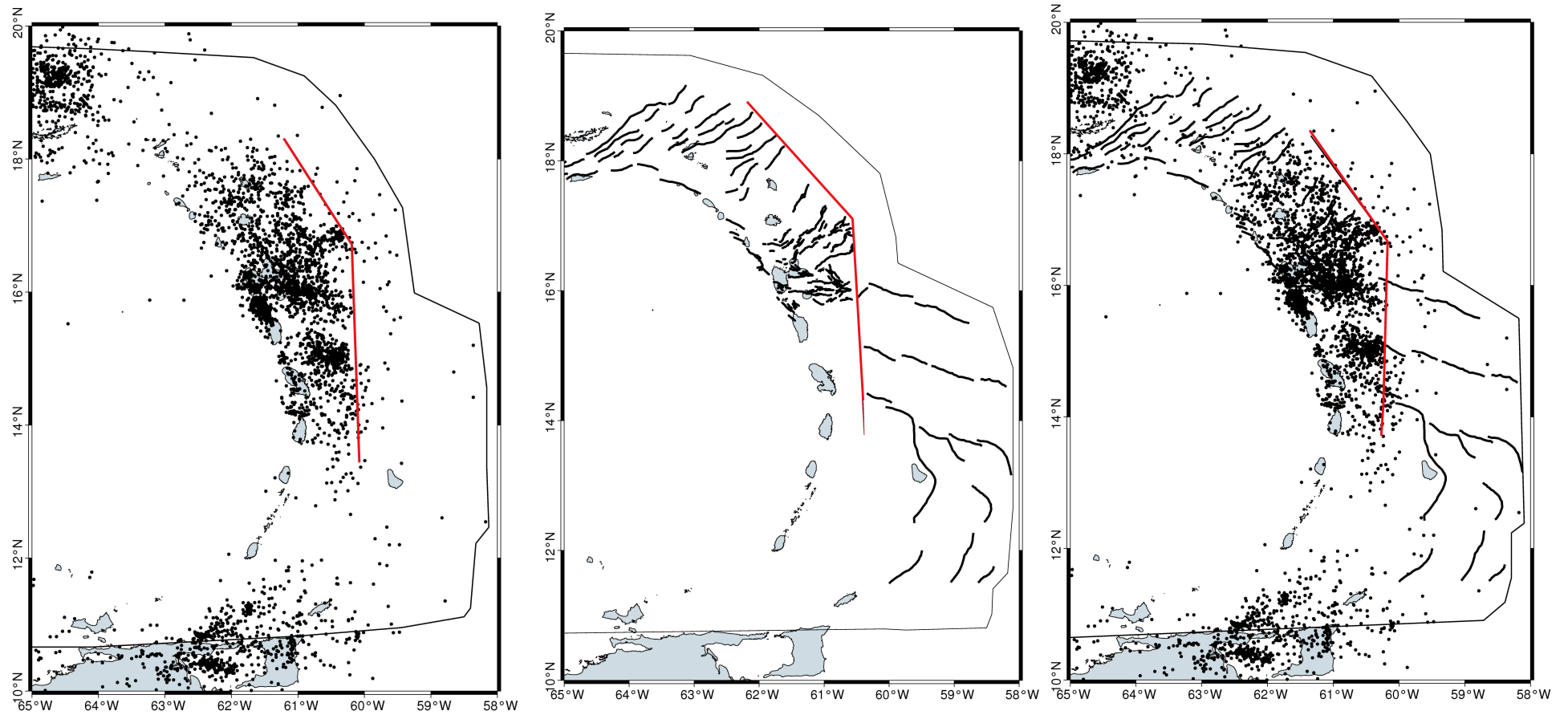
Figure A. 4. Relations entre la sismicité superficielle (< 50 km, catalogue CDSA) et la tectonique active (Feuillet et al., 2000).
