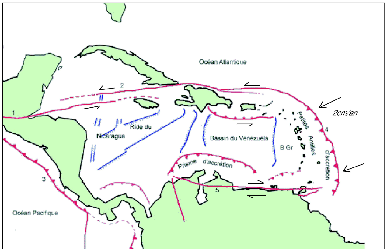
Figure 1.4. Schématisation de la géodynamique actuelle de la plaque Caraïbe. [1] Faille de Motagua-Polochie, [2] Faille Orientale, [3] Subduction de la plaque des Cocos, [4] Subduction de la plaque Amérique, [5] Faille de El Pilar.
