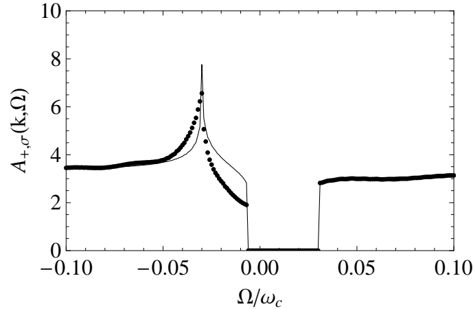
FIGURE 5.5 – Fonction spectrale pour de fortes interactions coulombiennes ( K_c = 0.2 ) avec a(k - k_F) = 0.006 en l'absence (trait plein) et en présence d'écrantage (point) avec \omega_{Sc}/\omega_c = 0.005 .
