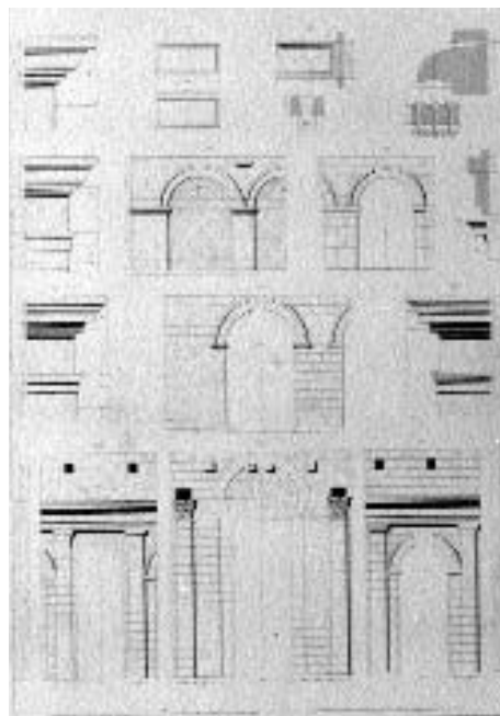
Fig. 306. « Détails des façades principales et latérales » du théâtre d'Orange. Dessins d'A.-N. CARISTIE, Monuments... , op. cit. [pl. xxxvi], 1856.
