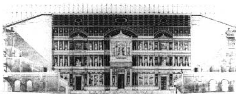
Fig. 250. « Étude de reconstitution de la partie centrale de la scène du théâtre d'Arles ». Dessin de J. FORMIGÉ, 1912. (Salon des Artistes de France en 1922.)
