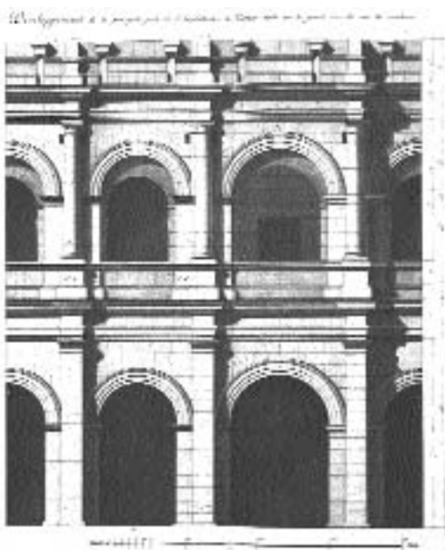
Fig. 204. « Développement de la principale porte de l'Amphithéâtre de Nîmes située sur le grand axe du côté du couchant ». Relevé de Ch.-L. CLÉRISSEAU, op. cit. [pl. xvi], 1778.
