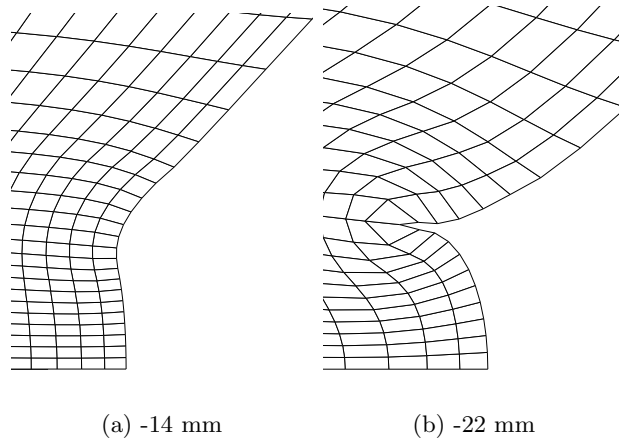
Figure IV.6 : Déformées en compression : formation des plis avec l'utilisation d'éléments linéaires.
