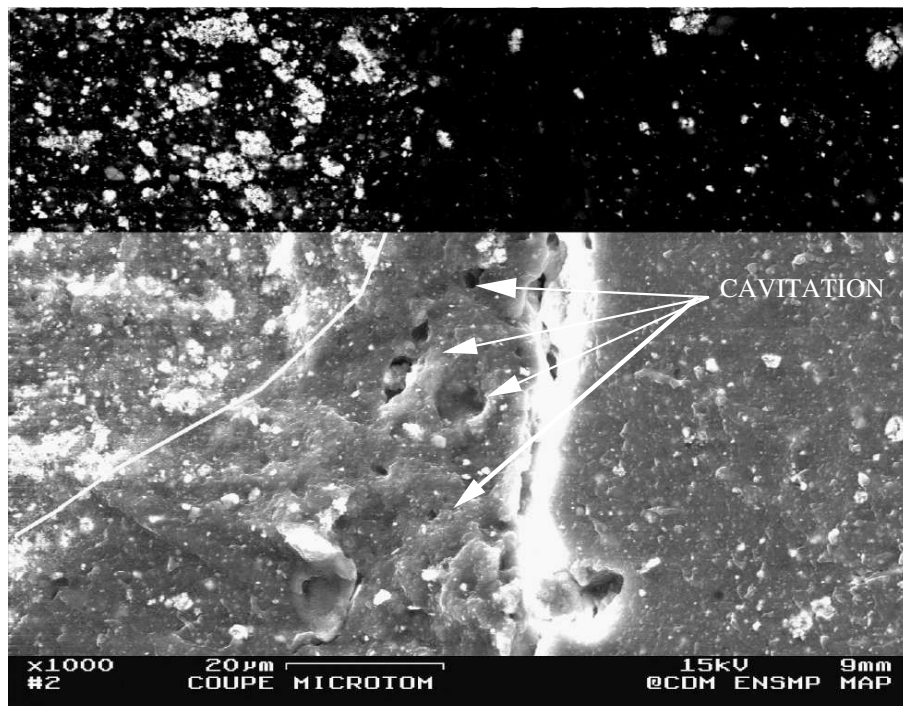
Figure III.20 : Zone de cavitation au-dessus de la particule.
