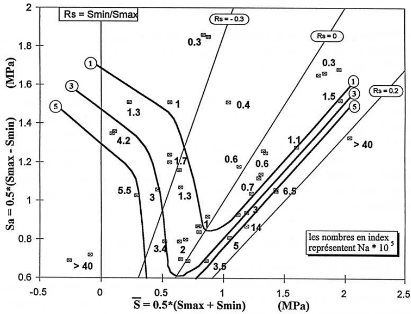
Figure V.6 : Diagramme de Haigh à deux paramètres, \Delta\sigma et \bar{\sigma} pour la prévision de la durée de vie des essais de fatigue en traction-compression sur Diabolos.
