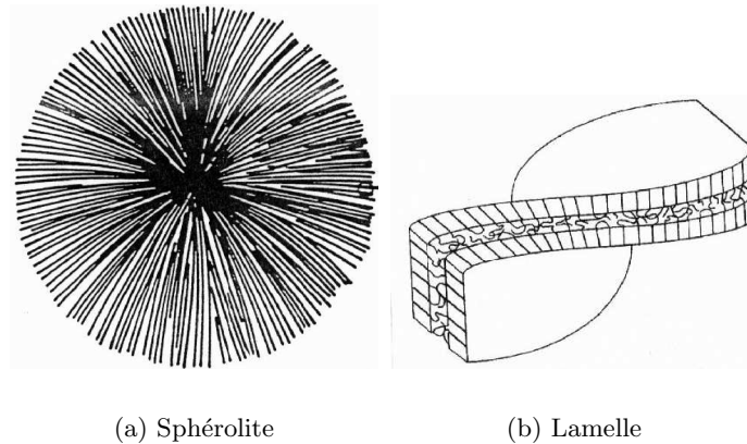
Figure I.13 : Schématisation de la superstructure sphérolitique et des lamelles qui la composent
