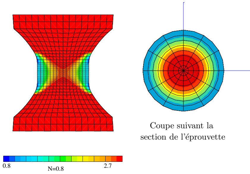
Figure VI.7 : Localisation de l'amorçage en traction-compression cyclique et torsion statique de 60^\circ sur Diabolo pour le critère C_{IBC} .
