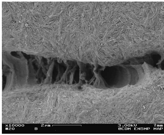
Figure III.27 : Crazing observé dans le PET[26].
