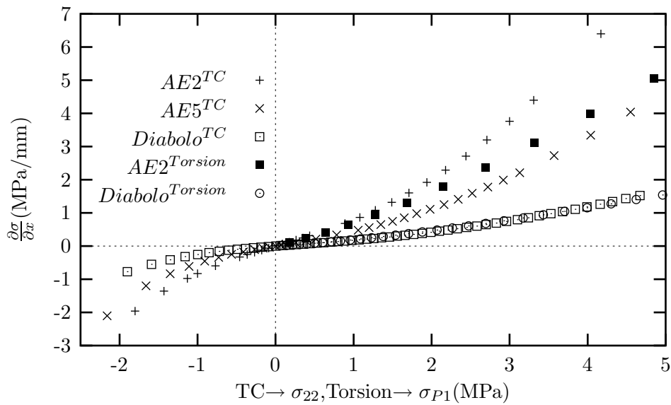
Figure IV.18 : Evolution des gradients de contrainte dans la zone d'amorçage pour chaque type d'essai.
