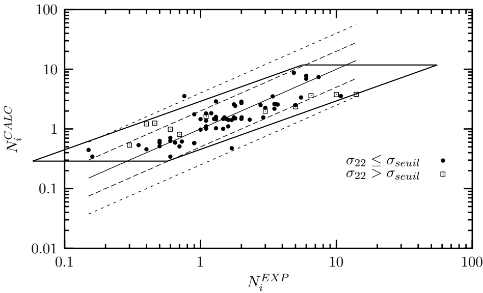
Figure VI.11 : Dispersion obtenue après optimisation du modèle. Les lignes en pointillés indiquent un rapport 2 puis 4 entre durée de vie expérimentale et durée de vie calculée. Durée de vie indiquée en 10^5 cycles.
