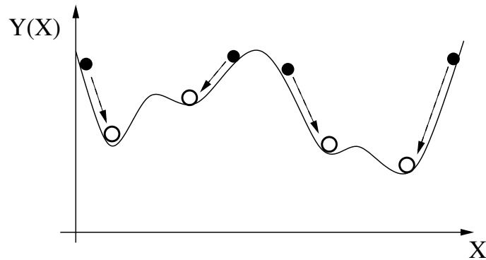
Figure V.14 : Algorithmes déterministes : dépendance vis-à-vis du point de départ. Rond plein : point de départ. Cercle : solution proposée à la fin de l'optimisation.
