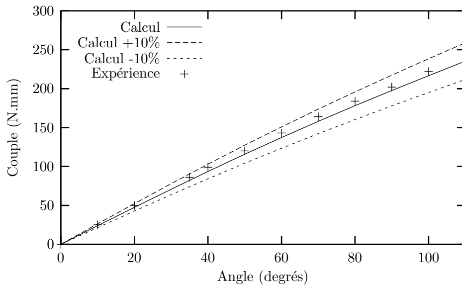
Figure IV.15 : Comparaison calcul-expérience : torsion sur AE2
