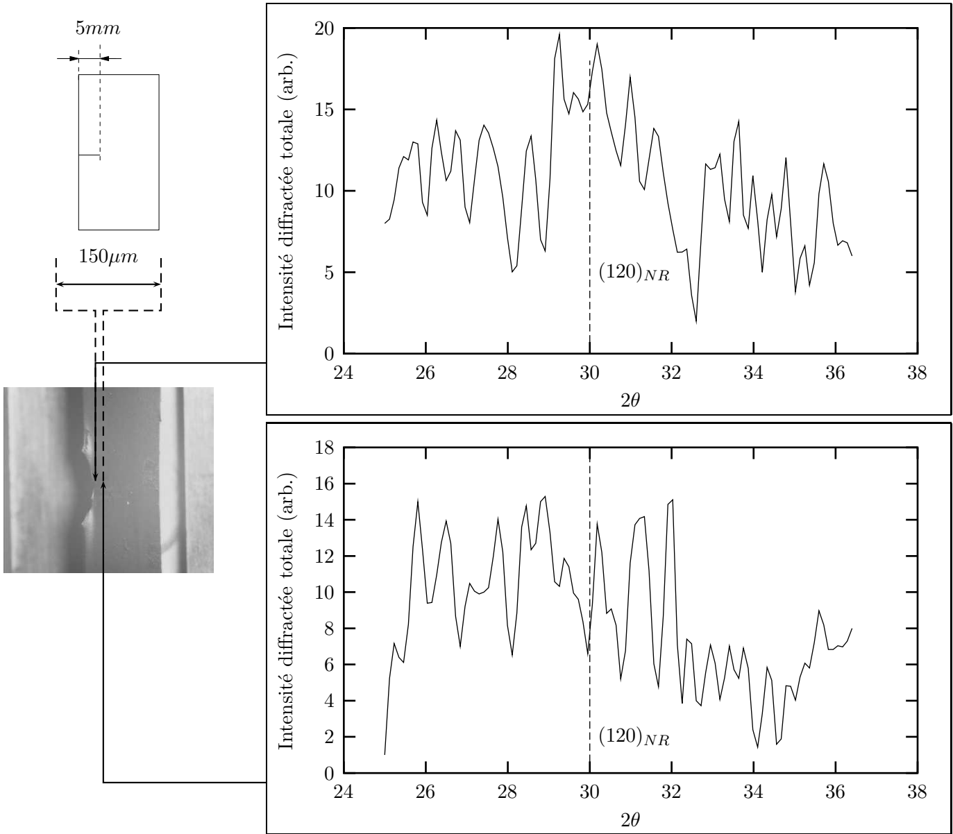
Figure I.23 : Mesures de l'intensité diffractée en \theta - 2\theta et micro-foyer
