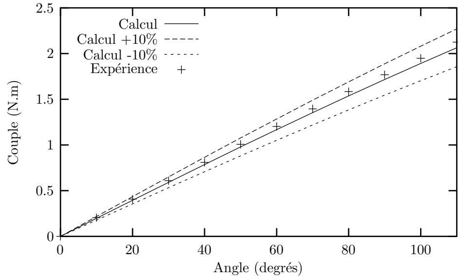
Figure IV.14 : Comparaison calcul-expérience : torsion sur Diabolo
