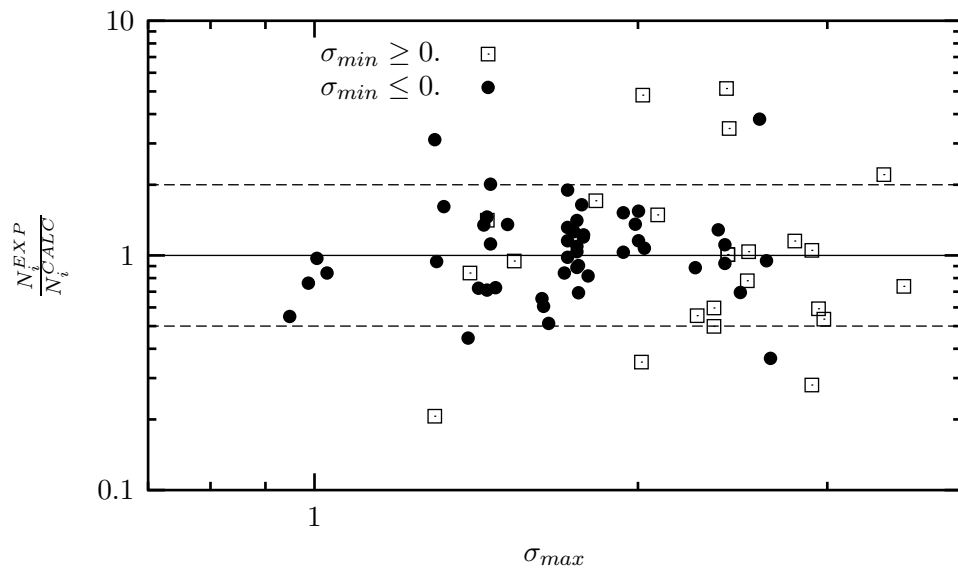
Figure V.18 : Evolution du rapport entre durée de vie expérimentale et calculée en fonction de la contrainte maximale atteinte au cours de l'essai.
