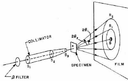
Figure I.15 : Dispositif utilisé pour la diffraction X
