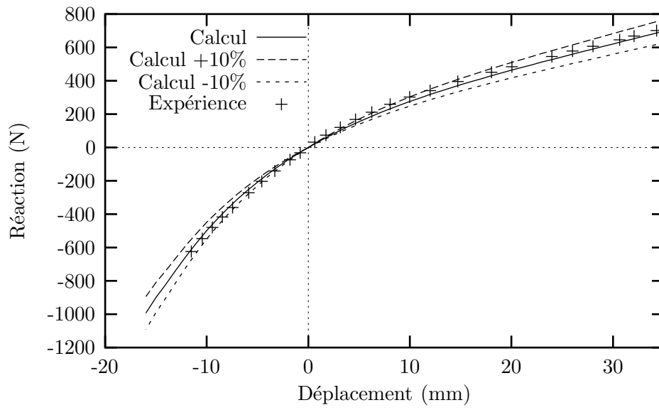
Figure IV.3 : Comparaison calcul-expérience : traction-compression sur diabolo
