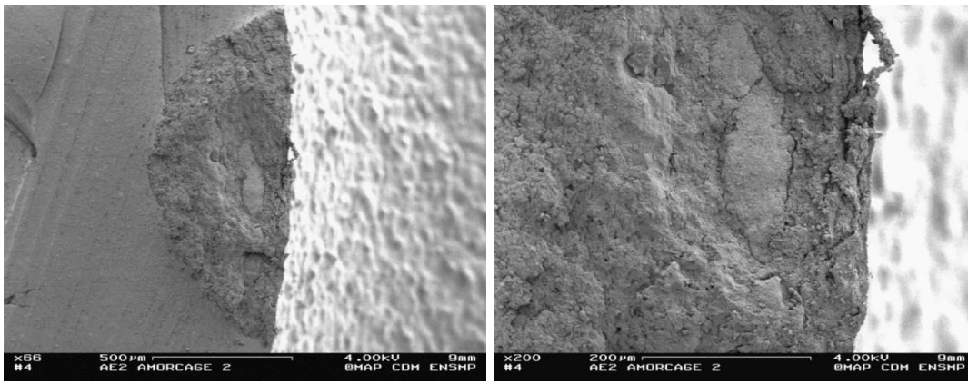
Figure III.39 : Faciès de rupture sur éprouvette axi-symétrique AE2 (essais AE2-TC-15). Amorçage sur un agglomérat de noirs de carbone
