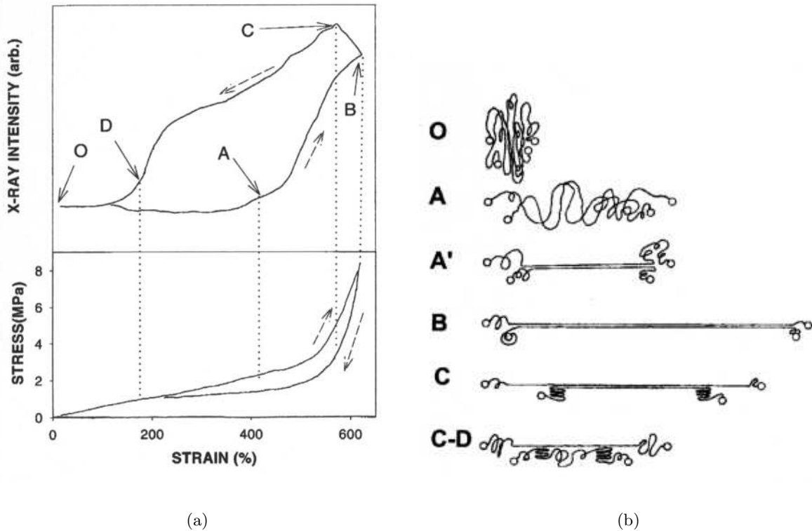
Figure I.27 : Mesures de diffraction X et essais de traction simultanés [49].
