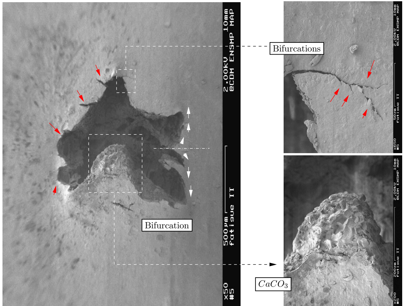
Figure III.22 : Amorçage à R positif (essais DIAB-TC-39n). Mise en évidence de la bifurcation des fissures.
