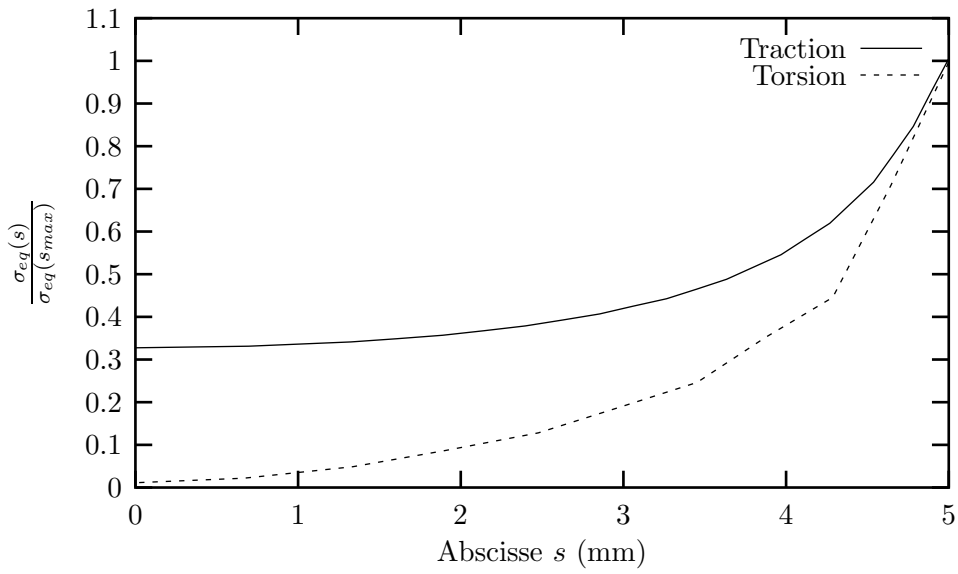
Figure VI.34 : Evolution du rapport \sigma_{eq}(s)/\sigma_{eq}(s_{max}) sur le lisset lbas pour une éprouvette AE2 et torsion et traction-compression à même niveau de \sigma_{eq}(s_{max}) .
