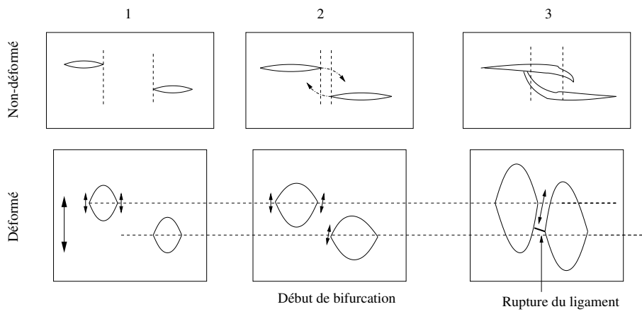
Figure III.56 : Schématisation du processus de coalescence de fissures en fatigue.
