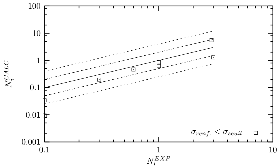
Figure VI.32 : Dispersion obtenues en appliquant le critère C_{CPA} aux essais de torsion sur éprouvettes AE5. Durée de vie indiquée en 10^5 cycles. .
