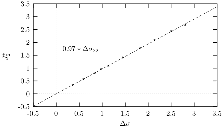
Figure VI.2 : Relation entre l'amplitude de contrainte et J_2^* pour les essais uniaxiaux.
