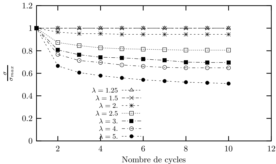
Figure I.9 : Evolution de la contrainte maximale atteinte à chaque cycle pour un essai de traction cyclique R = 0 et déformation imposée. Les résultats sont normalisés par rapport à la contrainte maximale atteinte à la première traction.
