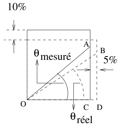
Figure III.48 : Fissures sur AE2 en torsion 0-100° (essai AE2-TOR-15).
