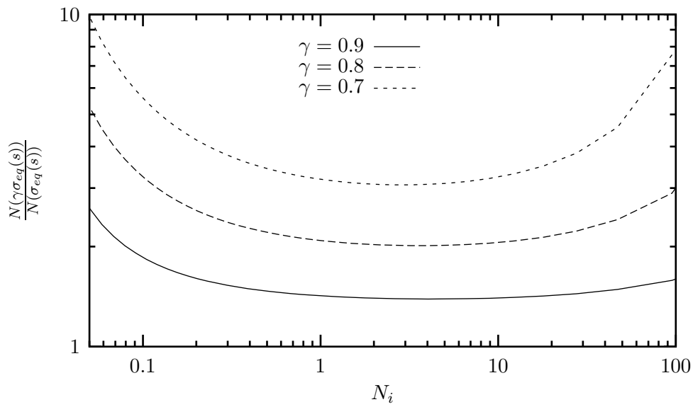
Figure VI.35 : Sensibilité de la durée de vie calculée à la variation de contrainte équivalente pour des essais sans renforcement.
