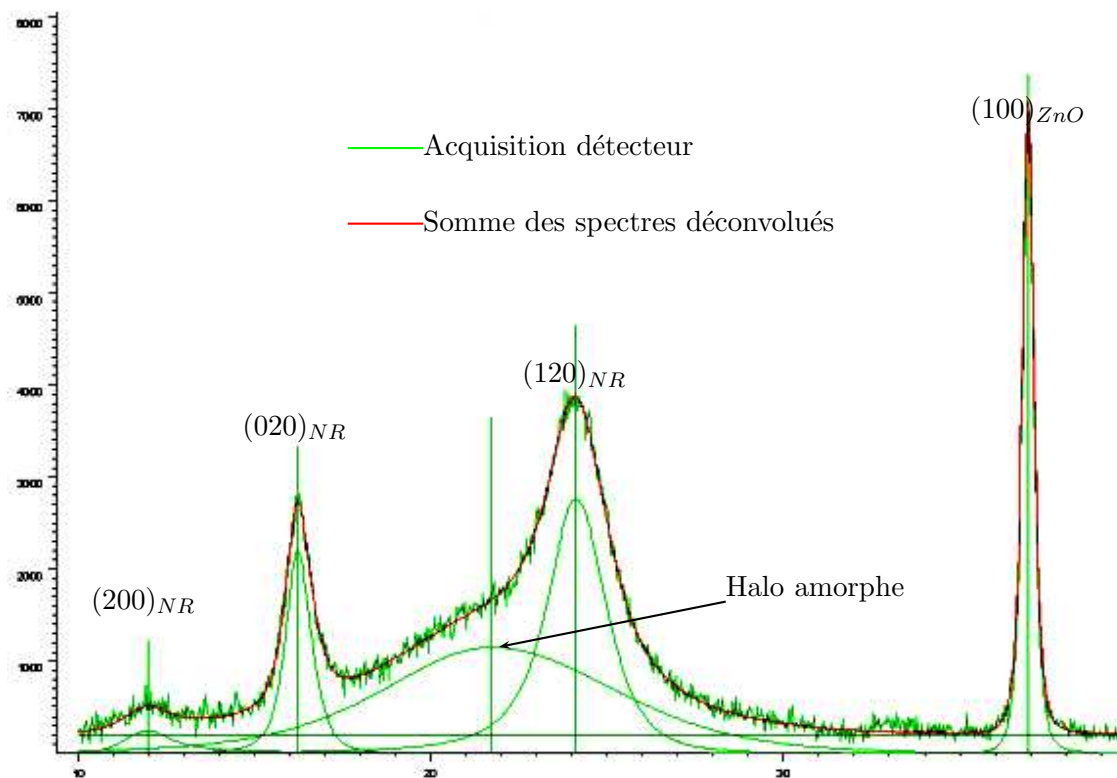
Figure I.18 : Exemple de déconvolution de spectres ( \lambda = 5.2 ).
