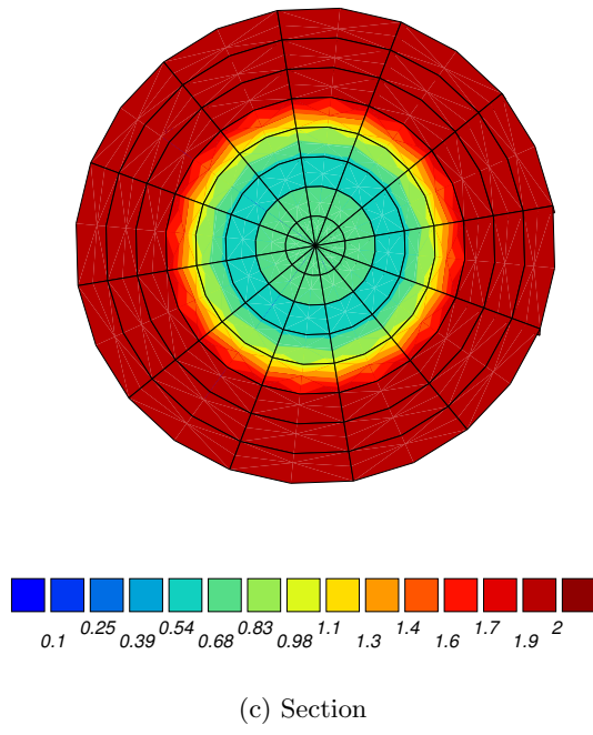
Figure VI.28 : Cartographie du nombre de cycles à l'amorçage en torsion statique et traction-compression. Essai DIAB-TSTTC-9 .
