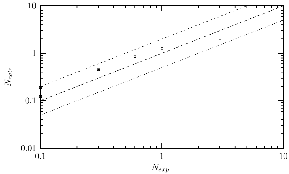
Figure VI.8 : Comparaison entre durées de vie expérimentales et durées de vie calculées en traction-compression sur AE5. Critère C_{IBC} .
