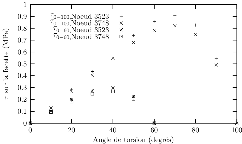
Figure III.53 : Evolution du cisaillement (Cauchy) sur les facettes matérielles associées à \vec{\sigma}^P au cours d'un essai de torsion.
