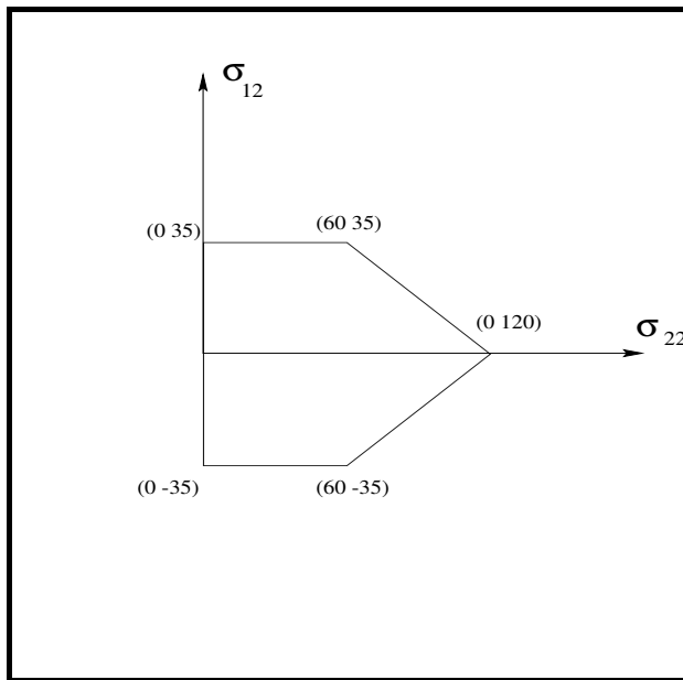
Figure A-III.2 : Chargement imposé
