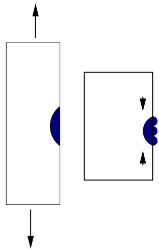
Figure III.32 : Origine de la formation des plis : flambements locaux en présence d'une zone de déformation visqueuse permanente.
