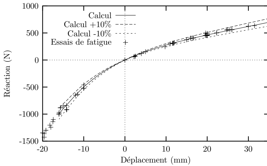
Figure IV.4 : Comparaison calcul-expérience : Résultats de fatigue sur diabolo
