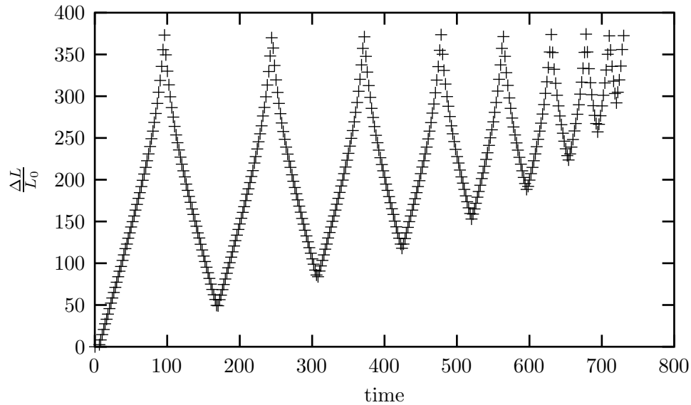
Figure I.24 : Pilotage en déformation .
