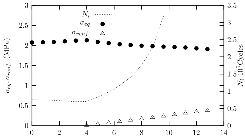
Figure VI.27 : Evolution de \sigma_{eq} , \sigma_{ref.} et N_i suivant la direction radiale dans la section de l'éprouvette.
