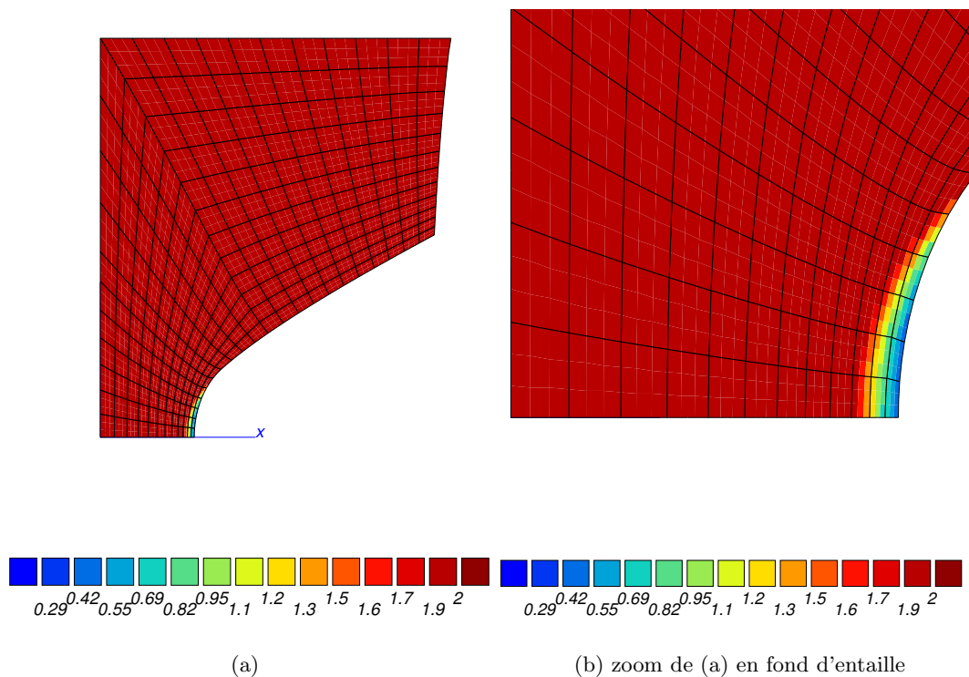
Figure VI.18 : Cartographie du nombre de cycles à l'amorçage en traction-compression sur AE2. Essai AE2-TC-18.
