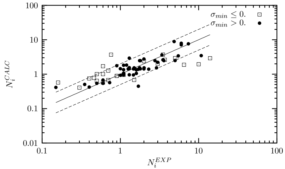
Figure V.17 : Dispersion des résultats de fatigue uniaxiale.
