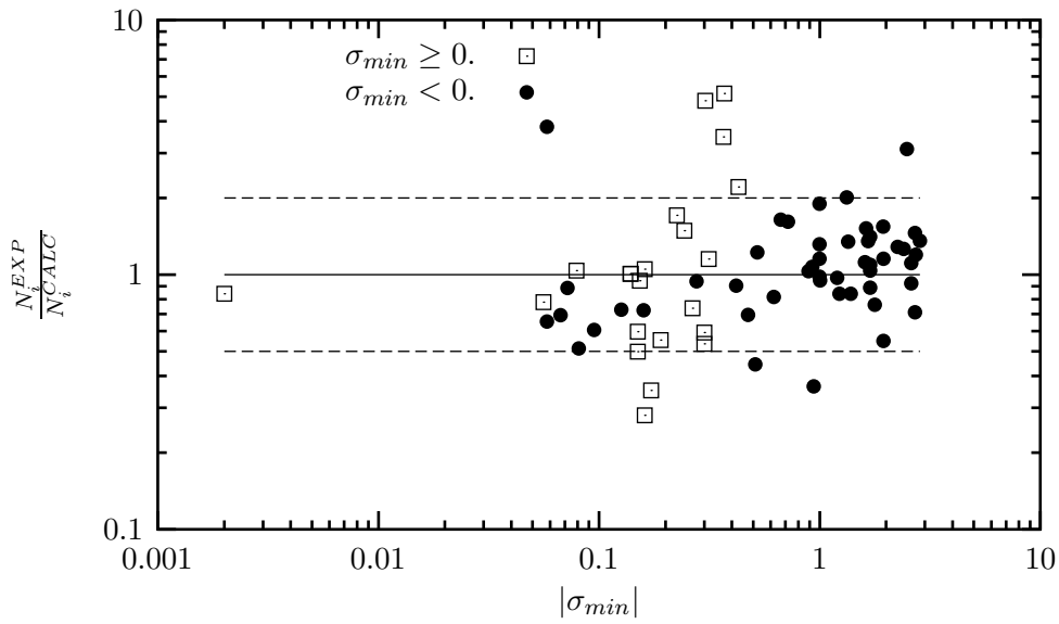
Figure V.19 : Evolution du rapport entre durée de vie expérimentale et calculée en fonction de la valeur absolue de la contrainte minimale atteinte au cours de l'essai.
