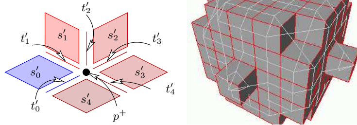
FIG. 6.4 – Ombrelle sur surface discrète et reconstruction polyédrique de surface discrète en 3D. A gauche est représentée la boucle autour de la 0-cellule p^+ traversant le bel s'_0 . Cette boucle forme le chemin de bels s'_0, \dots, s'_4 , séparés par les 1-cellules ( t'_i ). A droite, le graphe de bel-adjacence est surimposée sur le dessin de la surface discrète. On vérifie que les boucles ou ombrelles définissent les faces polyédriques de ce graphe.
