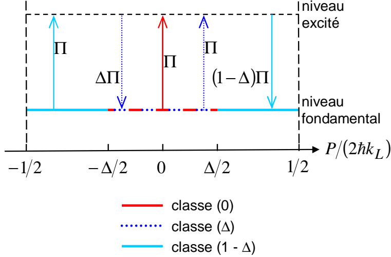
FIG. 3.7 – Représentation schématique des échanges par émission spontanée entre les classes de population (0), (Δ) et (1 - Δ). Sur le dessin, les différentes classes sont localisées par rapport à l'impulsion de leurs atomes. Cette représentation, périodique en P , est ici restreinte à la première zone de Brillouin [-\hbar k_L/2; +\hbar k_L/2[ ( [-\hbar k_L; +\hbar k_L[ en unités physiques). Les valeurs attachées aux flèches sont les taux de transfert entre chaque classe du niveau fondamental et le niveau excité.
