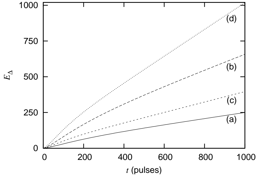
FIG. 3.10 – Energie totale E_{\Delta} de la classe d'atomes ( \Delta ) en fonction du temps, donnée par l'équation (3.29), et pour les cas (a–d) de la figure 3.5. Les paramètres D_q et t_s sont donnés par le “fit” résumé dans le tableau 3.2.
