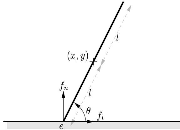
FIG. A.1: Le problème de Painlevé : une barre homogène glissant sur le sol.
