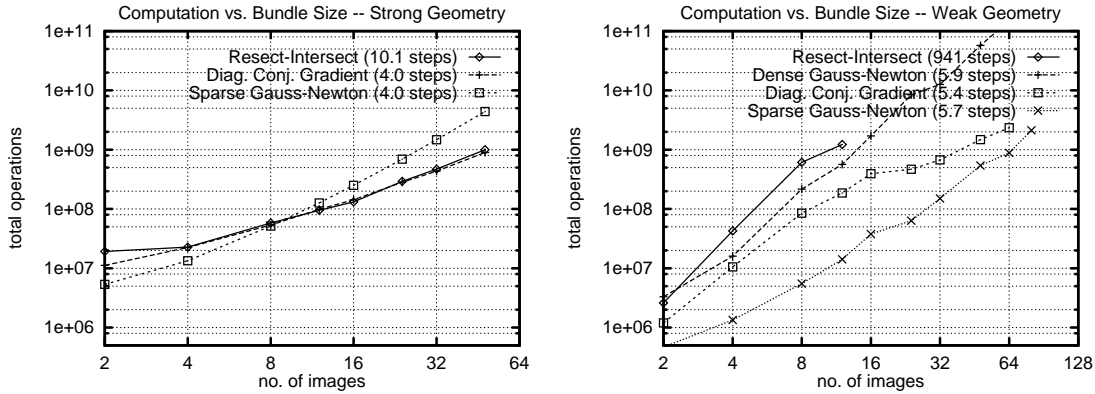
FIG. 8.2 – L'efficacité relative des algorithmes d'ajustement de faisceaux a une forte dépendance sur la géométrie du problème. À gauche: les algorithmes simplistes comme l'alternance classique résection - intersection marchent bien quand la géométrie est forte – ici, une nuage sphérique de points 3-D, contournée par un quart de cercle des caméras qui voient tous les points. À droite: quand la géométrie devient plus faible – ici une ligne de caméras qui voient chacune une zone locale d'une bande étendue de points, pour simuler un « strip » de photogrammétrie aérien – les méthodes simplistes deviennent trop inefficaces, et il faut adopter un méthode de type Newton qui exploite la structure du Hessien. Voir la référence [TMHF00] pour plus de détails.
