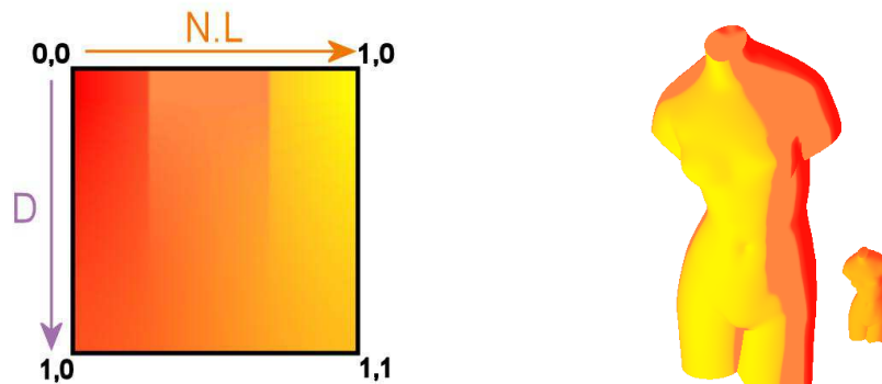
FIG. 2.7 – Xtoon : (à gauche) une texture 2d est utilisée pour contrôler l'éclairage ( N.L ) en fonction d'un paramètre de détail D . Par exemple (à droite) D peut être la profondeur depuis la caméra.
