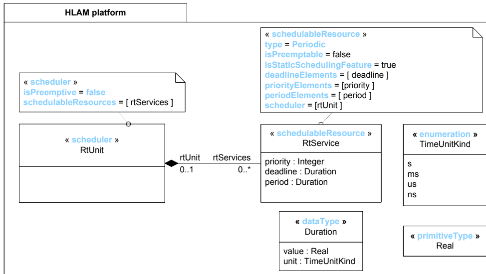
FIG. 7.2 – Extrait du modèle de domaine de la plate-forme HLAM utilisé pour produire le profil HLAM
