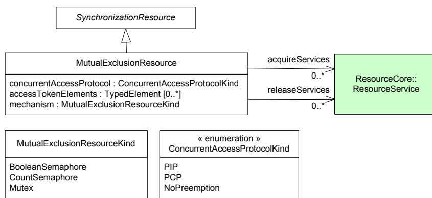
FIG. 6.14 – Description des ressources d'exclusion mutuelle
