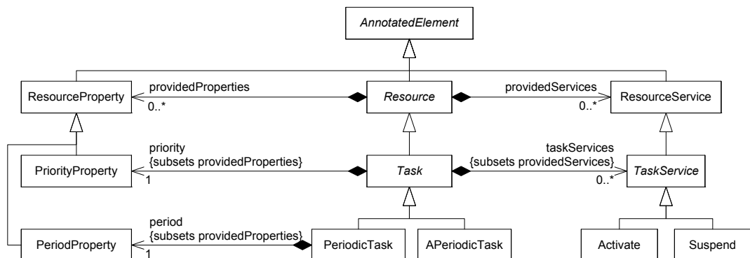
FIG. 3.4 – Agencement hiérarchique du modèle de domaine
