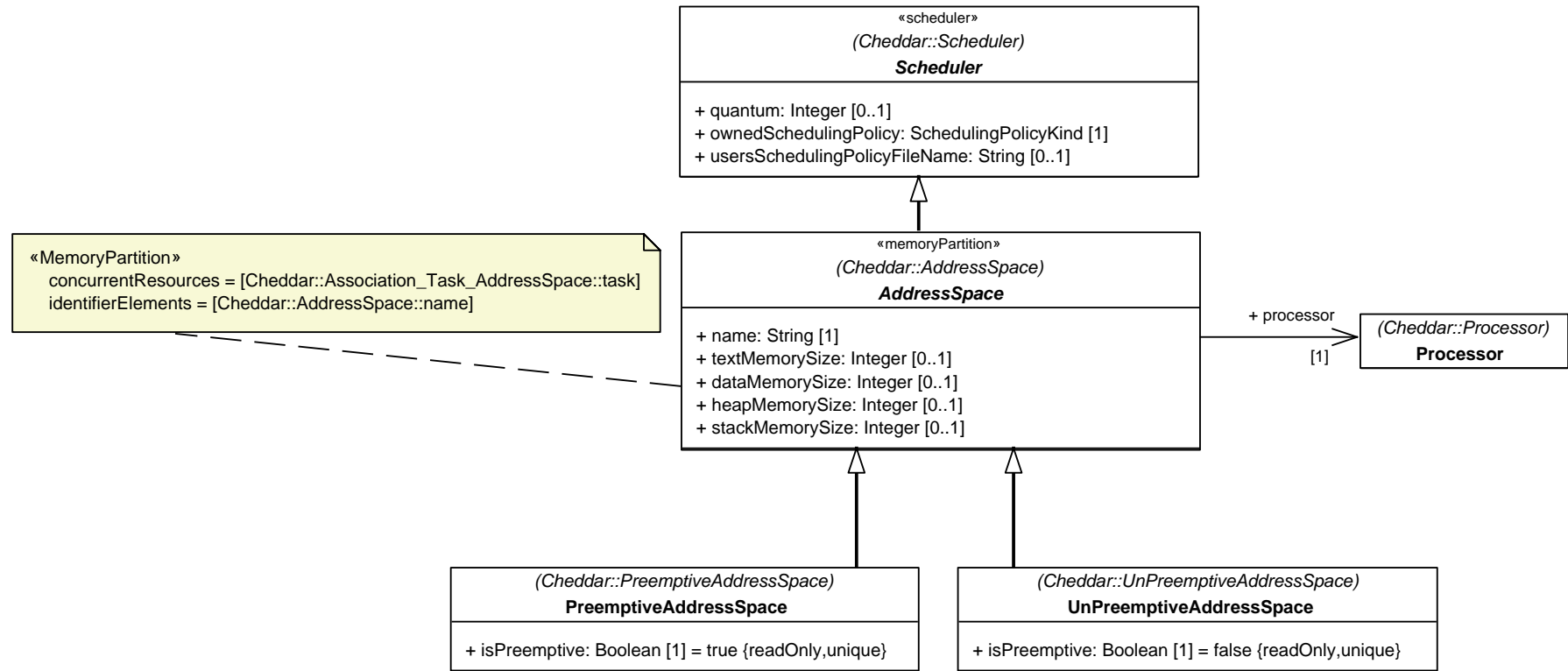
FIG. D.4 – Modélisation des partitions mémoires dans CHEDDAR
