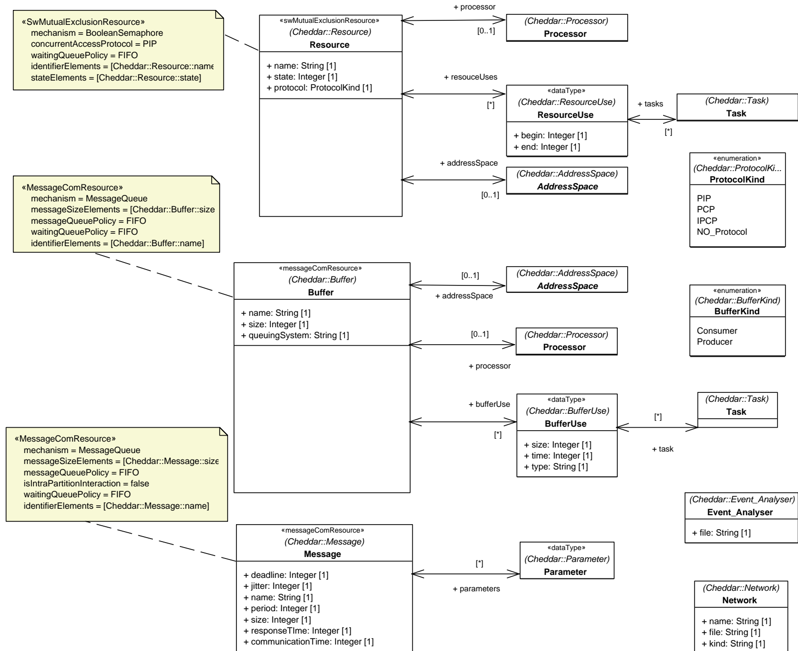
FIG. D.5 – Modélisation des ressources d'interaction du modèle CHEDDAR
