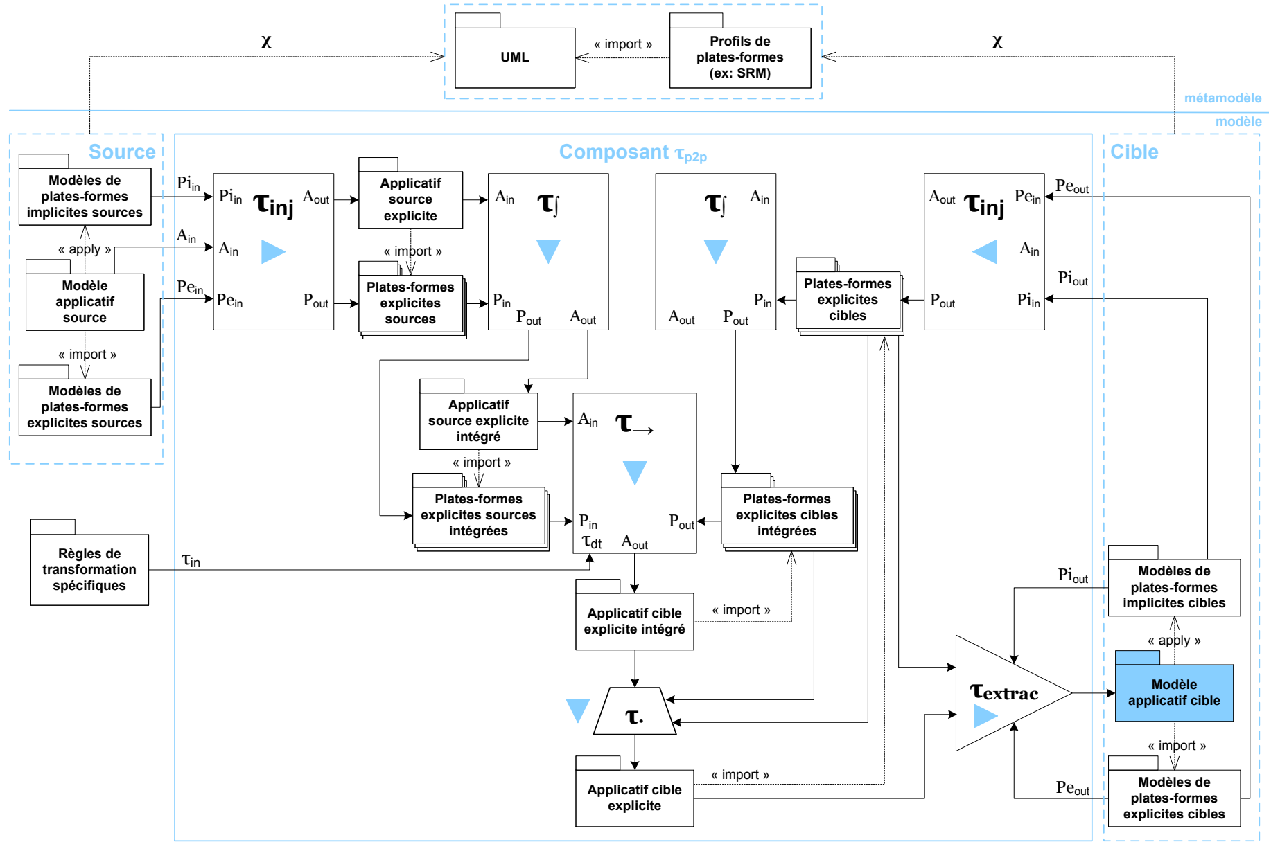
FIG. 7.7 – Synoptique du composant de transformation \tau_{p2p}
