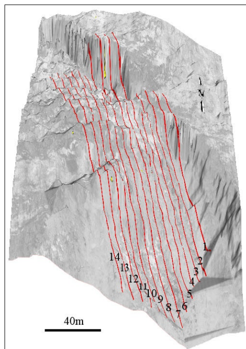
Figure III.44 : Localisation des coupes dans les acquisitions scanner-laser sur les Ruines de Séchilienne. (vue en relief avec ortho-image de 2003 drappée sur MNT scanner-laser de juin 2007)
