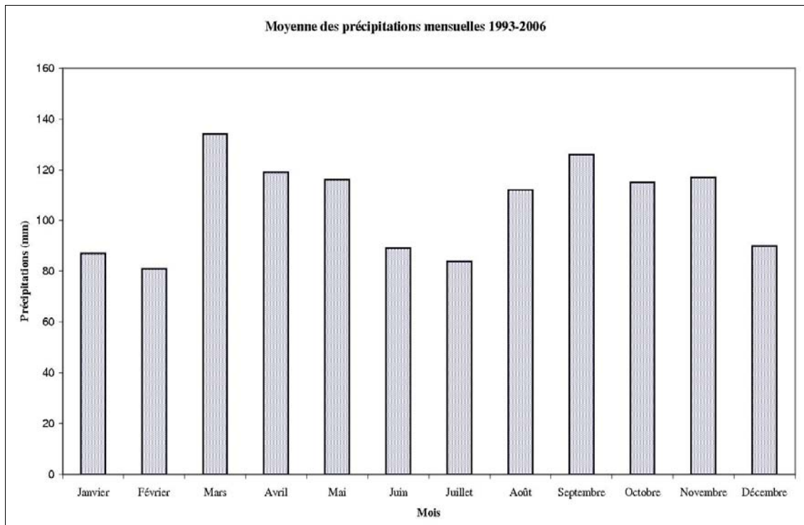
Figure III.12 : Moyenne mensuelle des précipitations de 1993 à 2006 sur la station du Mont-Sec. La moyenne mensuelle des précipitations est de 106 mm/mois, alors que la moyenne annuelle est de 1281 mm/an.
