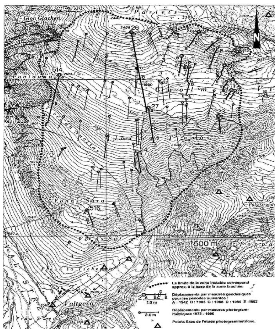
Figure IV.34 : Déplacements planimétriques obtenus par photogrammétrie (1973-1990).
