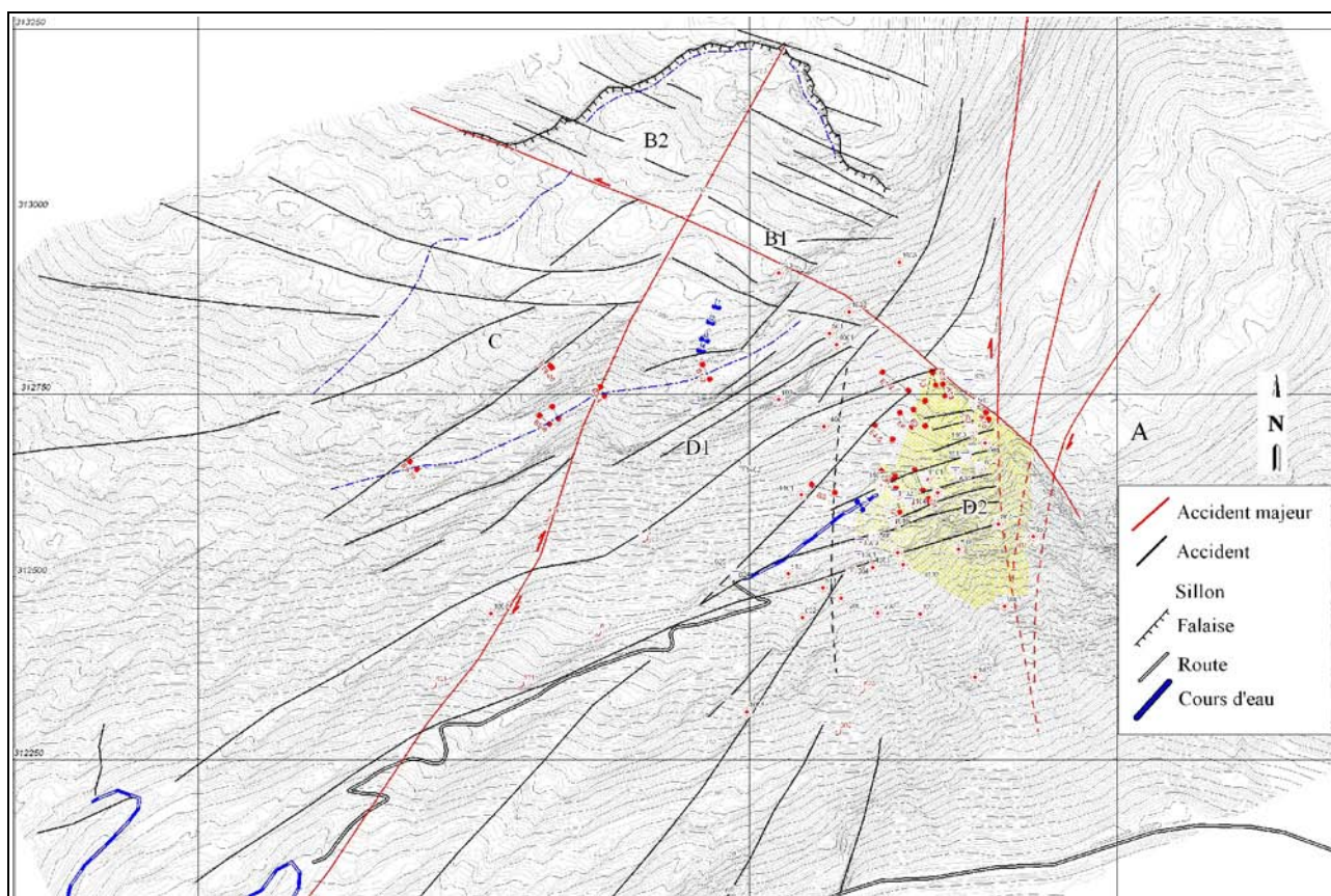
Figure III.7 : Schéma structural du versant sud du Mont-Sec. (modifié d'après l'esquisse de Pothérat (1995) sur images aériennes spécifiques de 1995)
