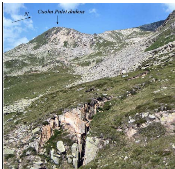
Figure IV.15 : Ouvertures en traction au nord de la grande ouverture (T1).
