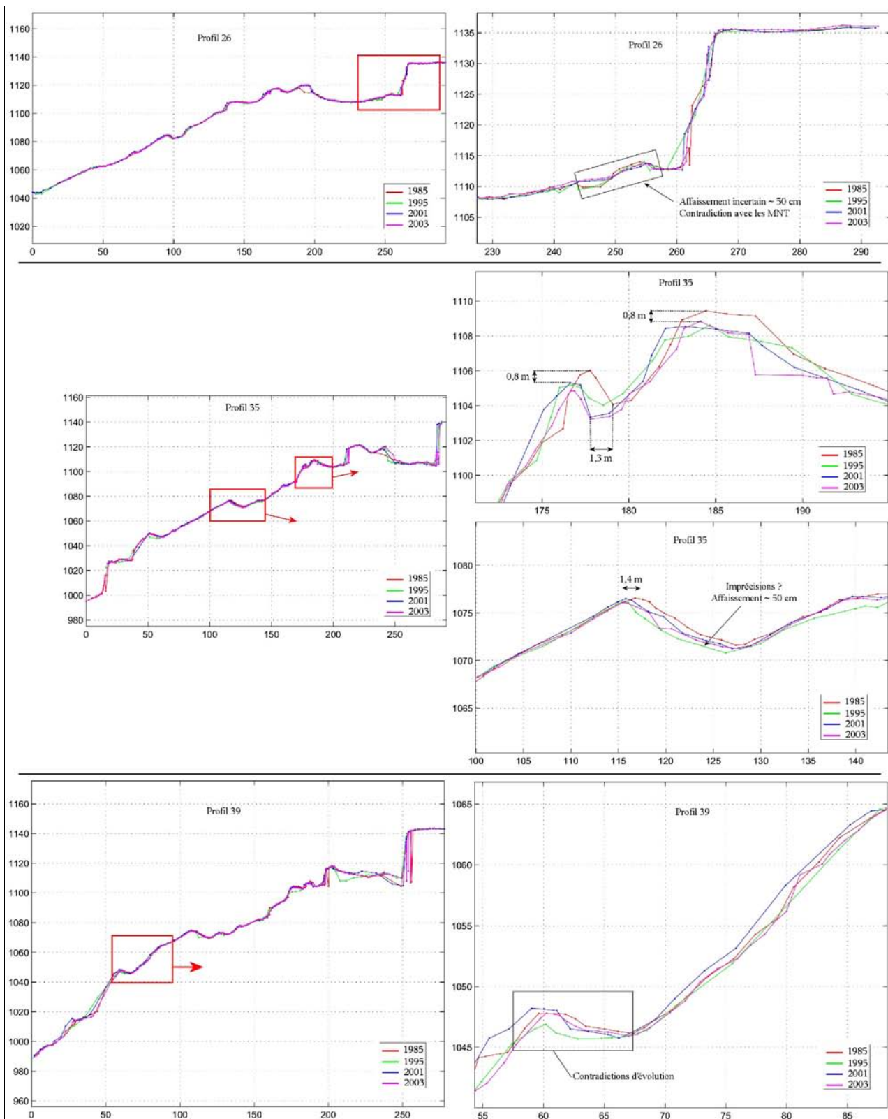
Figure III.34 : Profils n°s 26, 35 et 39 dans la zone d'affaissement sommitale dite des "Entonniers".
