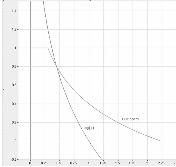
Figure 20 : Comparaison des normes : -\log(x) et notre norme (“our norm”)
