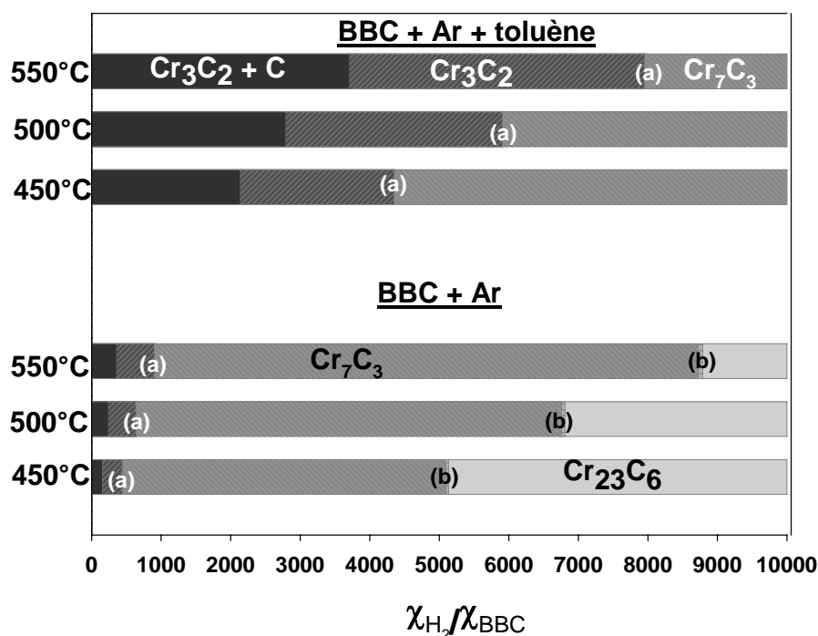
Figure IV.5 : Domaines de stabilité des phases condensées en fonction du rapport molaire hydrogène/BBC sous 1 atm à 450°C-550°C avec ou sans solvant (a) domaine biphasé \text{Cr}_3\text{C}_2 + \text{Cr}_7\text{C}_3 , (b) domaine biphasé \text{Cr}_7\text{C}_3 + \text{Cr}_{23}\text{C}_6
