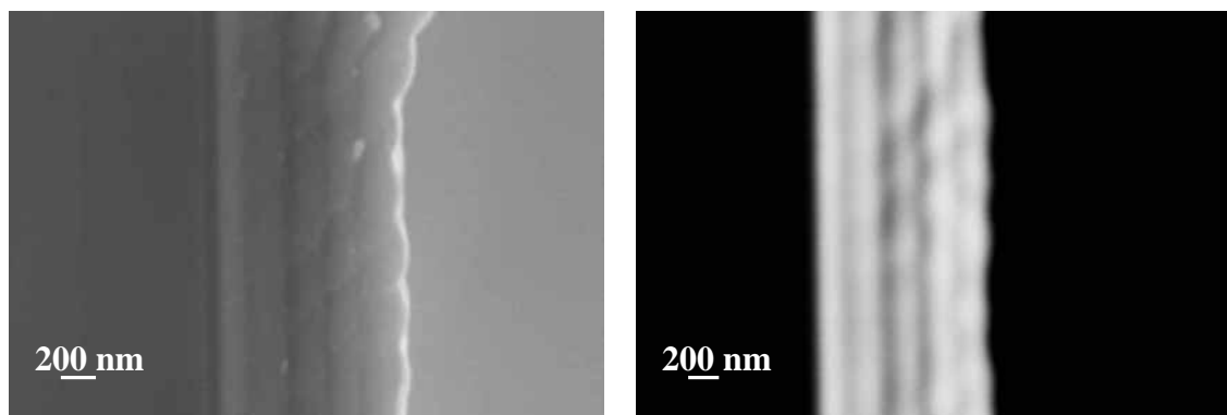
Figure V.18 : Clichés MEB en coupe (électrons secondaires à gauche et électrons rétrodiffusés à droite) d'un revêtement multicouche CrN/Cr-C avec \lambda=200 nm sur substrat SiN/Si.
