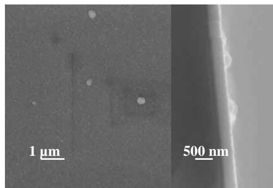
Figure III.16 : Morphologie de surface sur acier SS304L (à gauche) et section en coupe sur substrat Si (à droite) d'un revêtement \text{CrC}_x\text{O}_y obtenu sous atmosphère \text{N}_2 à partir d'une solution de \text{Cr}(\text{CO})_6 dans le toluène à 350^\circ\text{C} , \chi_P = 47 ppm (essai 15)
