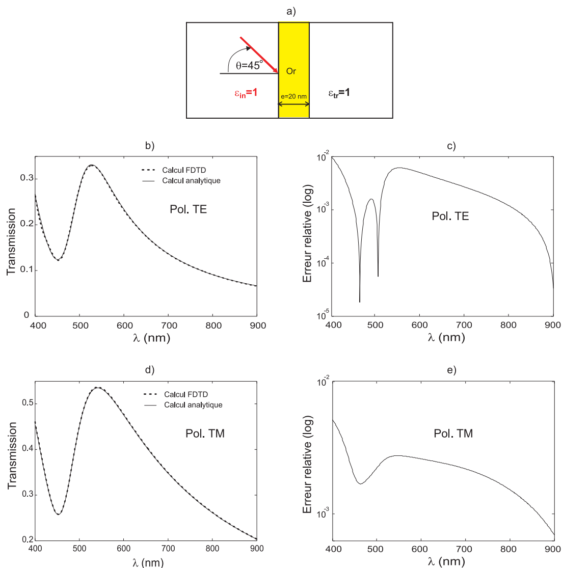
FIG. 3.14 – Transmission à travers une couche plane d’or; épaisseur=20 nm, \theta = 45^\circ and \phi = 0^\circ . b) et c) polarisation TE; d) et e) polarisation TM. Les résultats FDTD sont comparés à ceux théorique en b) et d). Les erreurs relatives sont présentées en c) et e).
