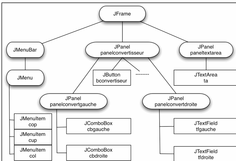
Figure 47 : Hiérarchie des composants de l'interface du convertisseur initial
