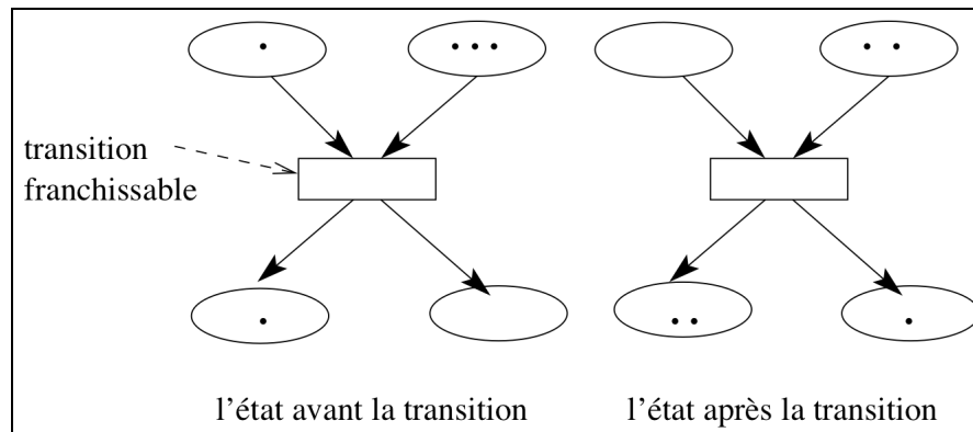
Figure 53 : Exemple de réseau de Petri
