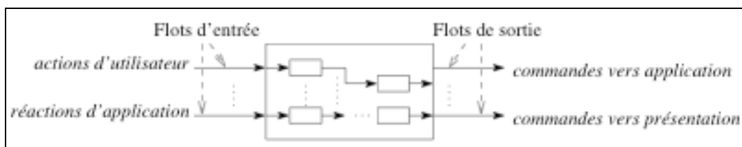
Figure 52 : Interacteur à flux de données
