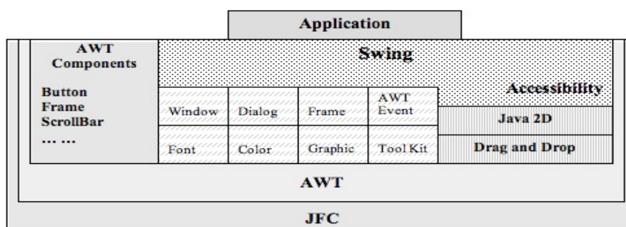
Figure 38 : Architecture de Java avec AWT et Swing (extrait de http://java.sun.com )
