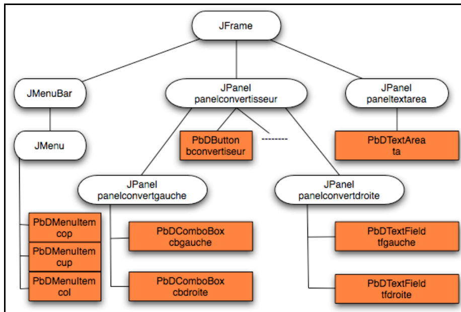
Figure 48 : Hiérarchie des composants de l'interface du convertisseur avec prise en compte de la PsE
