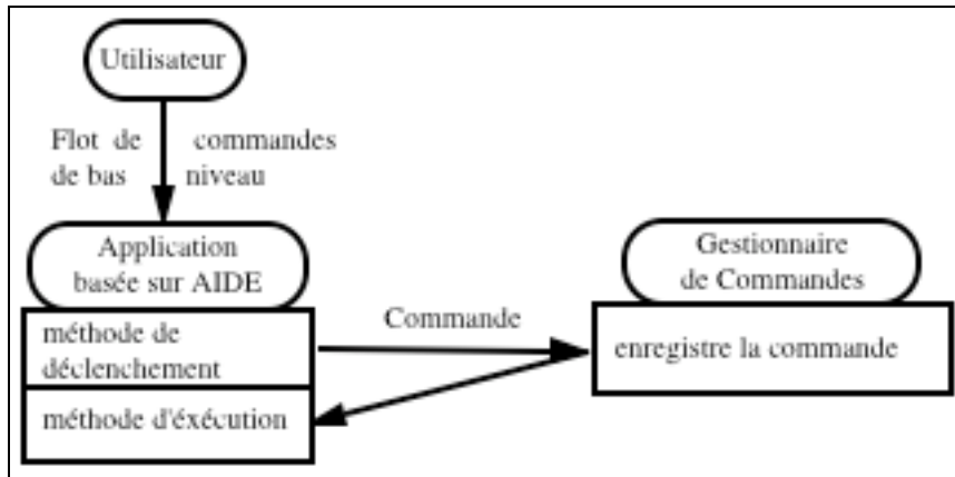
Figure 27 : Dialogue entre l'Application et AIDE lors de l'exécution d'une commande
