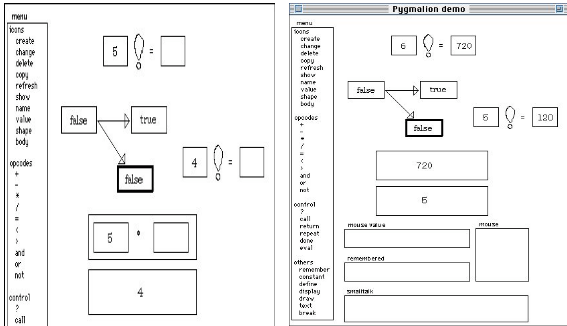
Figure 3 : Réalisation de la fonction « factorielle » à l'aide de Pygmalion
