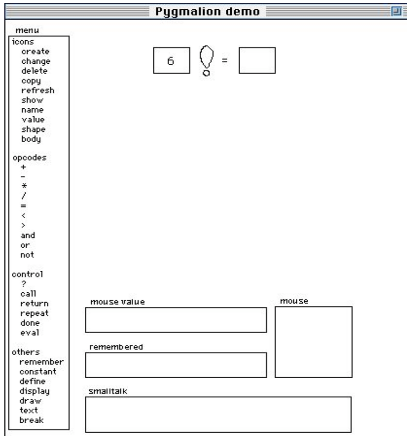
Figure 2 : Environnement Pygmalion
