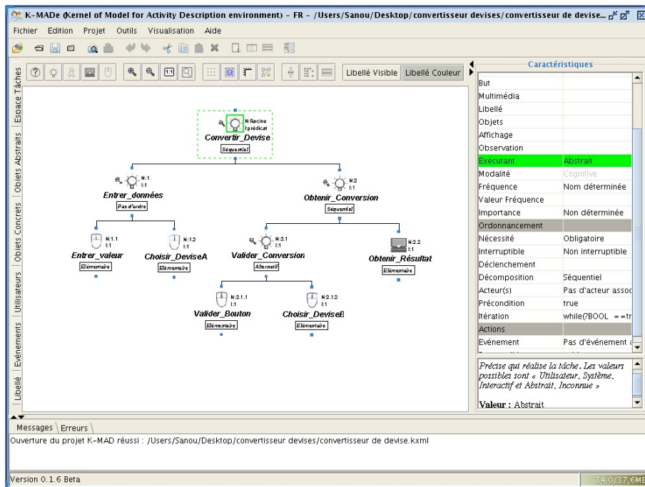
Figure 55 : Environnement K-MADE
