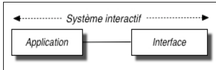
Figure 12 : Système interactif
