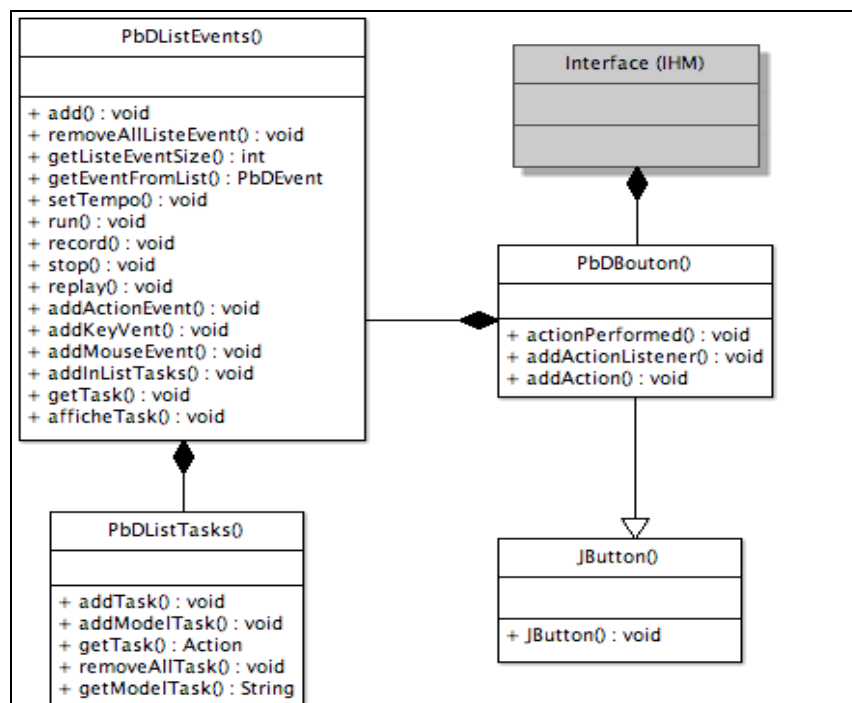
Figure 57 : Extrait du diagramme UML de PbDToolkit
