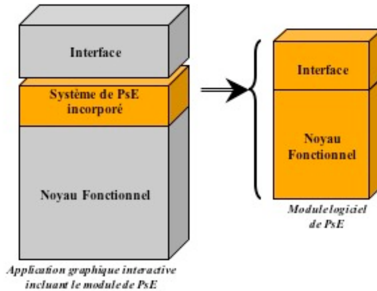
Figure 1 : Vision de l'architecture d'implémentation du module logiciel de la PsE
