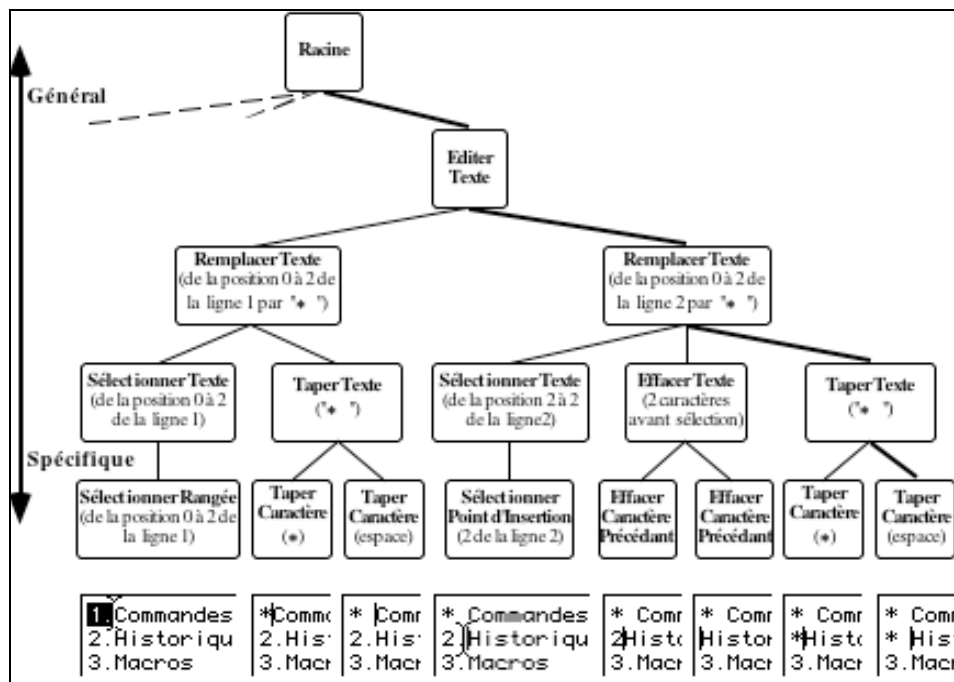
Figure 26 : Arbre de commandes pour une tâche de « Remplacer les numéros par des astérisques » dans une liste
