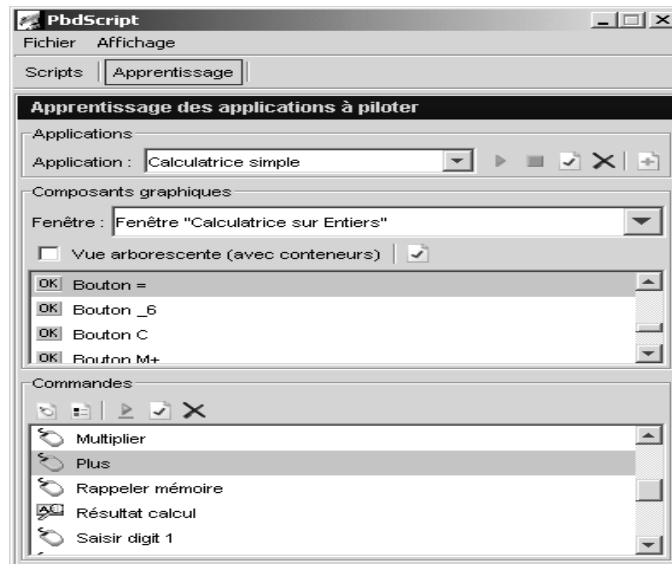
Figure 21 : Apprentissage des applications cibles dans PbdScript
