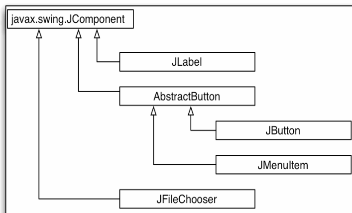
Figure 43 : Hiérarchie de classes de composants
