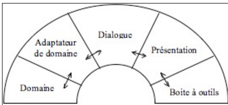
Figure 32 : Le modèle ARCH
