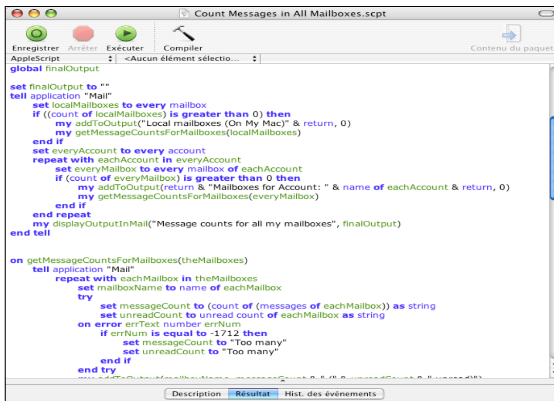
Figure 15 : Éditeur de Script sous Mac OS X
