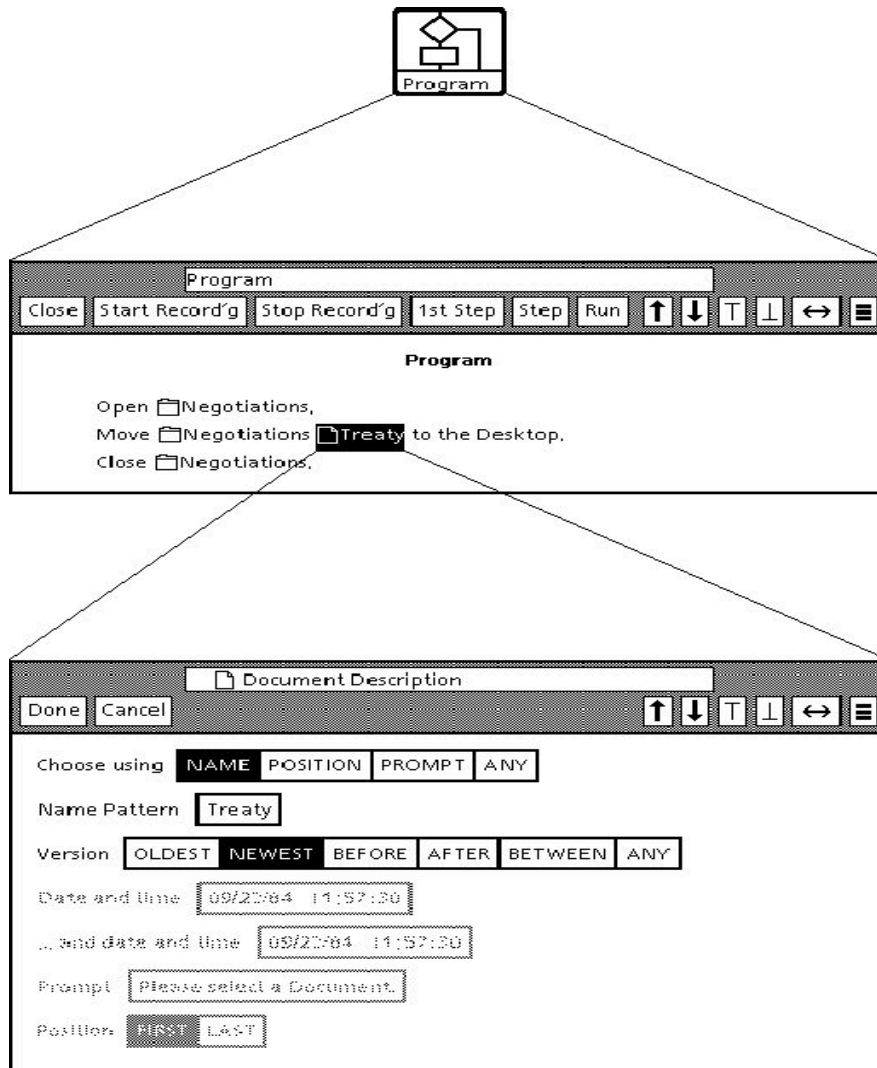
Figure 18 : SmallStar : une macro qui place la dernière version du fichier "Treaty" sur le bureau
