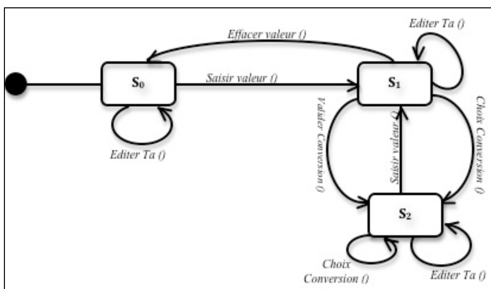
Figure 45 : Dynamique de l'application du Convertisseur
