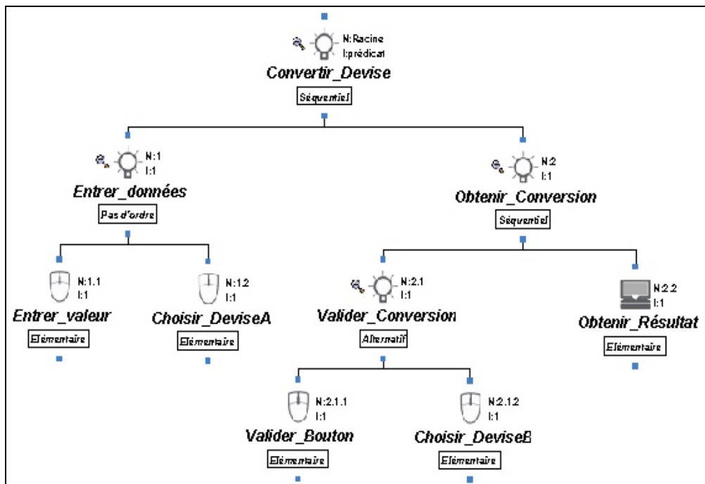
Figure 54 : Modèle de tâches K-MADe du Convertisseur de devise.
