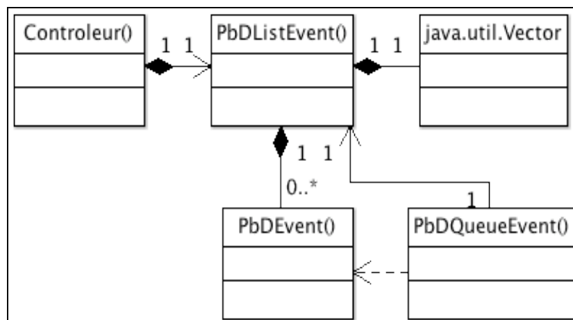
Figure 40 : Objets de coopération avec la classe PbDListEvent
