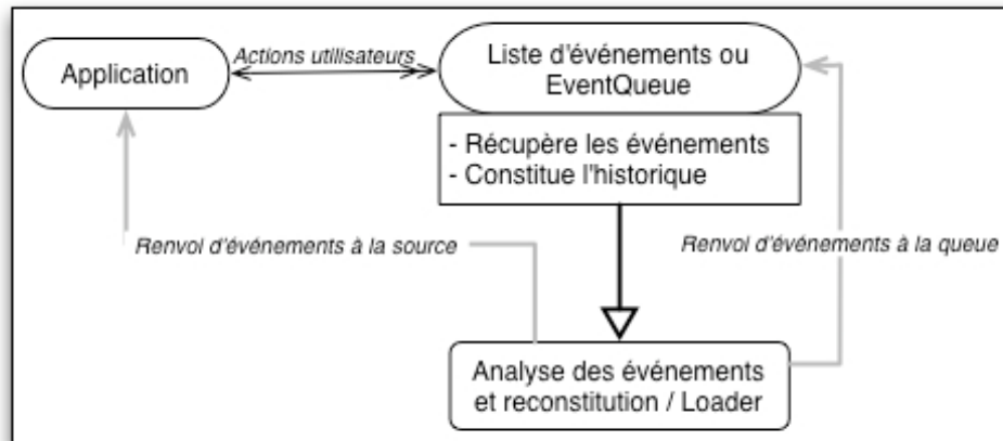
Figure 37 : Schéma d'architecture de coopération d'application incluant la PsE
