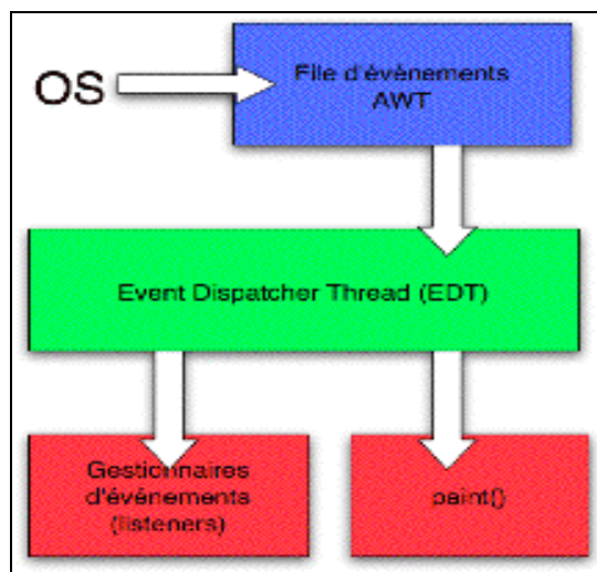
Figure 41 : Transmission des événements en Swing
