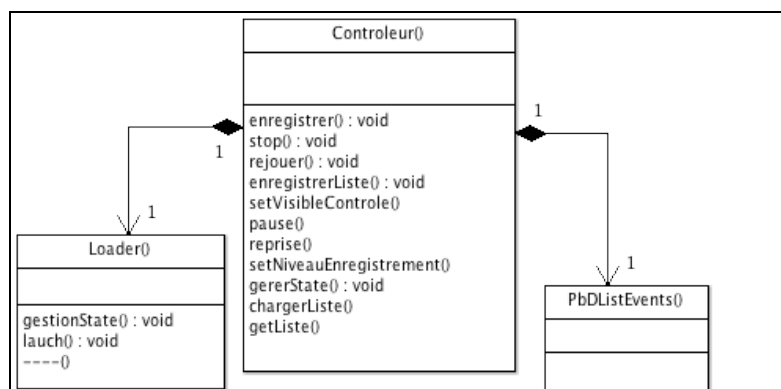
Figure 36 : Représentation UML des classes principales de gestion de PbDToolkit
