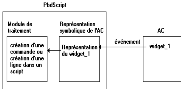
Figure 24 : Gestion d'événements émis par l'application cible (AC)
