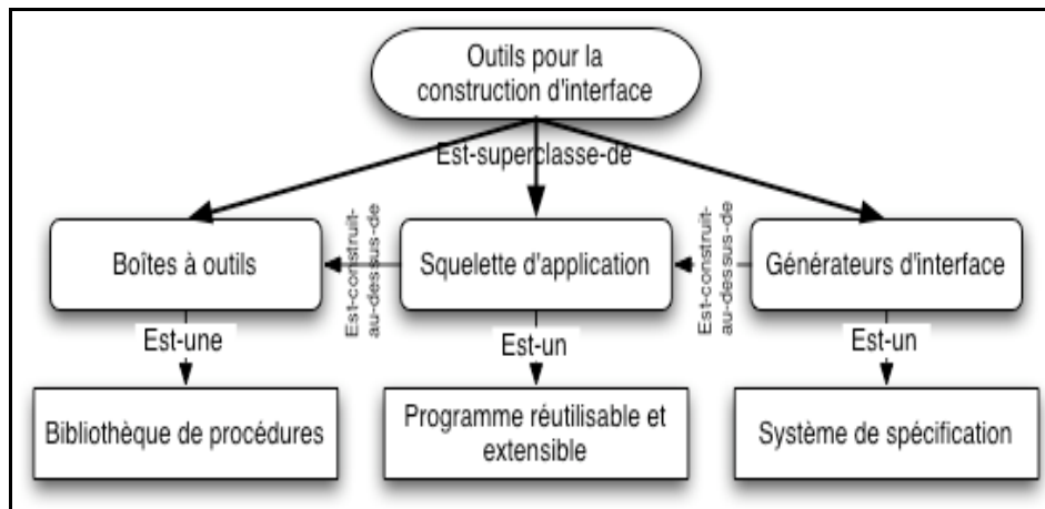
Figure 30 : Classification des outils de construction d'interfaces
