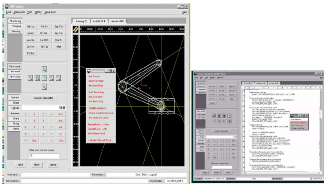
Figure 5: Environnement EBP
