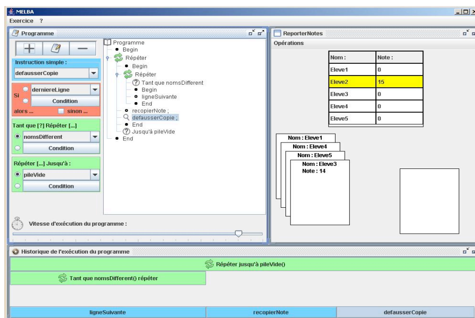
Figure 10 : Environnement MELBA
