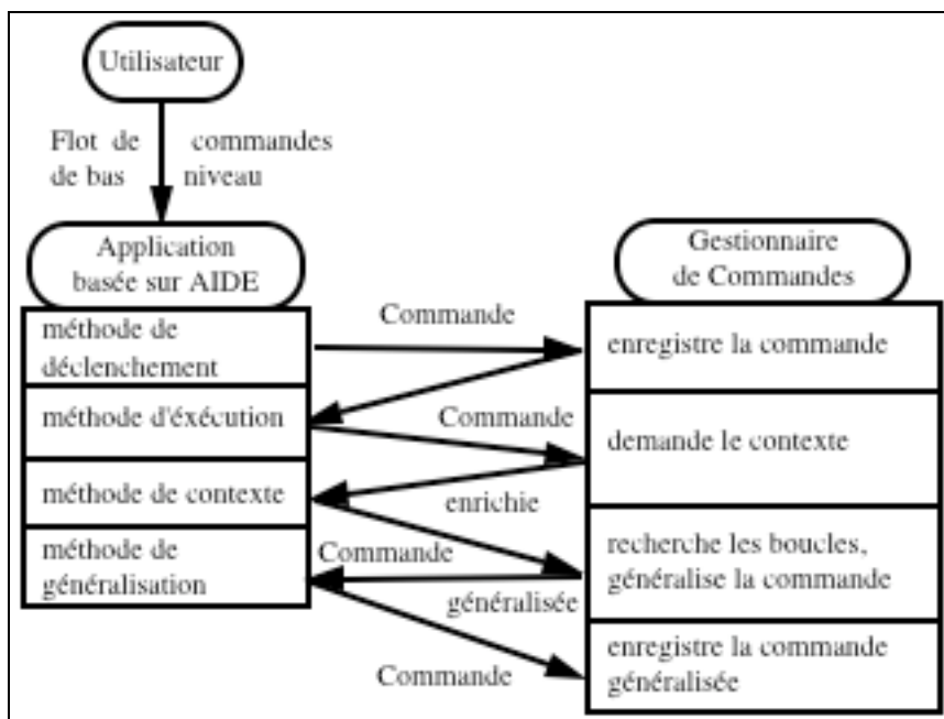
Figure 28 : Dialogue entre l'application et AIDE en mode enregistrement de macros
