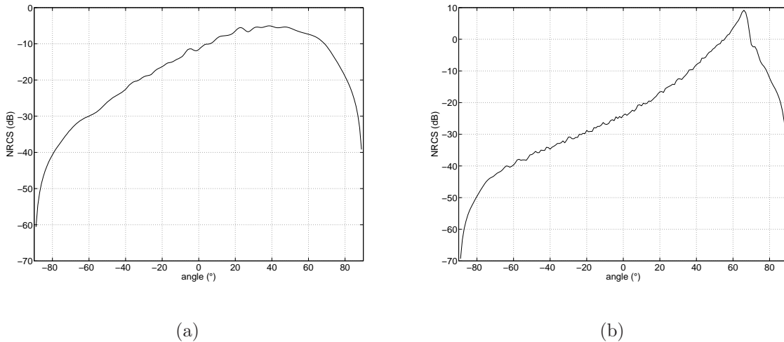
FIG. 2.18 – Module carré de \left(\frac{\partial S(q, q_0)}{\partial q_0}\right)_{q_0=0} : (a) surface gaussienne de hauteur quadratique moyenne de 0.083\lambda et de longueur de corrélation 0.5\lambda , (b) surface en k^{-4} avec une coupure basse fréquence de K/15 et une coupure haute fréquence de 4K .
