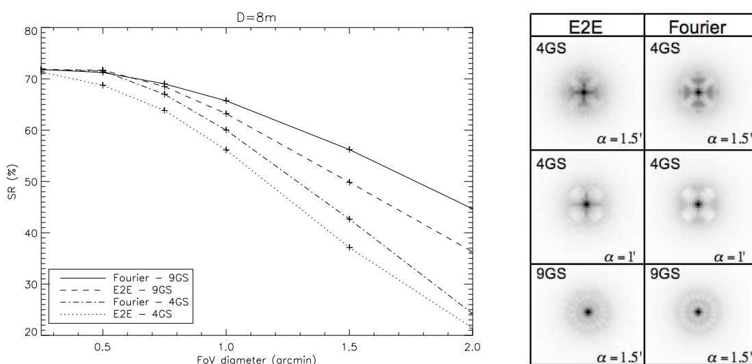
FIG. 7.13 – A gauche : Comparaison Fourier E2E pour un profil à 10 couches corrigé par 3 DMs. Le diamètre du télescope est de 8m. Deux constellations sont étudiées : 4 et 9 étoiles en cercle. A droite : Comparaison des PSFs.
