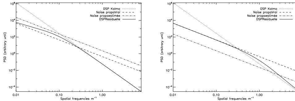
FIG. 6.10 – DSP turbulente, DSP de propagation du bruit et DSP résiduelle pour un reconstructeur MMSE avec une erreur sur le SNR. A gauche le bruit est sur-estimé d'un facteur 10. A droite, le bruit est sous-estimé d'un facteur 10.
