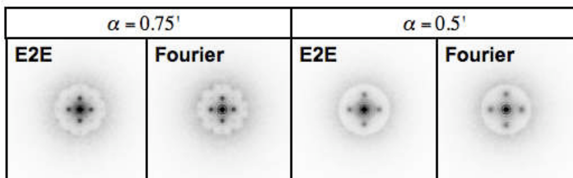
FIG. 7.12 – Comparaison des PSFs obtenues avec les codes Fourier et E2E dans des cas de bons recouvrements. Le télescope est un 8m avec un constellation à 4 étoiles. \alpha représente le diamètre de la constellation.
