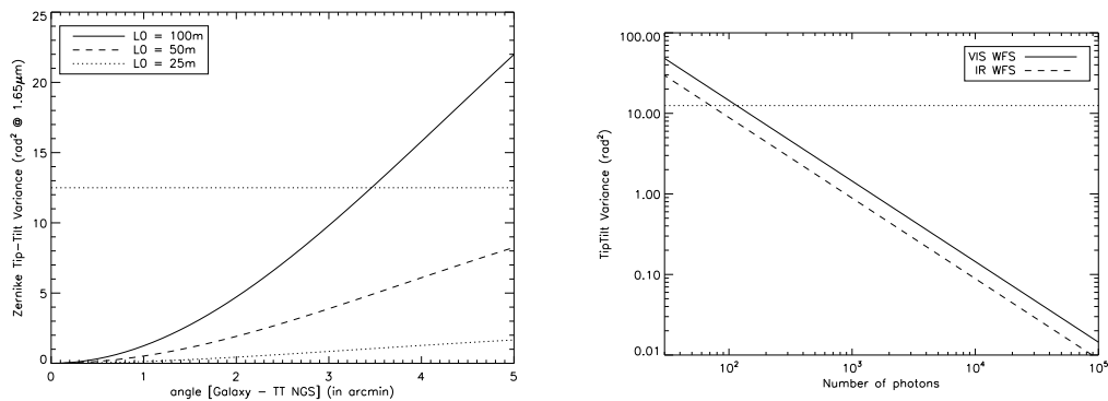
FIG. 8.13 – Variations résiduelles. A gauche : erreur d'anisoplanétisme pour trois valeurs de L_0 . A droite : variance de bruit de photons pour un analyseur dans le visible et dans le proche infra-rouge.
