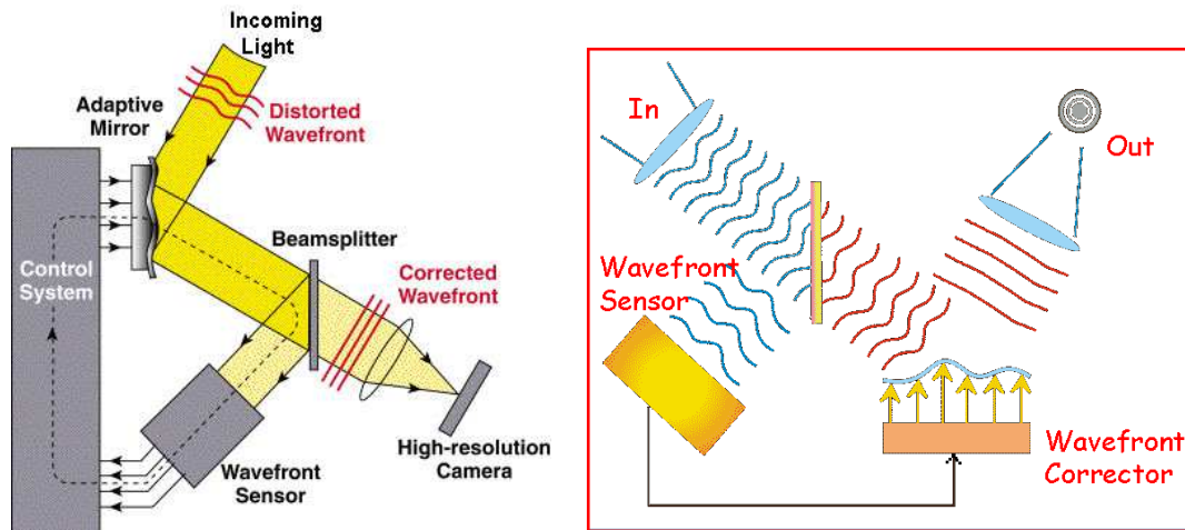
FIG. 6.1 – Schéma de principe d'un système d'optique adaptative. A gauche dans une configuration boucle fermée et à droite dans une configuration boucle ouverte.
