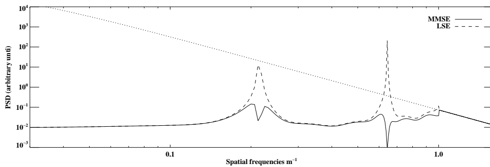
FIG. 7.8 – Coupe de la DSP résiduelle d'aliasing dans un cas MMSE et un cas LSE. r_0 = 0.11\text{m} à 0.5\mu\text{m} . La fréquence de coupure est de 1\text{m}^{-1} .
