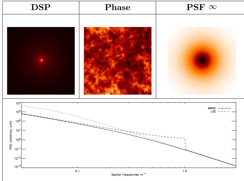
FIG. 6.8 – Erreur de reconstruction et propagation du bruit d’analyse. En haut et de gauche à droite : DSP, Phase instantanée et PSF pose infinie pour le reconstructeur MMSE. En bas, coupe dans la DSP selon l’axe des x . r_0 = 0.44\text{m} à 1.65\mu\text{m} . La fréquence de coupure est de 1\text{m}^{-1} . Le bruit d’analyse est de 50\text{rd}^2 dans cet exemple. La DSP est donnée en échelle Log, la phase en échelle linéaire et la PSF en échelle Log inversée. Les seuils sont ajustés individuellement.
