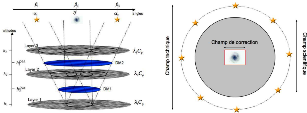
FIG. 7.4 – Illustration de la géométrie et des notations. A gauche : synthèse de notations d'angles. A gauche : définitions des angles utilisés. A droite : définition du champ technique, champ scientifique et champ de correction. Le champ technique (en pointillé) est le champ dans lequel on peut aller chercher les étoiles guides. Le champ scientifique (surface grise) est le champ dans lequel on peut aller chercher les objets d'intérêt. Le champ de correction (carré rouge) correspond aux zones où la correction est optimisée. L'exemple présenté ici correspond à un cas de LTAO.
