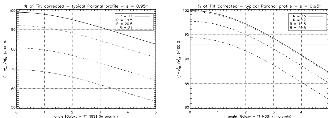
FIG. 8.14 – Pourcentage de correction de la variance atmosphérique de Tip/Tilt en fonction de la magnitude et de la distance angulaire de l'étoile naturelle. A gauche : pour un L_0 de 50m. A droite : pour un L_0 de 100m.
