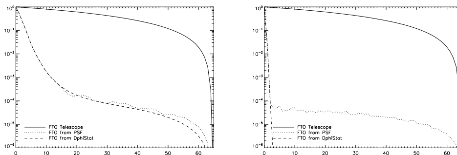
FIG. 6.18 – Comparaison des FTO “vraies” (notée “FTO from PSF”) et “stationnarisées” (notée “FTO from DphiStat”) dans un cas purement turbulent. A gauche : r_0=1.5 . A droite : r_0=0.44 . La ligne continue symbolise la FTO théorique du télescope.
