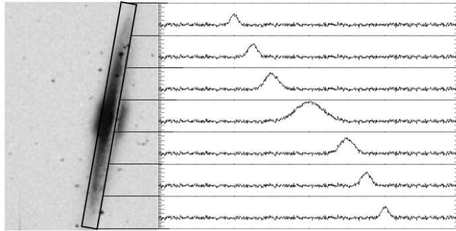
FIG. 2.9 – Illustration de la mesure d'une courbe de rotation pour une galaxie spirale. Pour chaque point résolu le long de la fente, on mesure le décalage Doppler d'une raie en émission dans cet exemple. La dispersion est plus forte au centre où la contribution du bulbe est plus importante.
