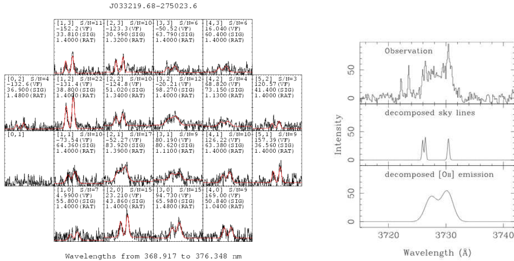
FIG. 3.2 – Exemple d’ajustement simultané des raies du ciel et du doublet [OII]. A gauche, on montre les 20 spectres individuels avec le meilleur ajustement superposé en rouge. A droite, on montre la procédure d’ajustement avec l’observation, les raies du ciel et l’émission [OII].
