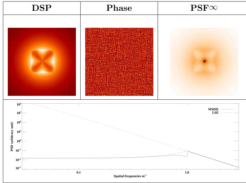
FIG. 6.12 – Erreur d’aliasing. En haut et de gauche à droite : DSP, Phase instantanée et PSF pose infinie pour le reconstructeur LSE. En bas, coupe dans la DSP selon l’axe des x . r_0 = 0.44\text{m} à 1.65\mu\text{m} . La fréquence de coupure est de 1\text{m}^{-1} . La DSP est donnée en échelle Log, la phase en échelle linéaire et la PSF en échelle Log inversée. Les seuils sont ajustés individuellement.
