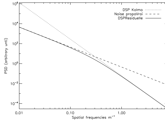
FIG. 6.9 – DSP turbulente, DSP de propagation du bruit et DSP résiduelle pour un reconstituteur MMSE sans erreur sur le SNR. On s'intéresse ici à la zone de transition entre les fréquences dont le SNR est \gg 1 ( f < 0.1m^{-1} ) et les fréquences pour lesquelles le SNR devient \ll 1 ( f > 1m^{-1} ).
