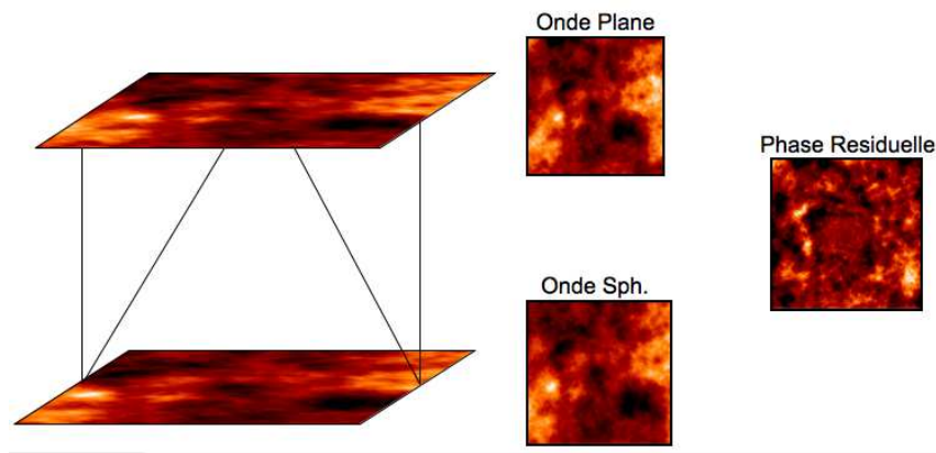
FIG. 6.17 – Principe de simulation de l'effet de cône sur la phase résiduelle. On dilate les phases en altitudes d'un coefficient proportionnel à leur altitude et à l'altitude de la source laser. La phase résiduelle est formée par la différence entre l'onde sphérique et l'onde plane.
