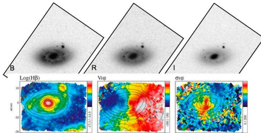
FIG. 2.11 – Principales techniques de spectroscopie intégrale de champ. D'après Jeremy Allington-Smith.
