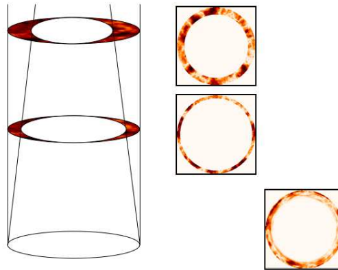
FIG. 7.14 – Illustration des zones non-vues de turbulence dans une géométrie onde plane / onde sphérique. La phase résiduelle est la somme des anneaux de turbulences non-vues.
