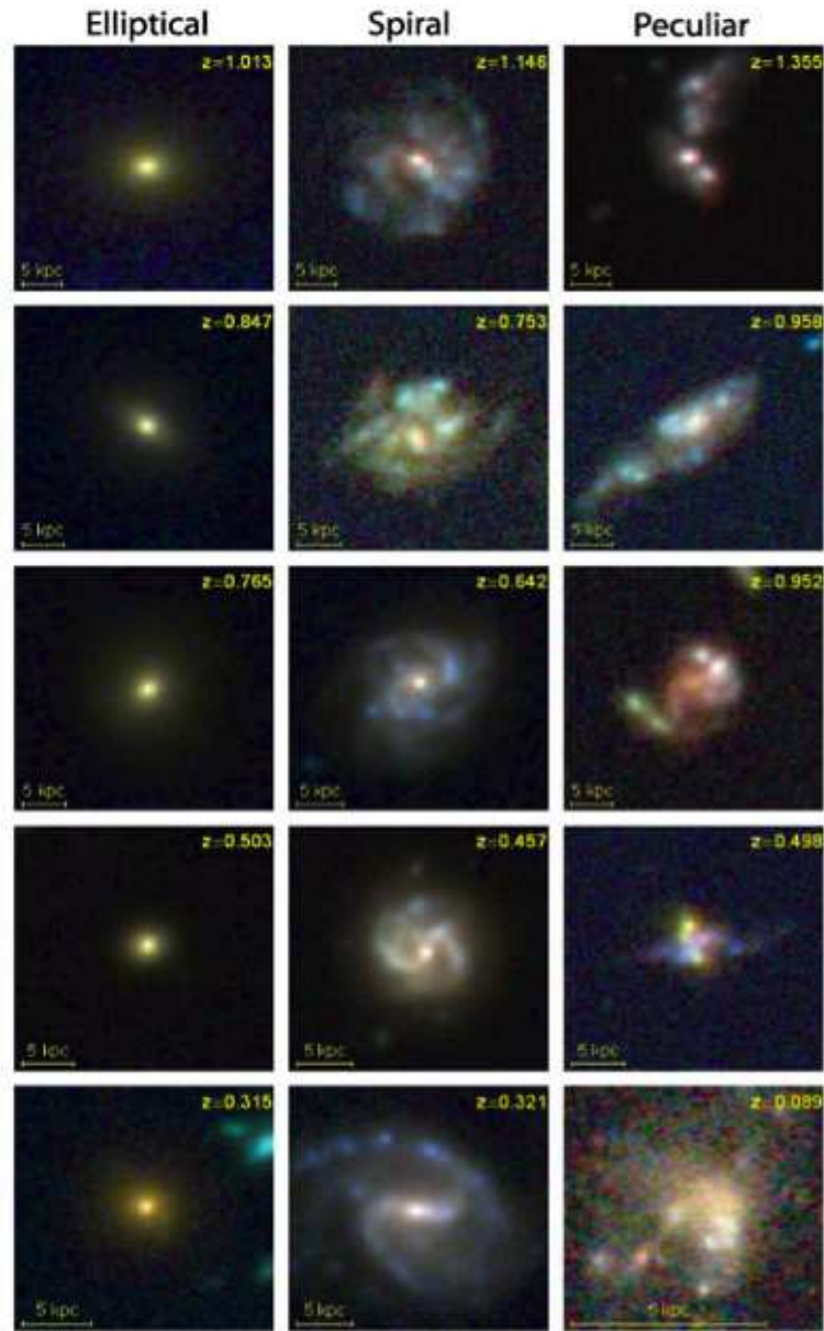
FIG. 1.2 – Evolution des galaxies de différents types morphologiques. Les galaxies sont classées par z décroissant. Tiré de Abraham et van den Bergh (2001).
