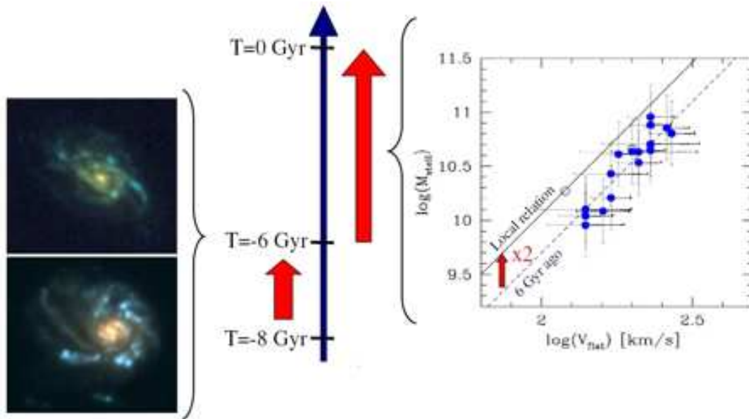
FIG. 3.6 – Histoire schématique de l'évolution des galaxies spirales.
