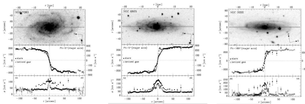
FIG. 2.10 – Courbe de rotations de 3 galaxies locales avec leur dispersion de vitesse, pour les étoiles et le gaz. D’après Pizzella et al. (2004)
