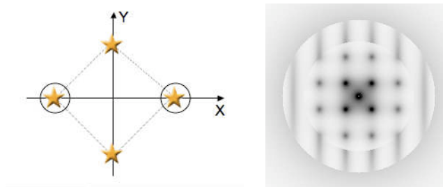
FIG. 7.7 – Multipitch d'analyse. A gauche : Constellation "4 GS". Les étoiles encadrées sont analysées par des sous-pupilles de taille d=0.4m ( f_c = 1.25m^{-1} ), les deux autres étoiles sont analysées par des sous-pupilles de taille d=0.55m ( f_c = 0.9m^{-1} ). A droite : DSP correspondante.
