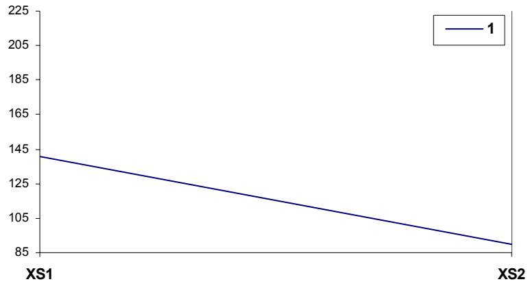
Signature multibande des centres de classe : estrans rocheux faiblement immergés
