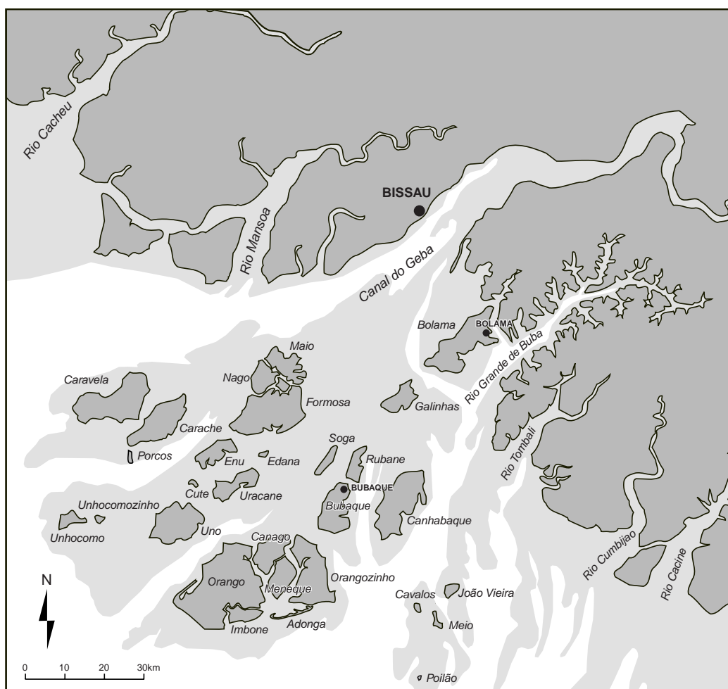
ill. n°2 : L'archipel des Bijagos, présentation générale
