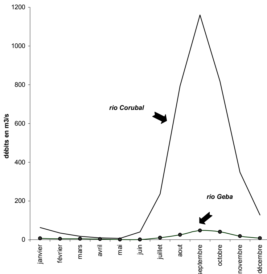
ill. n°47 : Débits moyens calculés entre 1977 et 1994 pour le rio Corubal à Saltinho et entre 1978 et 1993 pour le rio Geba à Sonaco amont.
