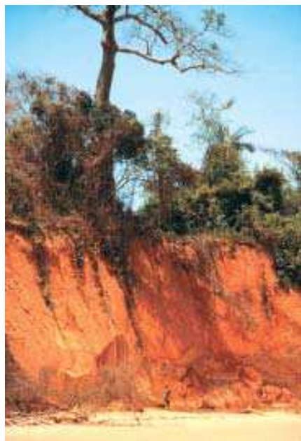
ill. n°72 : Types et profils des falaises de l'archipel des Bijagos
