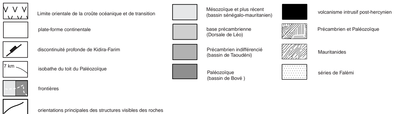
ill. n°35 : Juxtaposition des principaux traits géologiques et structuraux de l'Afrique de l'Ouest au voisinage de la Guinée Bissau
