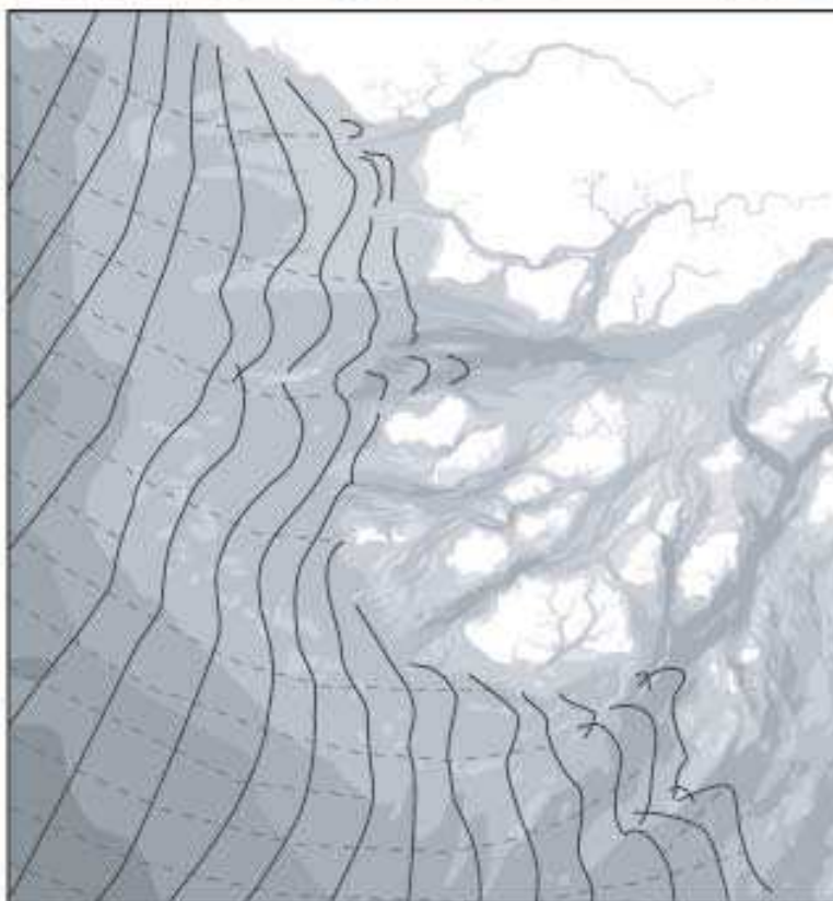
ill. n°59 : Propagation de la houle à la côte selon deux directions d'origine (d'après F. Cuq, 1979)
