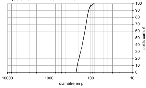
jo95be03 - mz : 162 - si : 0.89
