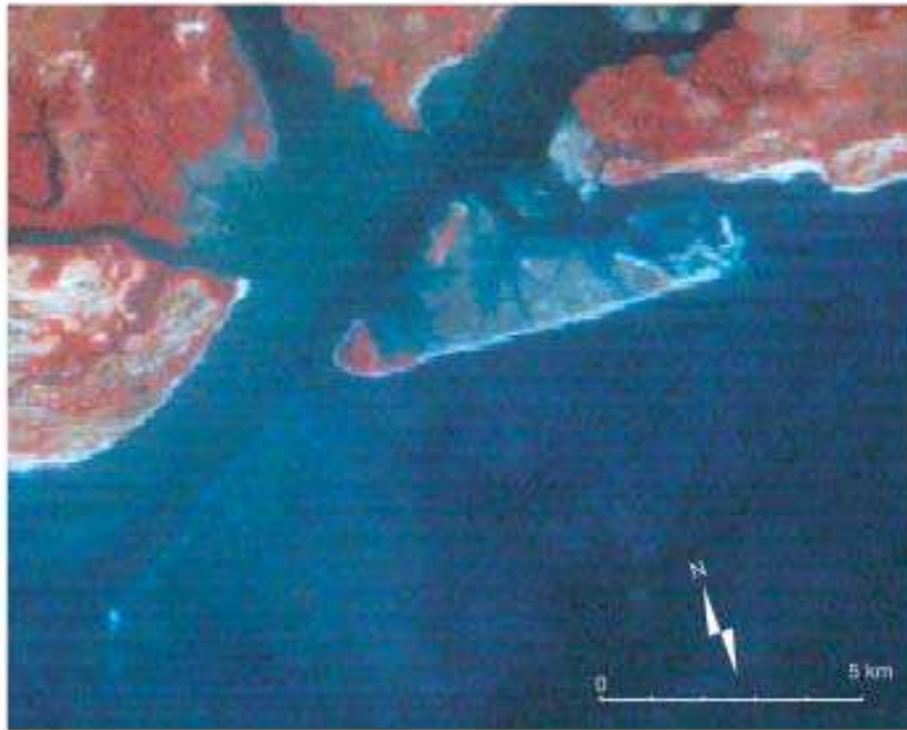
Extrait d'une composition colorée Landsat2 - bandes 4 5 7 - 10/03/1973
