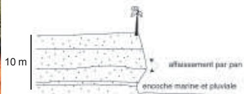
c) falaise vive de l'île de Meio limono-argileuse
