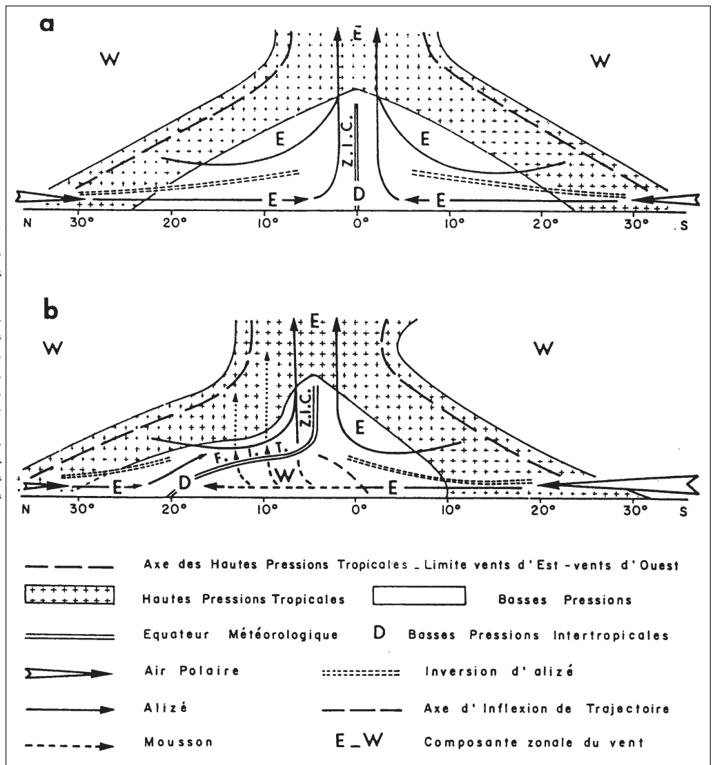
ill. n°40 : Coupe de la structure verticale moyenne de la troposphère tropicale (extrait de M. Leroux, 1983)
