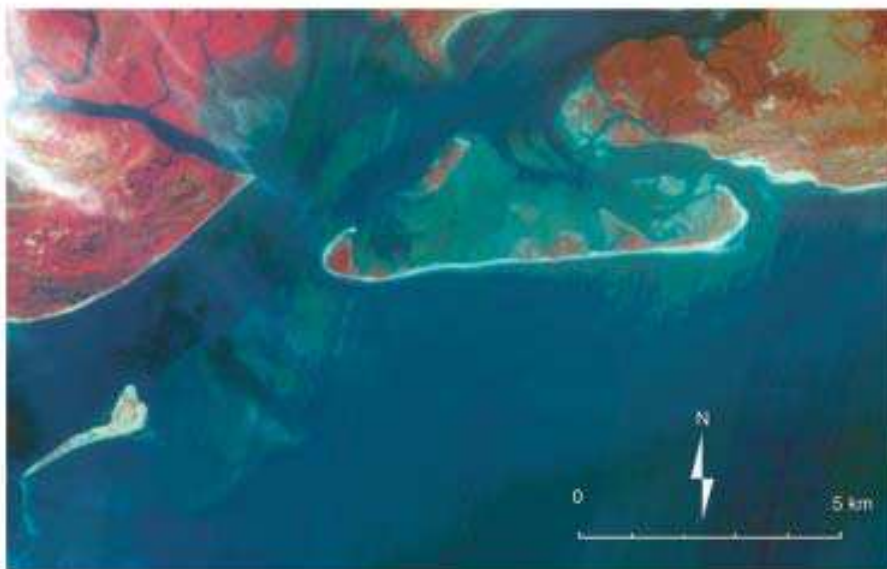
Extrait d'une composition colorée SPOT1 - bandes 1 2 3 - 10/02/1990
