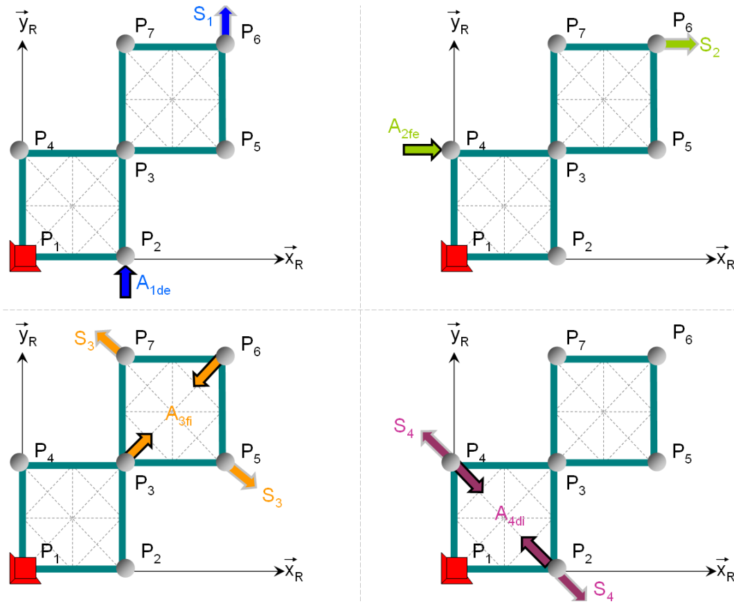
FIGURE 2.9 – Cas test du double carré à 4 DDLS. L'actionneur A_{1de} impose un déplacement vertical au point P_2 (DDL n°1), l'actionneur A_{2fe} applique une résultante mécanique horizontale au point P_4 (DDL n°2), l'actionneur A_{3fi} exerce une résultante mécanique entre les points P_3 et P_6 (DDL n°3), et l'actionneur A_{4di} impose un déplacement entre les points P_2 et P_4 (DDL n°4).
