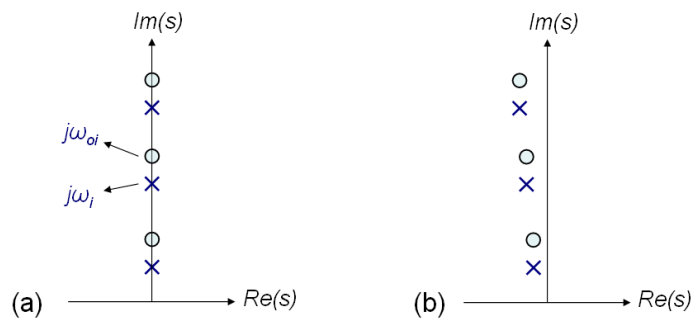
FIGURE 4.10 – Lieux des pôles ( \times ) et des zéros ( \circ ) dans le plan complexe d’un système à alternance pôles/zéros : (a) Cas non-amorti. (b) Cas légèrement amorti. (Seule la partie supérieure du plan complexe est représentée, la figure étant symétrique par rapport à l’axe réel.)
