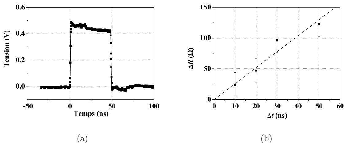
Fig. 6.7 : (a) Tension mesurée aux bornes d'une résistance de 50\ \Omega connectée en série avec une nano-piste de résistance R \approx 0,9\ \text{k}\Omega , pendant l'application d'une impulsion d'amplitude U \approx 9\ \text{V} et de durée 50\ \text{ns} aux bornes de la piste. (b) Augmentation de la résistance de la nano-piste, déduite de traces similaires à (a), en fonction de la durée \Delta t de l'impulsion électrique appliquée, d'amplitude U \approx 9\ \text{V} . La ligne pointillée est une droite d'ajustement de pente 2,6\ \Omega.\text{ns}^{-1} .
