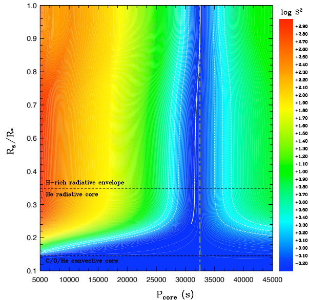
FIG. 4.3: Profil de rotation de l'étoile sdB pulsante Feige 48 (ligne blanche), représenté en termes du logarithme de la fonction de mérite S^2 (échelle de droite), dont les limites 1\text{-}\sigma , 2\text{-}\sigma et 3\text{-}\sigma de la solution optimale sont indiquées par les contours en pointillés. Les paramètres structuraux sont fixés à leur valeur optimale. La ligne blanche s'écarte peu du trait vertical tiret-pointé correspondant à la période orbitale du système, soit 32\,486 s. Sont également indiquées, en tirets horizontaux, les transitions entre l'enveloppe d'hydrogène et le cœur d'hélium, ainsi qu'entre ce dernier et le cœur convectif riche en carbone et oxygène.
