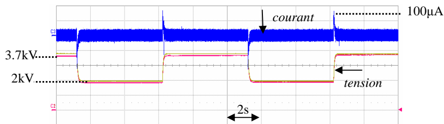
Figure 3.22 : Courbes caractéristiques de tension et courant au sein du générateur en polymère diélectrique
