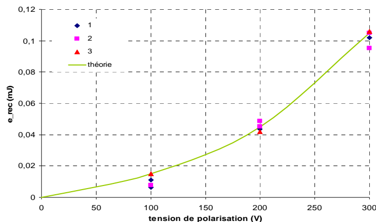
Figure 4.18 : Energie récupérée pour un cycle à tension constante
