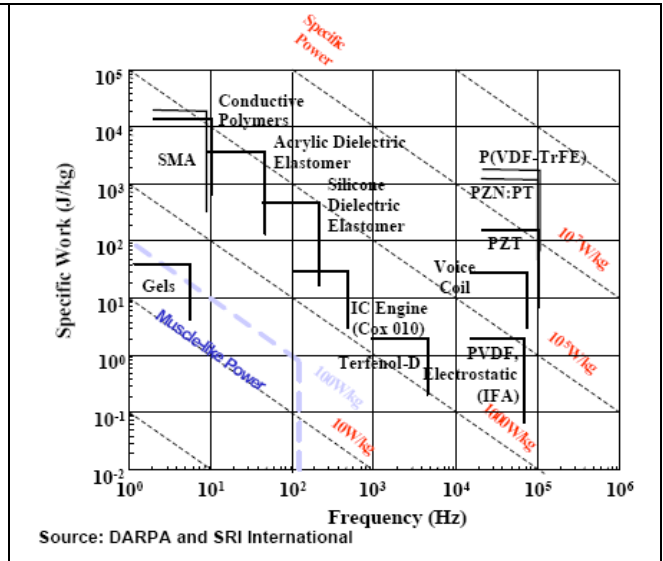
Figure 1.2 : Travail spécifique-fréquence pour différents matériaux électroactifs
