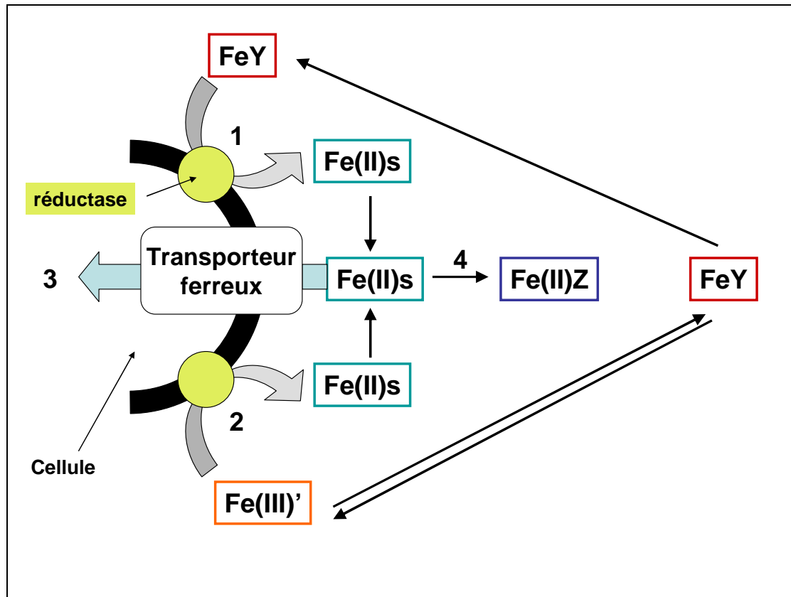
Figure 1 : Présentation du modèle Fe(II)s présenté par Shaked et collaborateurs (Shaked et al., 2005). Le fer ferrique Fe(III) , sous forme complexé Fe(Y) ou sous forme non complexé Fe(III)' , est réduit par des réductases membranaires (1) (2) en fer ferreux Fe(II)s . Ce fer réduit peut ensuite être transporté au sein de la cellule via un transporteur ferreux (3) ou se complexer à un ligand Z dans le milieu (4).
