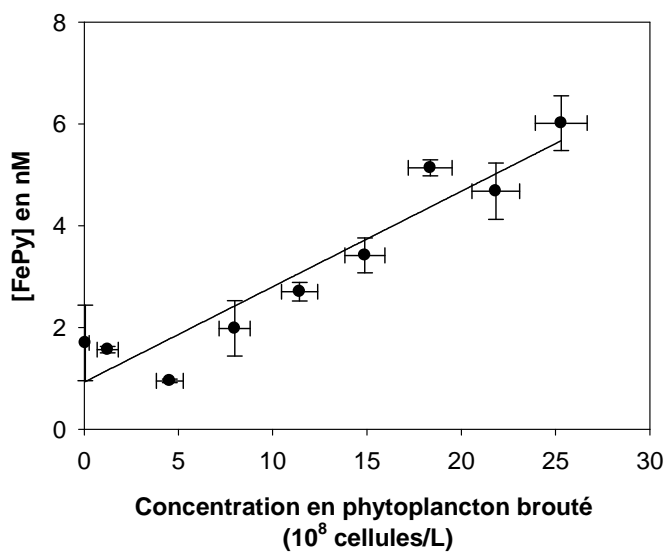
Figure 36 : Relation entre la concentration en FePy dans l'eau de mer et la quantité de cellules phytoplanktoniques broûtées. « k » représente la quantité de FePy libérée par cellule broûtée (en mole FePy.cellule broûtée -1 ).
