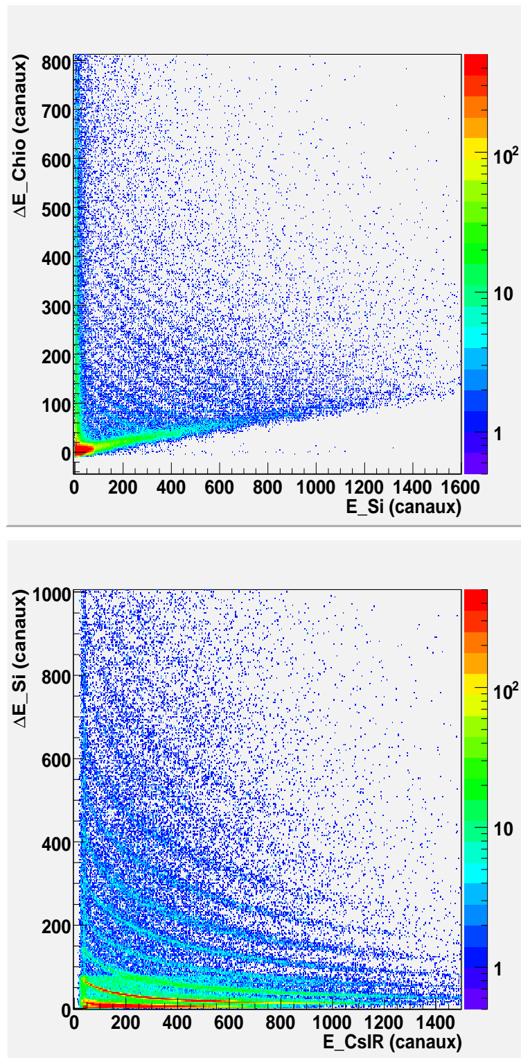
FIG. 1.7 – Matrices d'identification d'un télescope triple. Ces données sont celles du système ^{124}Xe + ^{112}Sn à 32 MeV/u. En haut, la matrice \Delta E_{Chio} - E_{Si} , en bas, la matrice \Delta E_{Si} - E_{CsI}
