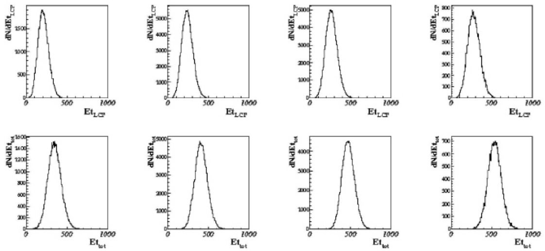
FIG. B.25 – Xe+Sn à 32 MeV/u. La dissipation. Première ligne : L'énergie transverse des particules légères ( Z=1, Z=2 ). Deuxième ligne : L'énergie transverse totale.
