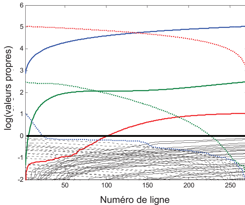
Figure 16 : Graphique contenant les informations du EFA forward et EFA backward de \mathbf{D}_{\text{ex}} , la ligne horizontale en trait noir épais représente le niveau de bruit en dessous duquel on ne considère plus les contributions détectées..
