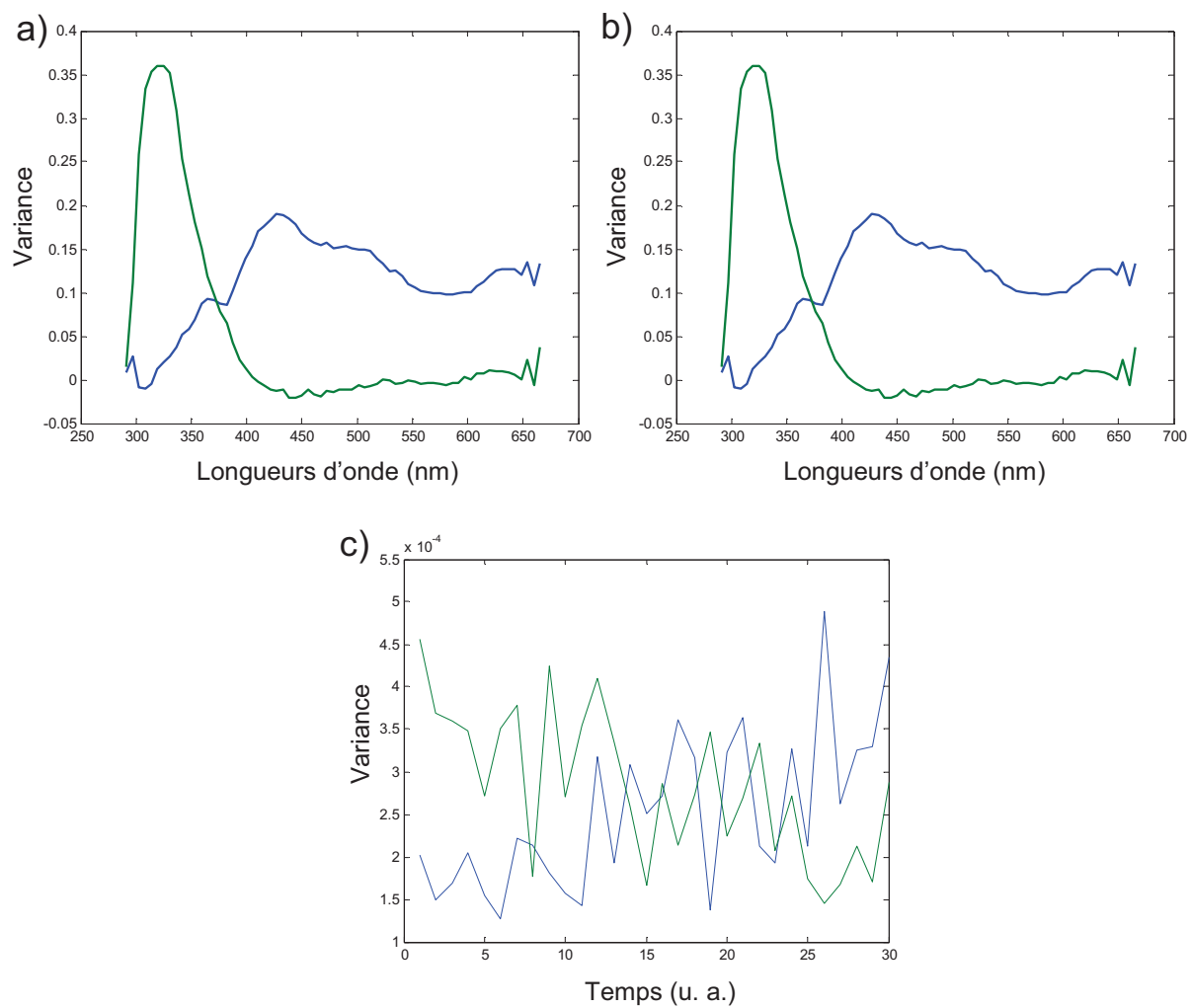
Figure 88 : Loadings de la matrice \Sigma obtenus par PARAFAC a) 1 er mode b) 2 nd mode c) 3 ème mode.
