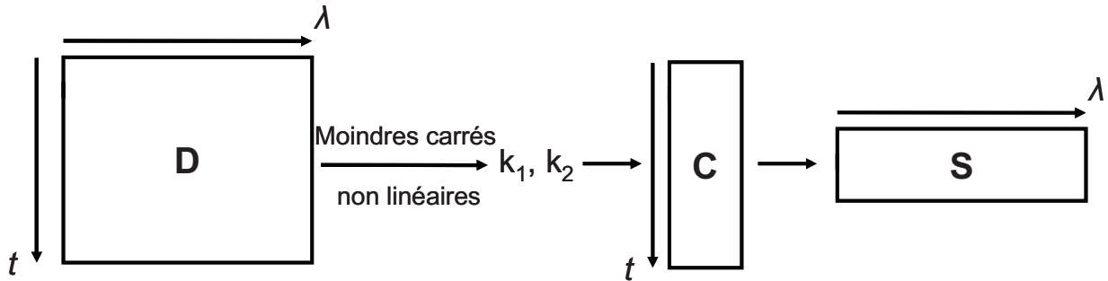
Figure 26 : Principe de la méthode des moindres carrés non linéaires, la matrice D est utilisée pour estimer les paramètres d'un modèle (ici deux paramètres cinétiques k_1 et k_2 ) qui sont ensuite utilisés pour calculer C et S .
