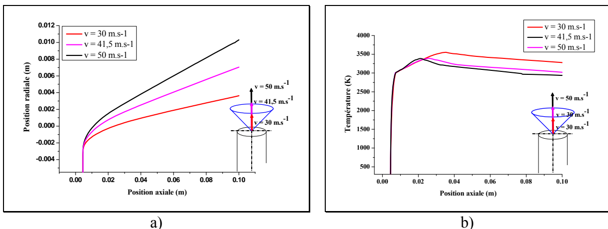
Figure III-6 : a) Trajectoires et b) Températures à la surface d'un particule de zircon ( d_p = 25\mu\text{m} ) injectée avec différentes vitesses et avec \Phi = 0^\circ et \delta = 20^\circ
