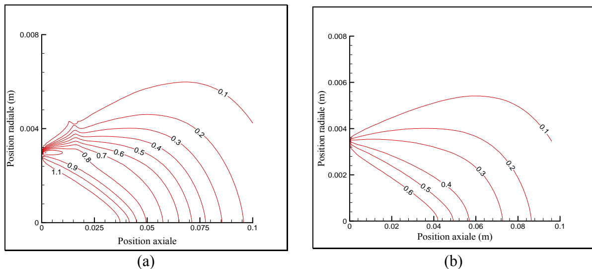
Figure IV-21 : Iso-conductivités thermiques ( \text{W.m}^{-1}.\text{K}^{-1} ) dans le plan axial contenant l'injecteur pour des jets Ar-H 2 (a) 60 L.min -1 (1,25 g.s -1 ) 25% vol en hydrogène et (b) 50 L.min -1 (1,23 g.s -1 ) 10 % vol en hydrogène
