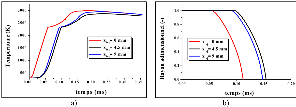
Figure IV-15 : Comparaison de l'évolution en fonction du temps (a) de la température de la surface et (b) des fronts de fusion dans un particule d'alumine de 30 μm de diamètre injectée à différentes positions axiales, dans les conditions de projection de référence
