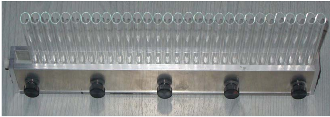
Figure IV-61 : Dispositif de récupération de poudre au dessous de l'injecteur
