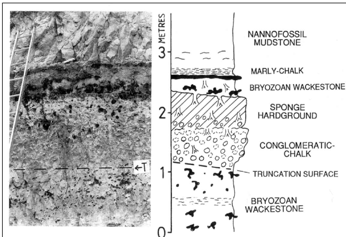
Figure A.6 : Modèle de remplissage des chenaux d'Etretat (d'après Quine et Bosence, 1991).
