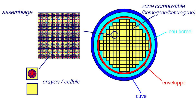
FIG. 1.5 – Géométrie radiale multi-échelle d'un cœur
