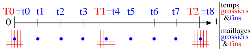
FIG. 5.1 – Deux échelles, en temps et espace, emboîtées pour la représentation quasi-statique du flux de neutrons.
