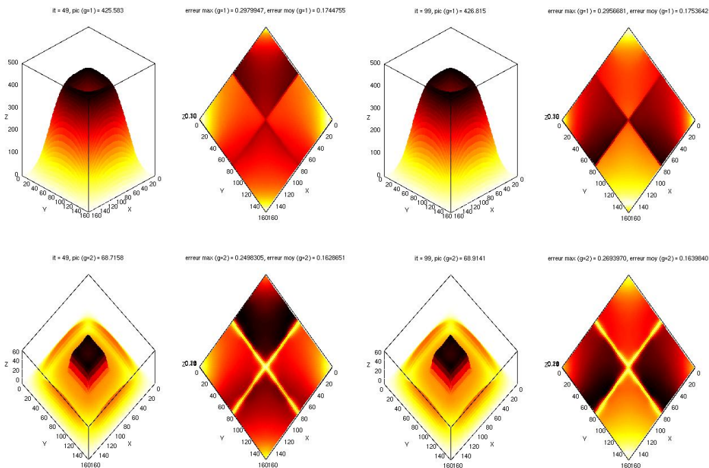
FIG. 9.8 – Flux et erreurs 2D avec LQS ( \delta t = 1\text{ms} et maillage grossier 2 \times 2 ) à l'état médian ( t = 0.1\text{s} ) et final ( t = 0.2\text{s} ) sans utiliser des coefficients de discontinuité.
