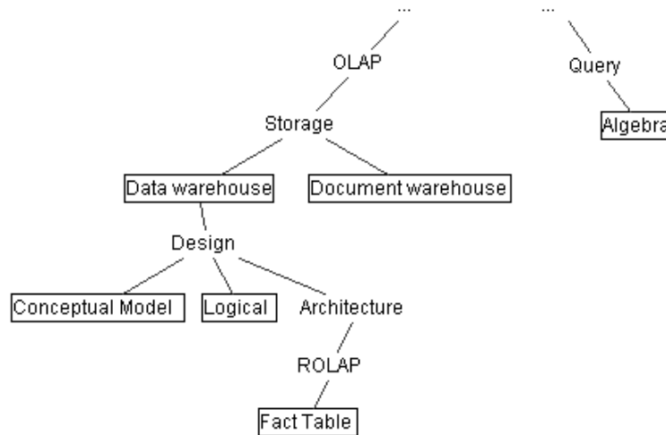
Figure 47 – Le positionnement des différents mots-clé dans l’ontologie de domaine O_{IS} (représenté partiellement).
