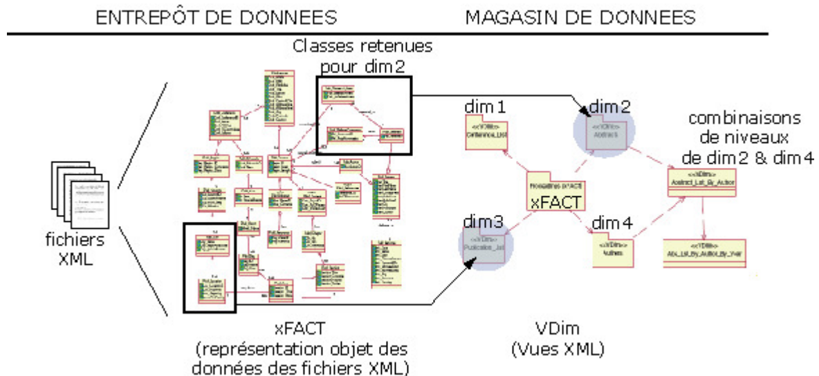
Figure 17 - Constitution des dimensions virtuelles à partir du xFACT [Nassis et al., 2004] .
