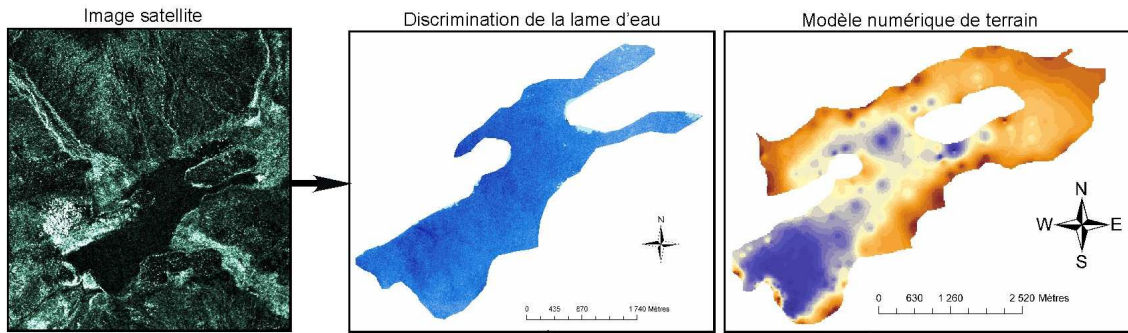
Figure 88 : Méthode de détermination du volume d'eau du lac (apports de la télédétection et du SIG)
