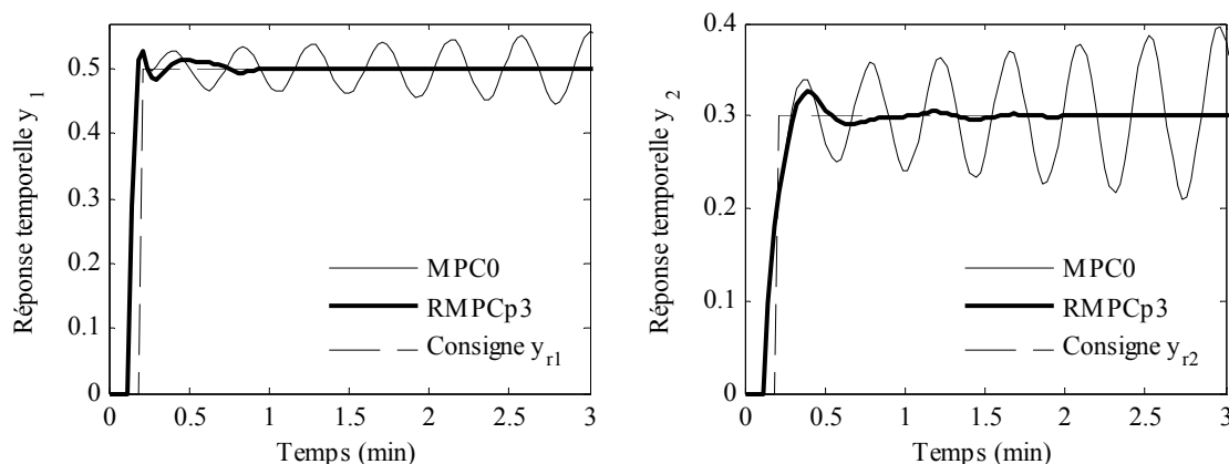
Figure 4.28 Influence d'une dynamique négligée sur le transfert u_1/y_1 considérée en A_0 . Sorties du réacteur : Concentration du fluide (à gauche) ; Température du réacteur (à droite)
