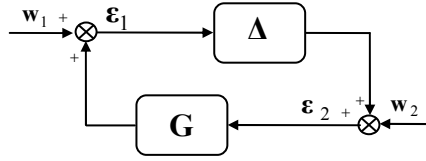
Figure 3.4 Théorème du petit gain
