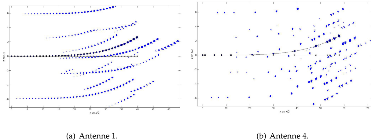
FIG. 4.5: Résultats de 500 autocalibrations par une méthode de sous-espace/modules constants d'antennes fortement déformées, environnement bruité.
