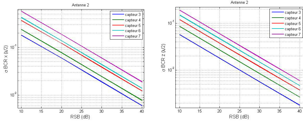
FIG. 2.5: Bornes de Cramèr-Rao en x et z des capteurs de l'antenne 2.
