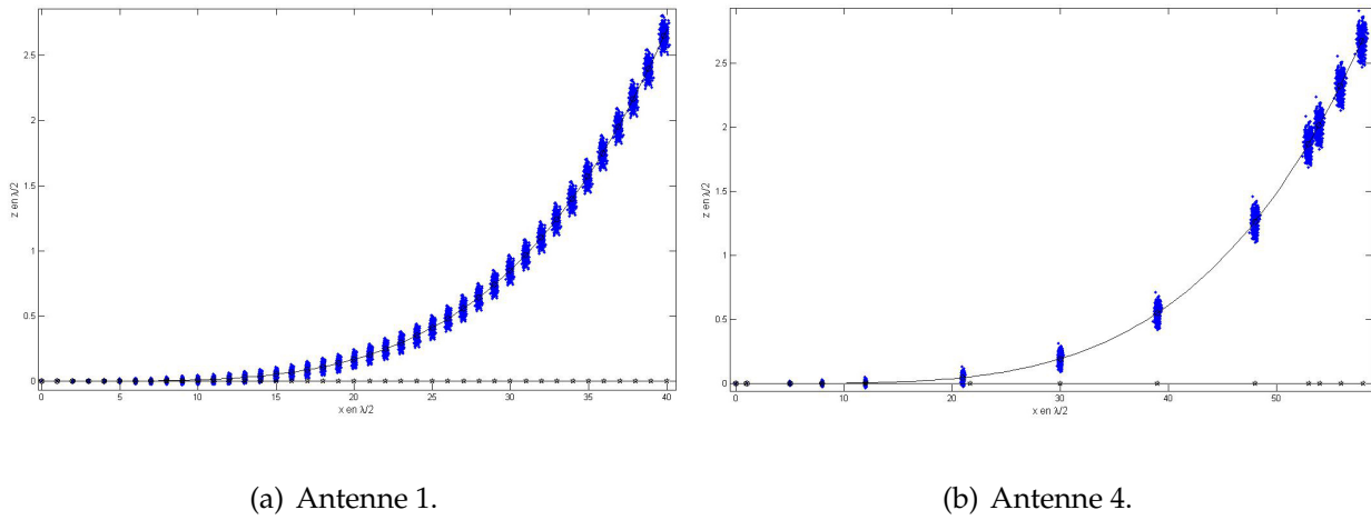
FIG. 4.6: Résultats de 500 autocalibrations de grandes antennes fortement déformées, avec contraintes de déformations, environnement bruité.
