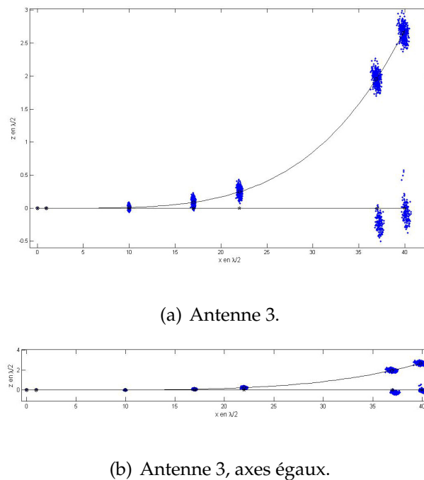
FIG. 4.7: Résultats de 500 autocalibrations de l'antenne 3 fortement déformée, avec contraintes de déformations, environnement bruité (RSB=20dB, N_s = 300 ).
